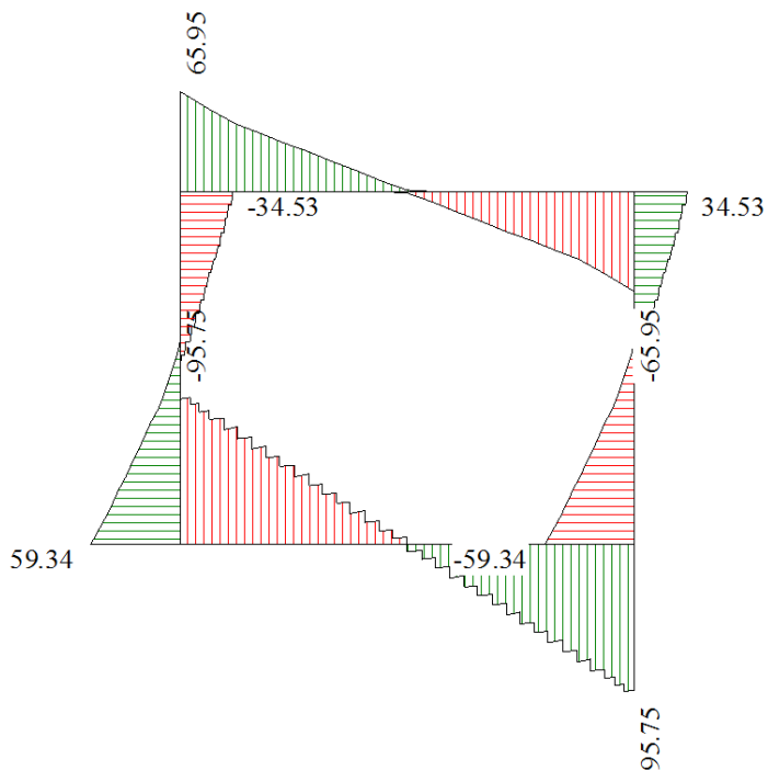
Figura 9 - Diagramma involuppo taglio - SLU
