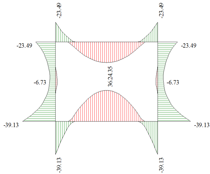
Figura 7 - Diagramma involuppo momento flettente – SLU
