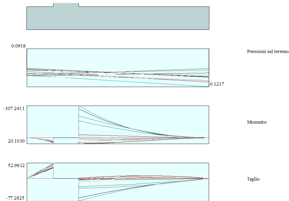
Figura 14 - Diagramma involucro sollecitazioni – fondazione
