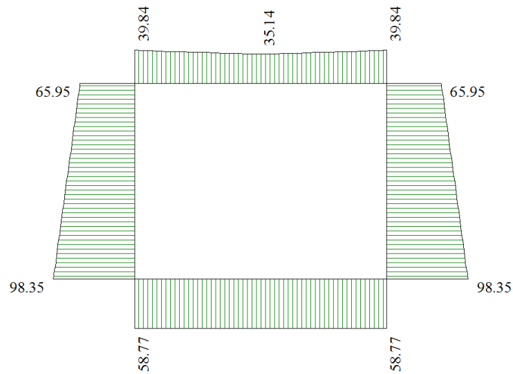
Figura 11 - Diagramma involuppo sforzo normale - SLU
