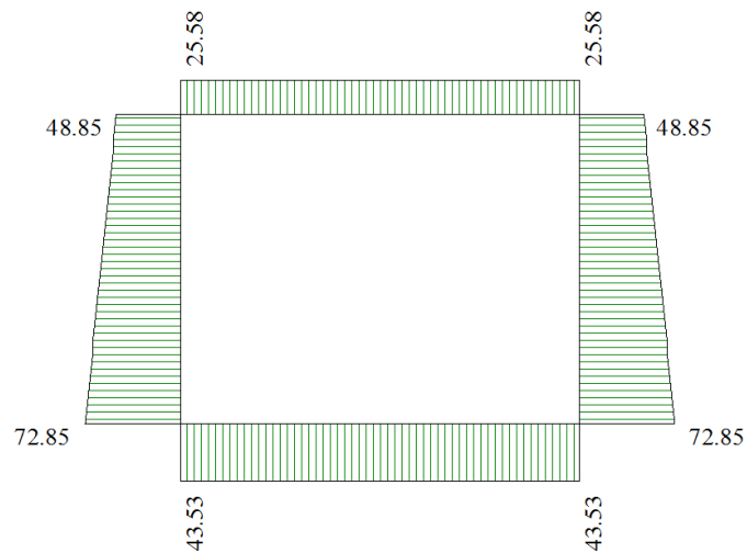
Figura 12 - Diagramma involuppo sforzo normale - SLE
