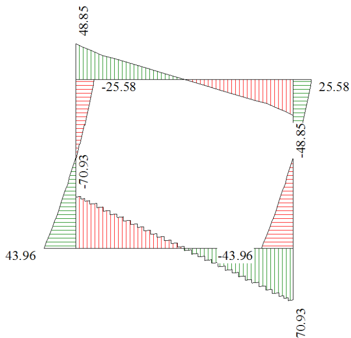
Figura 10 - Diagramma involuppo taglio - SLE
