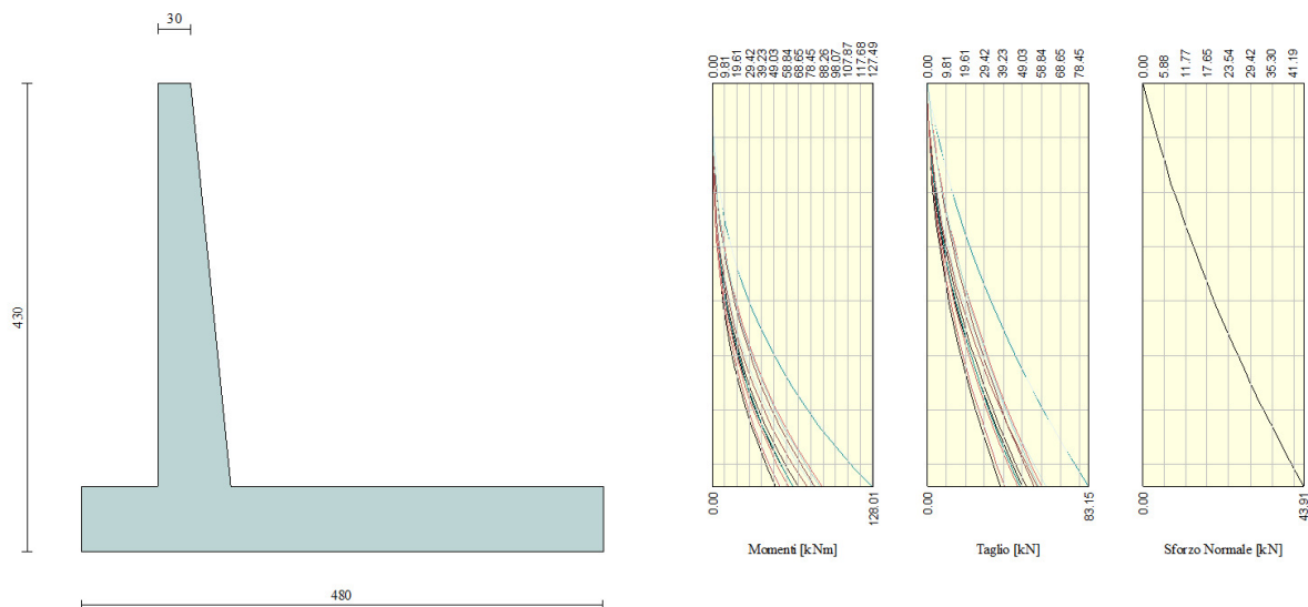
Figura 13 - Diagramma involuppo sollecitazioni – paramento
