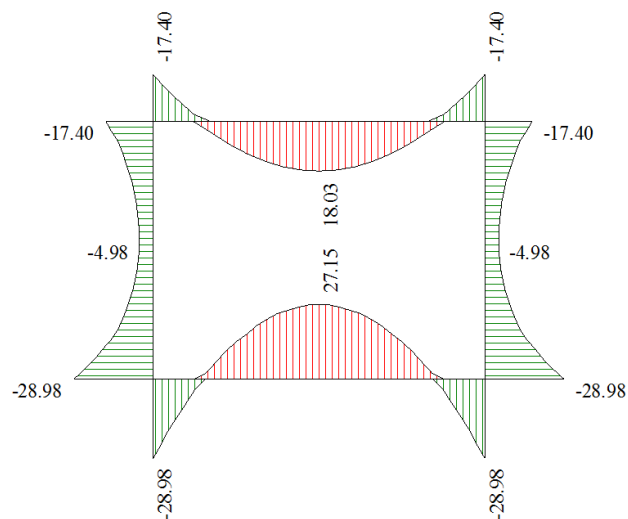
Figura 8 - Diagramma involuppo momento flettente – SLE
