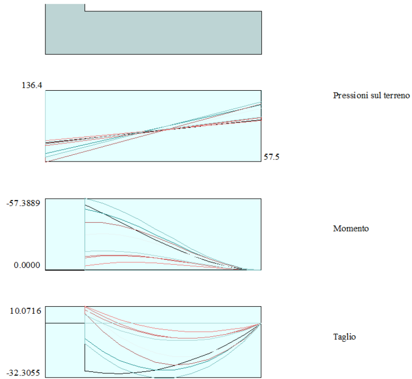
Figura 10 - Diagramma involucro sollecitazioni – fondazione
