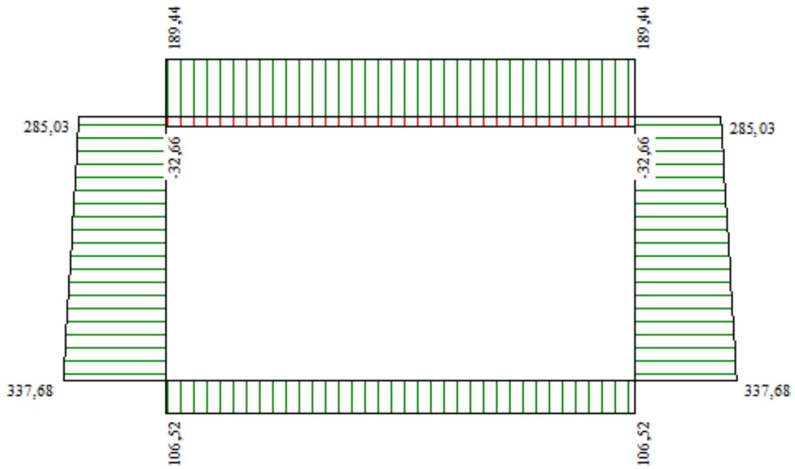
Figura 7 - Diagramma involuppo sforzo normale - SLU
