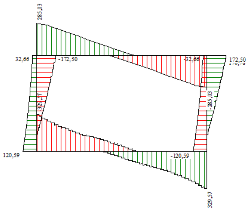
Figura 5 - Diagramma involuopo taglio - SLU
