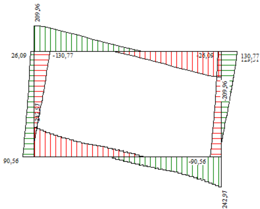
Figura 6 - Diagramma involuopo taglio - SLE
