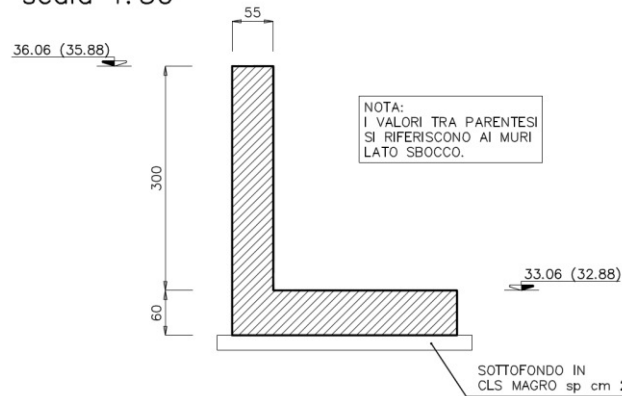
SEZIONE MURI SCATOLARE E-E scala 1:50
