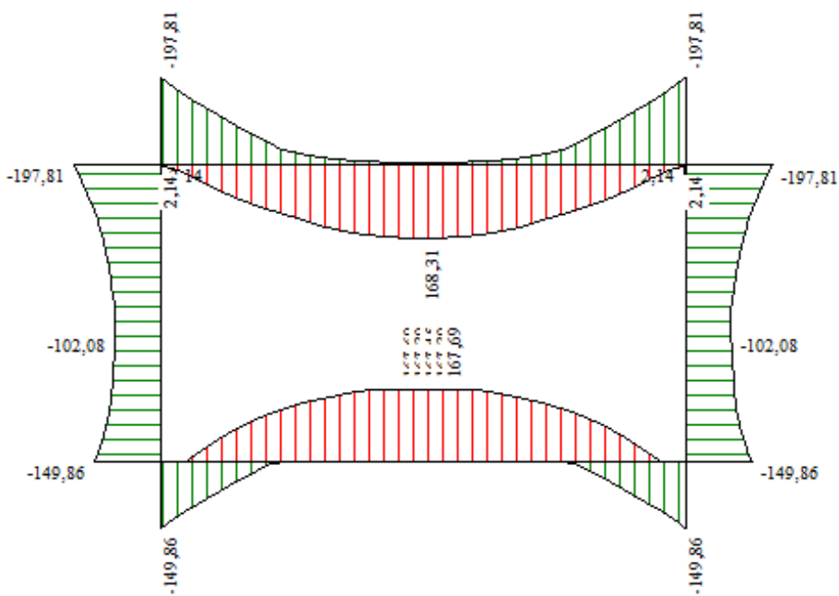
Figura 4 - Diagramma involuppo momento flettente – SLE
