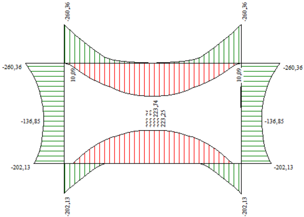
Figura 3 - Diagramma involuppo momento flettente – SLU
