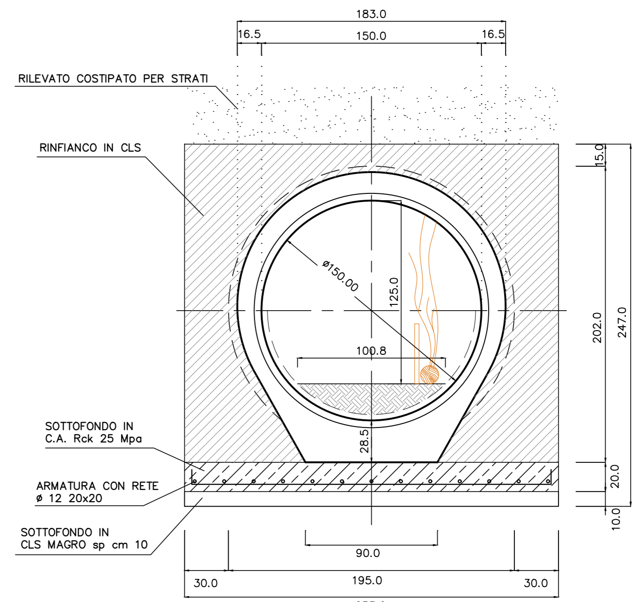
SEZIONE B-B scala 1:25
