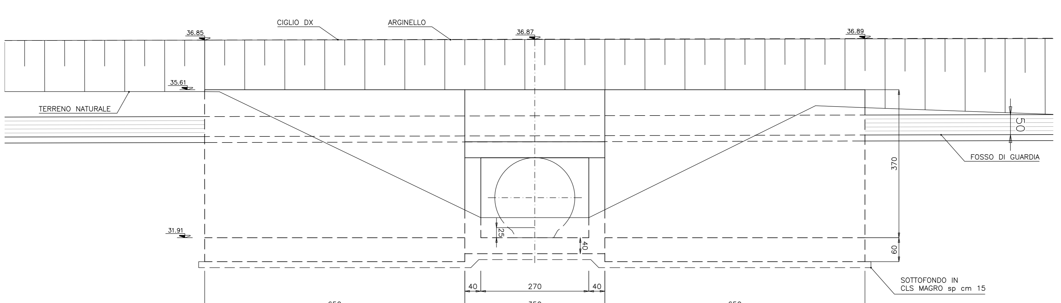
SEZIONE D-D scala 1:50
