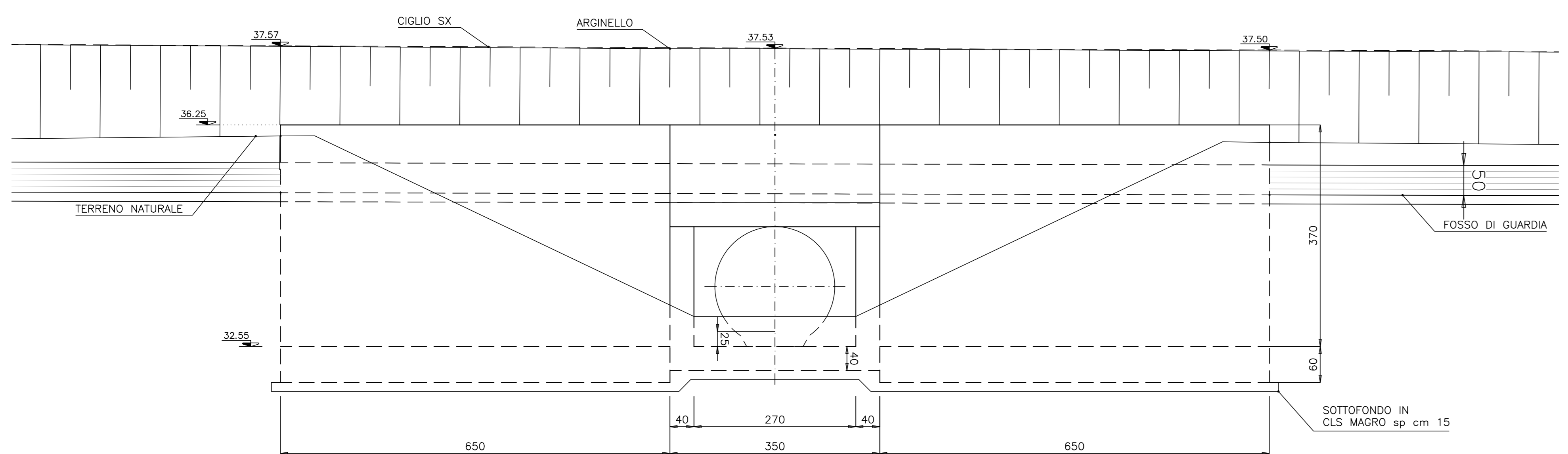
SEZIONE C-C scala 1:50
