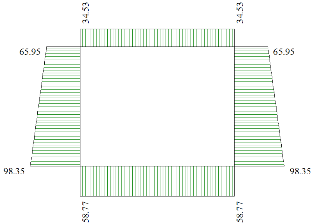
Figura 11 - Diagramma involuppo sforzo normale - SLU
