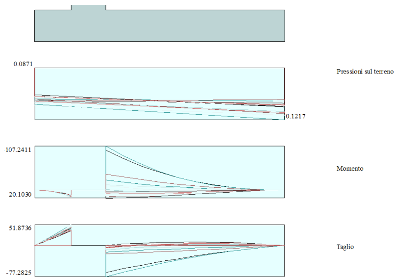
Figura 14 - Diagramma involuipo sollecitazioni – fondazione
