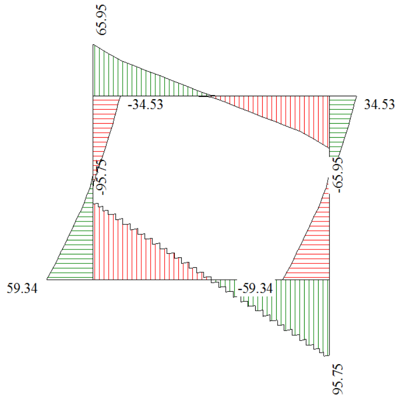
Figura 9 - Diagramma involuppo taglio – SLU
