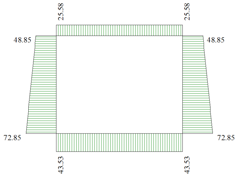
Figura 12 - Diagramma involuppo sforzo normale - SLE
