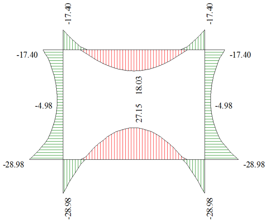
Figura 8 - Diagramma involuppo momento flettente – SLE
