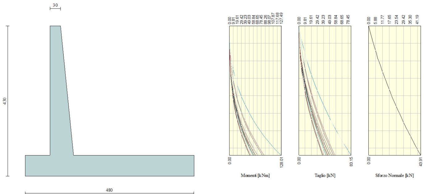
Figura 13 - Diagramma involuppo sollecitazioni - paramento
