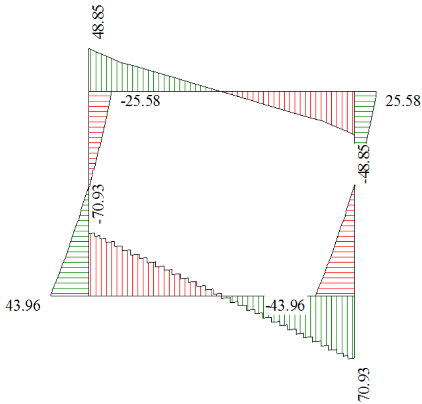
Figura 10 - Diagramma involuppo taglio - SLE
