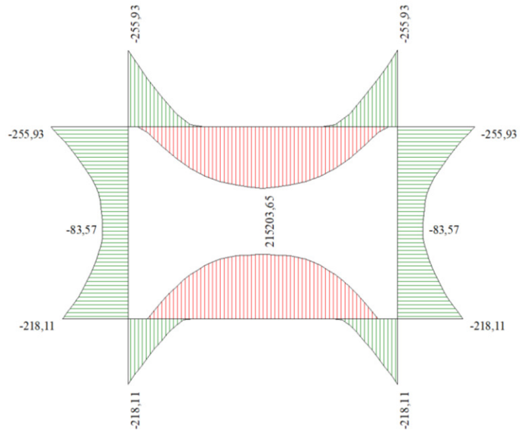
Figura 3 - Diagramma involuppo momento flettente - SLU
