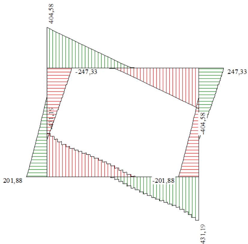
Figura 5 - Diagramma involuppo taglio - SLU
