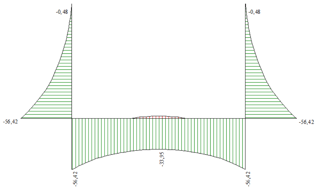
Figura 9 - Diagramma involuppo momento flettente – SLU
