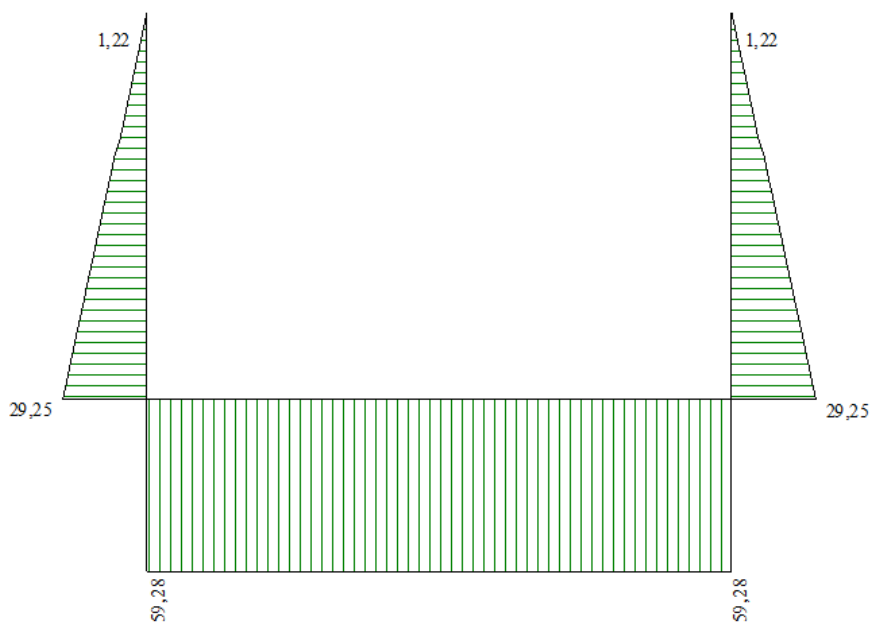
Figura 13 - Diagramma involuipo sforzo normale - SLU
