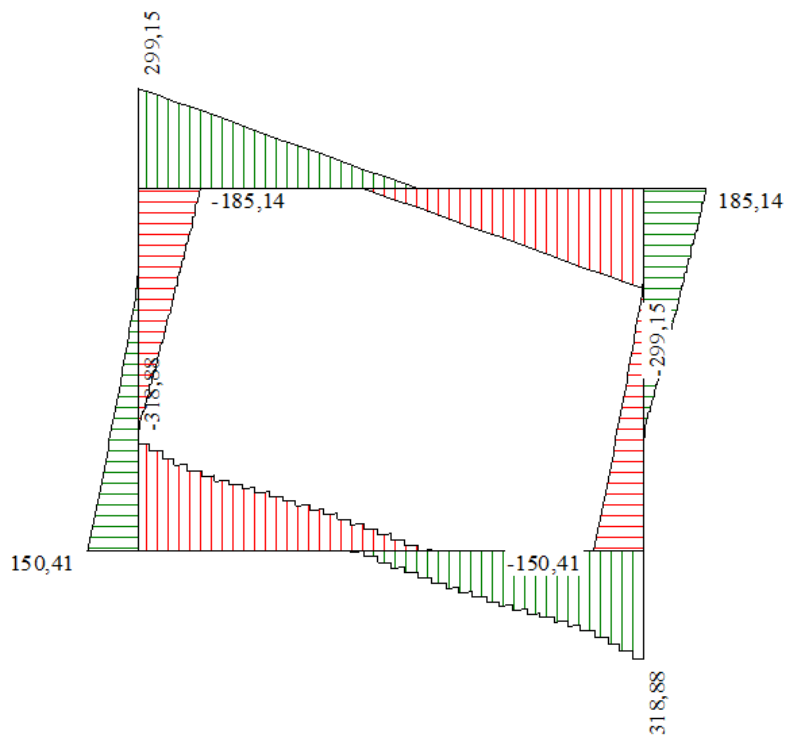
Figura 6 - Diagramma involuppo taglio - SLE
