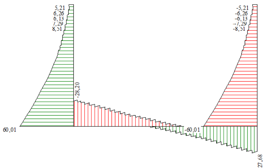
Figura 10 - Diagramma involuipo momento flettente – SLE
