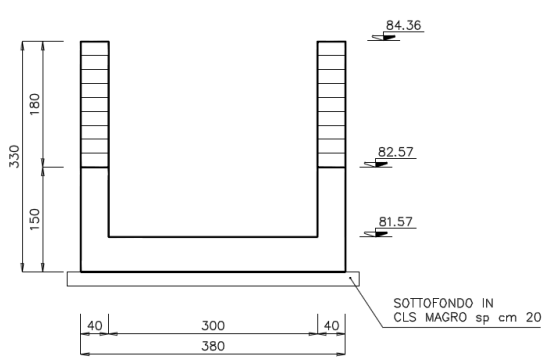
SEZIONE MURI SCATOLARE G-G scala 1:50
