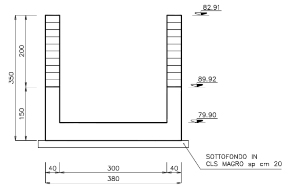
SEZIONE MURI SCATOLARE H-H scala 1:50
