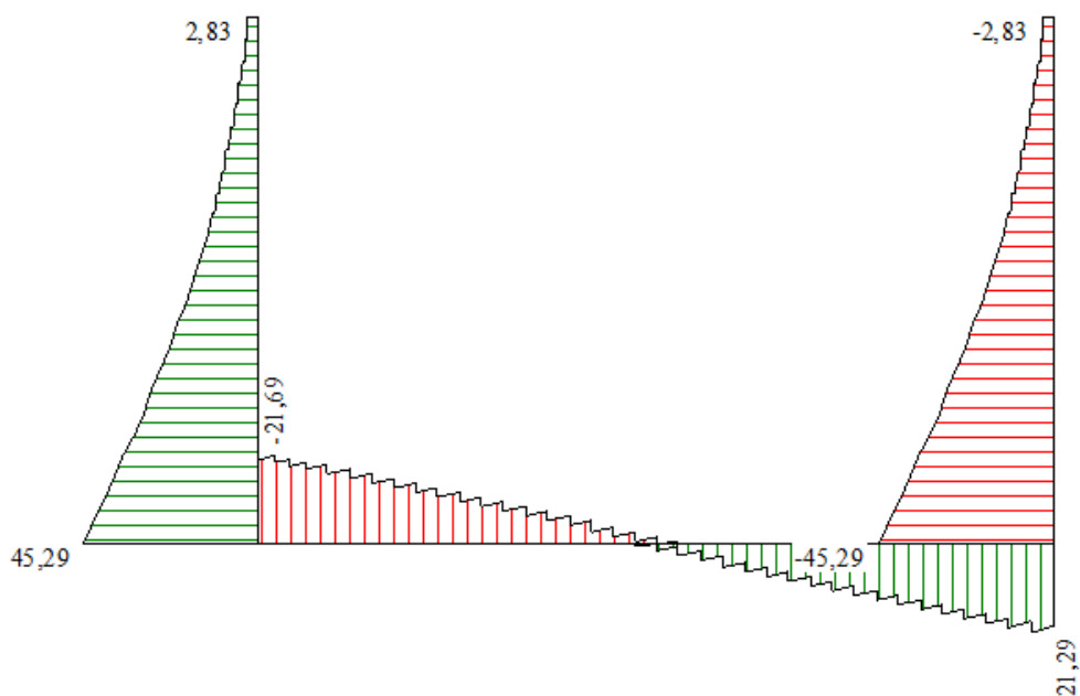
Figura 12 - Diagramma involuipo taglio - SLE
