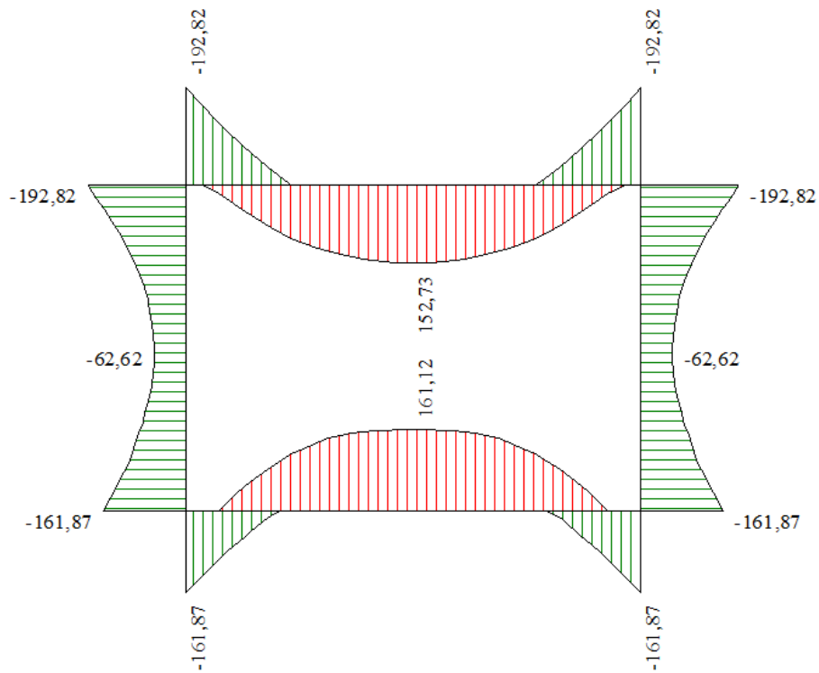
Figura 3 - Diagramma involuppo momento flettente - SLU
