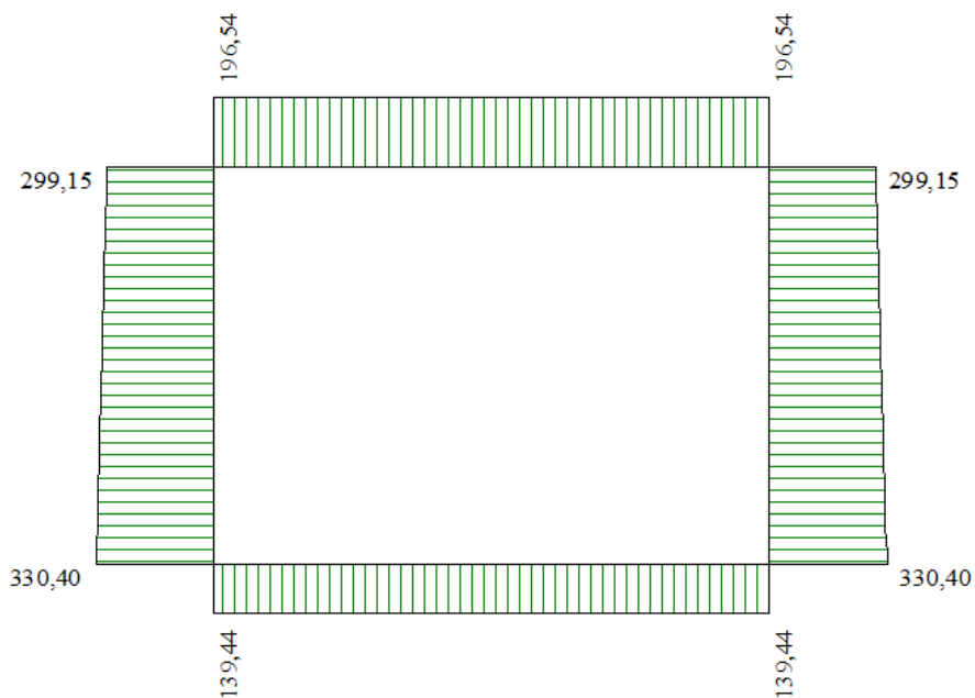
Figura 7 - Diagramma involuppo sforzo normale - SLU
