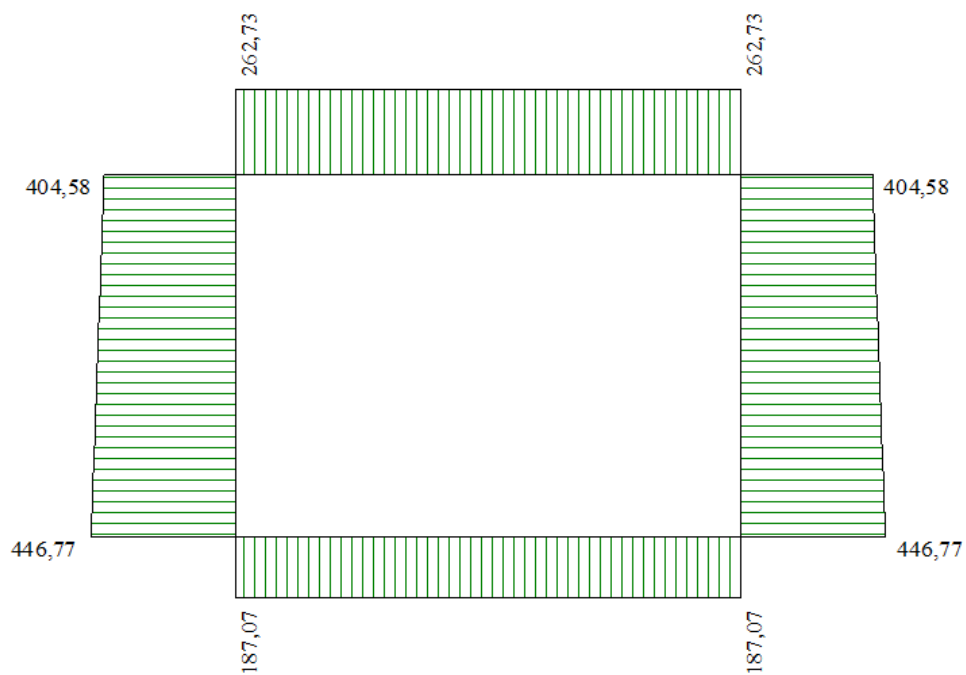
Figura 7 - Diagramma involuppo sforzo normale - SLU
