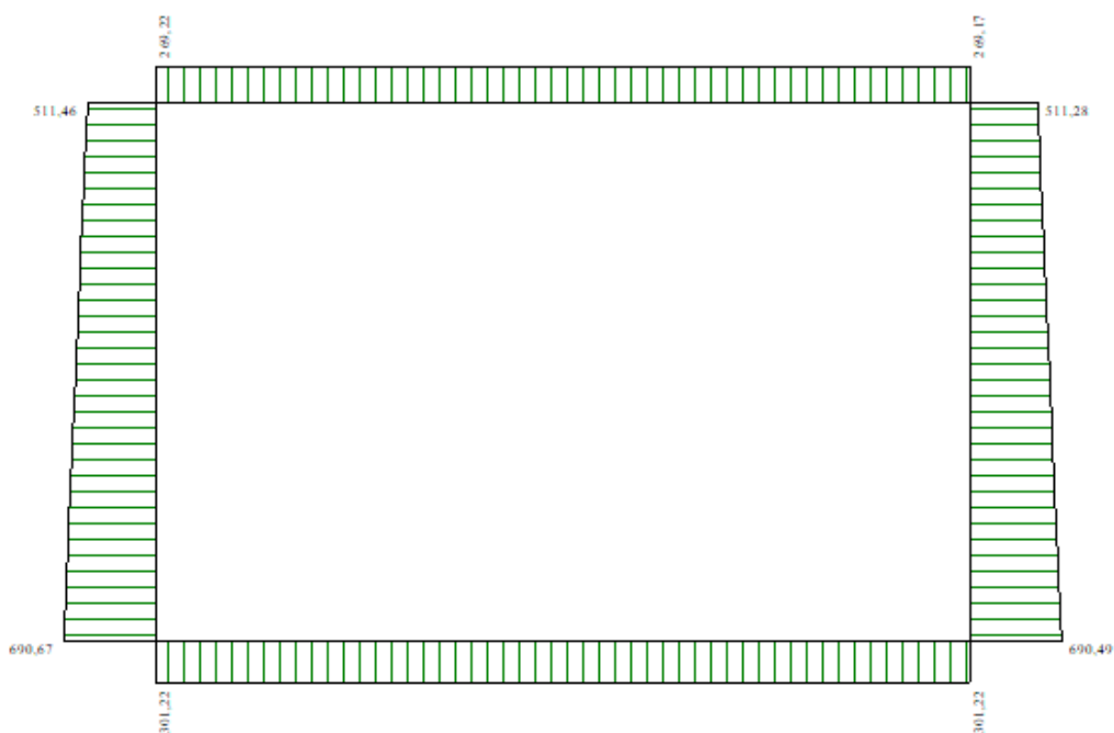
Figura 7 - Diagramma involuppo sforzo normale - SLU
