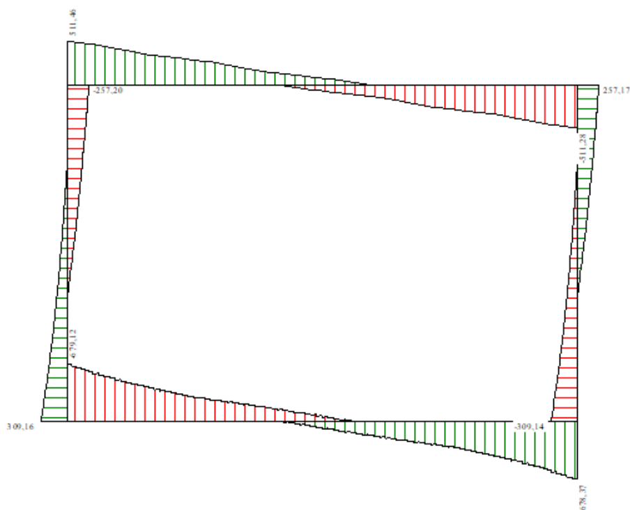
Figura 5 - Diagramma involucro taglio – SLU
