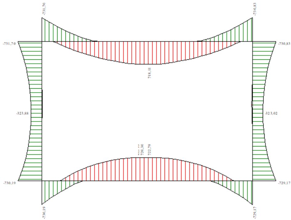
Figura 3 - Diagramma involuppo momento flettente – SLU
