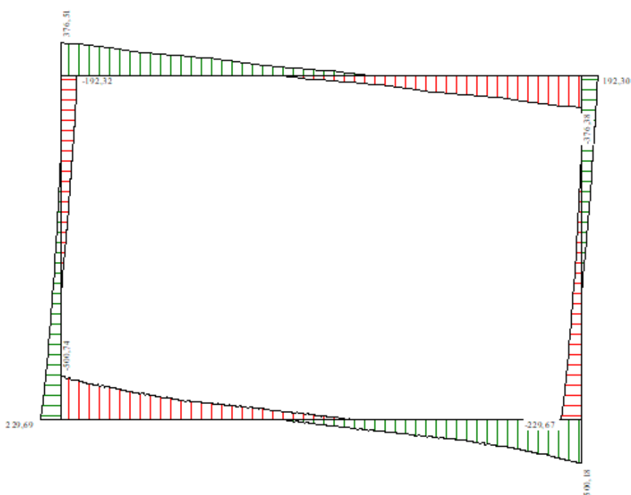
Figura 5 - Diagramma involucro taglio – SLU
