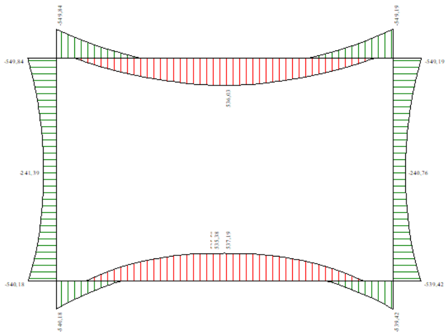
Figura 3 - Diagramma involuppo momento flettente – SLU
