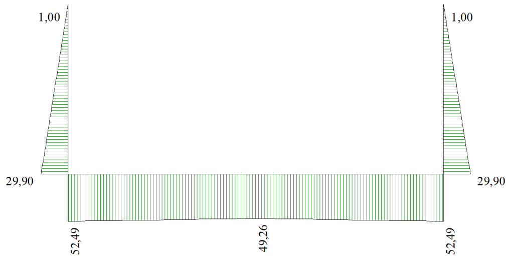
Figura 16 - Diagramma involuppo sforzo normale - SLE
