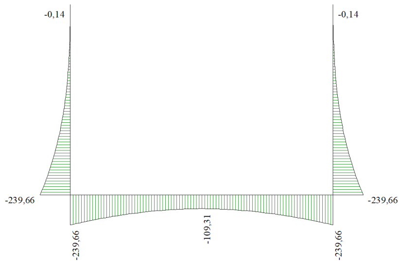
Figura 24 - Diagramma involuppo momento flettente – SLE
