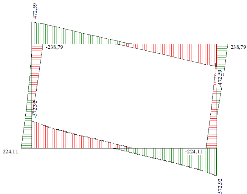
Figura 7 - Diagramma involuppo taglio – SLU
