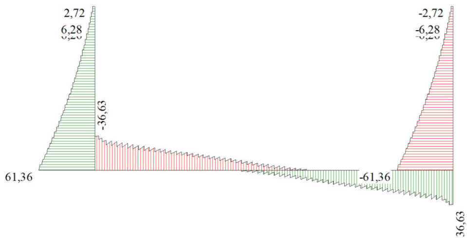
Figura 13 - Diagramma involuppo taglio – SLU
