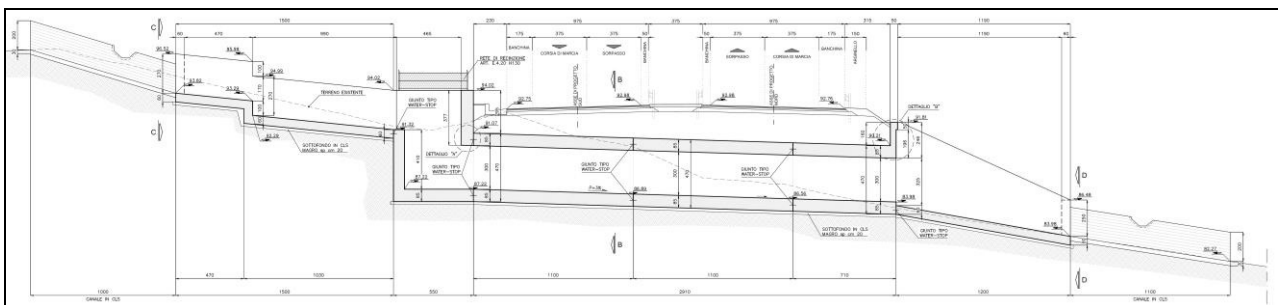
Figura 2 – Profilo longitudinale
