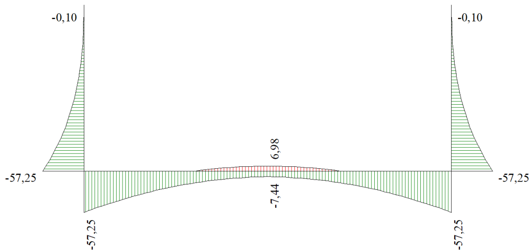
Figura 12 - Diagramma involuppo momento flettente – SLE
