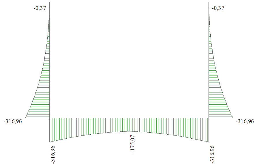
Figura 23 - Diagramma involuppo momento flettente – SLU
