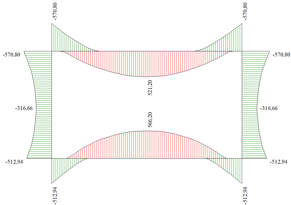
Figura 5 - Diagramma involuppo momento flettente – SLU
