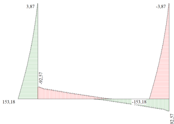
Figura 25 - Diagramma involuppo taglio – SLU
