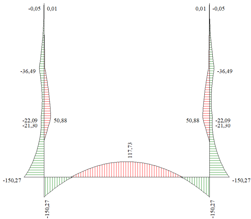
Figura 18 - Diagramma involuopo momento flettente – SLE
