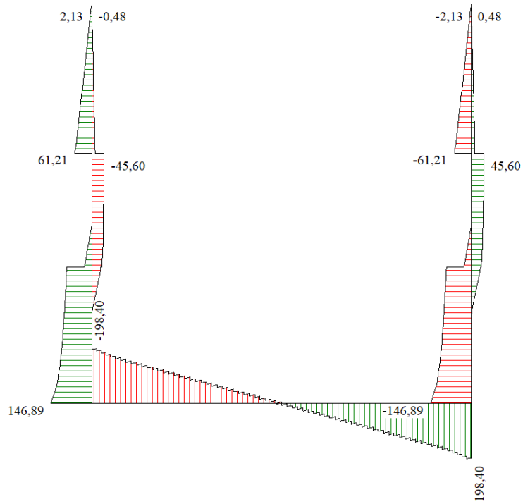
Figura 19 - Diagramma involuppo taglio – SLU
