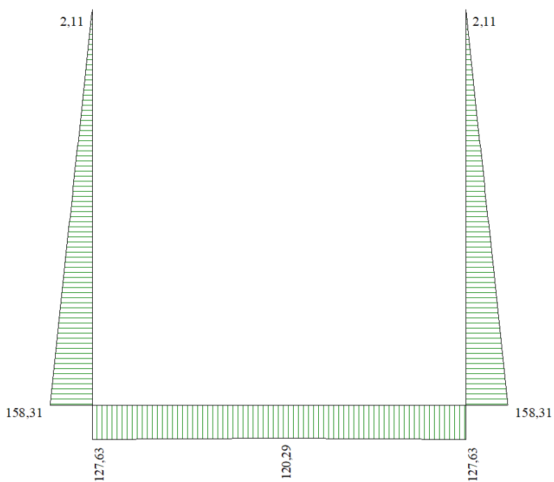
Figura 22 - Diagramma involuppo sforzo normale - SLE
