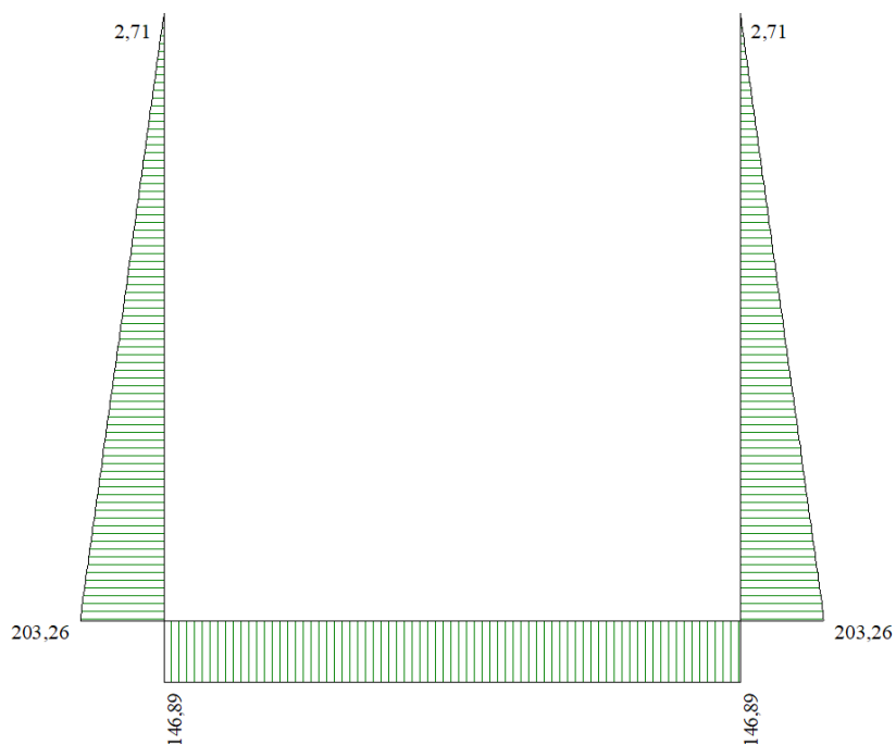
Figura 21 - Diagramma involuppo sforzo normale – SLU
