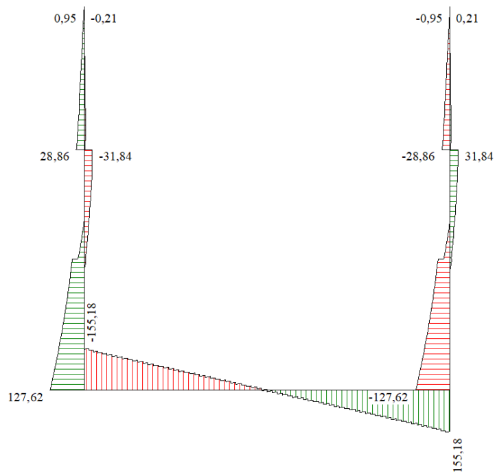
Figura 20 - Diagramma involuppo taglio – SLE
