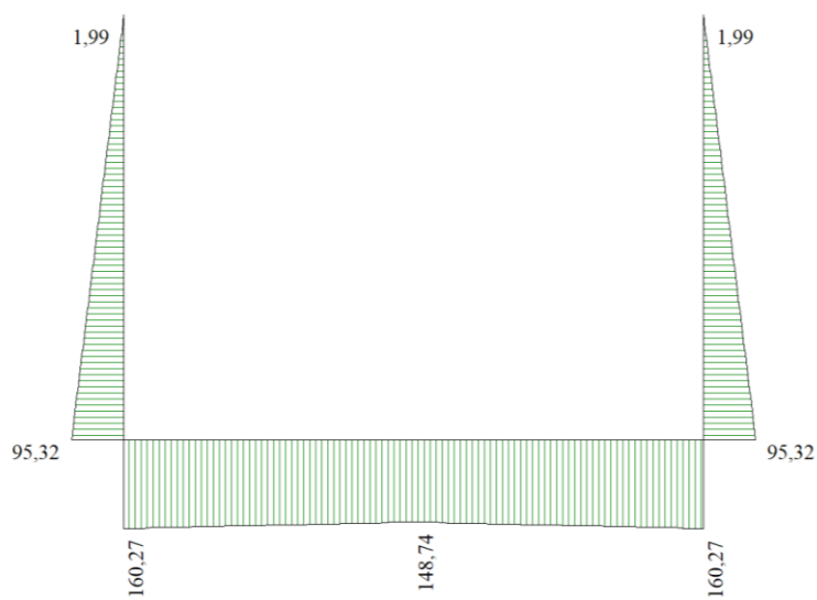
Figura 27 - Diagramma involuppo sforzo normale – SLU
