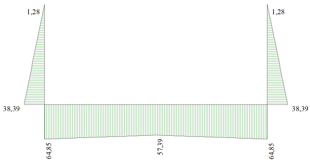
Figura 15 - Diagramma involuppo sforzo normale – SLU
