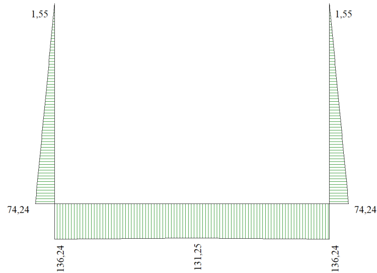
Figura 28 - Diagramma involuppo sforzo normale - SLE
