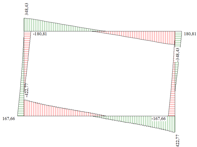
Figura 8 - Diagramma involuppo taglio – SLE
