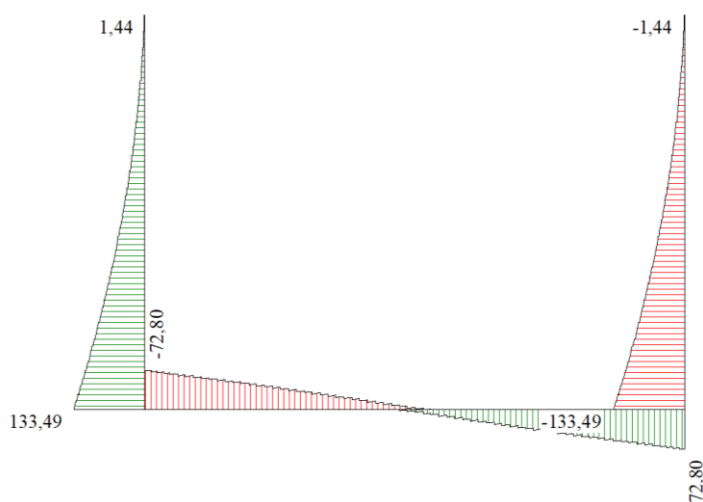
Figura 26 - Diagramma involuppo taglio – SLE
