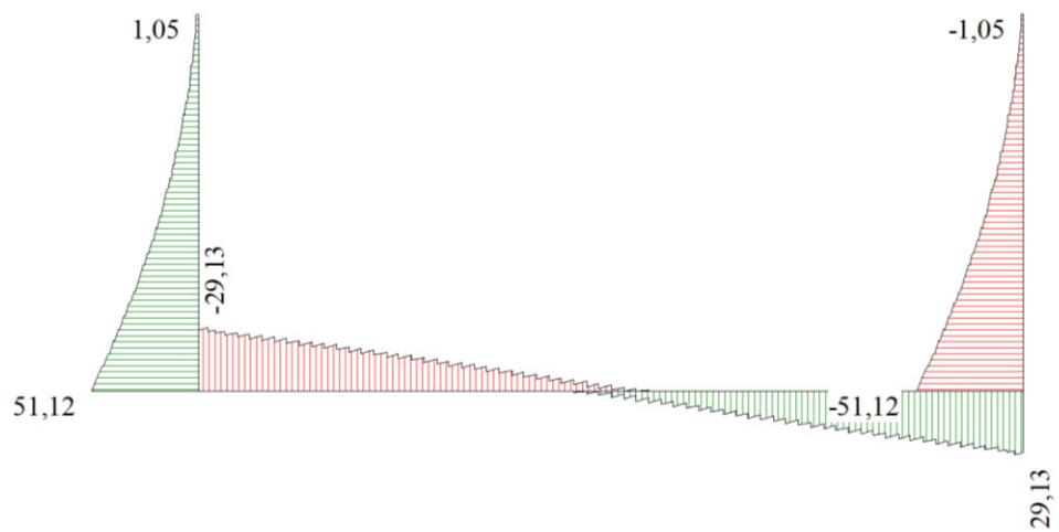
Figura 14 - Diagramma involuppo taglio – SLE
