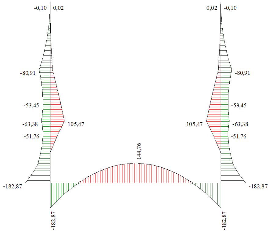
Figura 17 - Diagramma involuopo momento flettente – SLU
