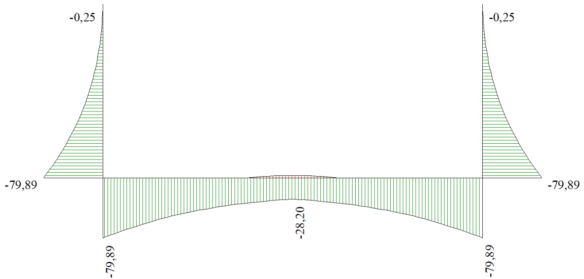
Figura 11 - Diagramma involuppo momento flettente – SLU
