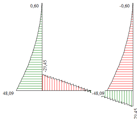
Figura 6 - Diagramma involuppo taglio – SLE
