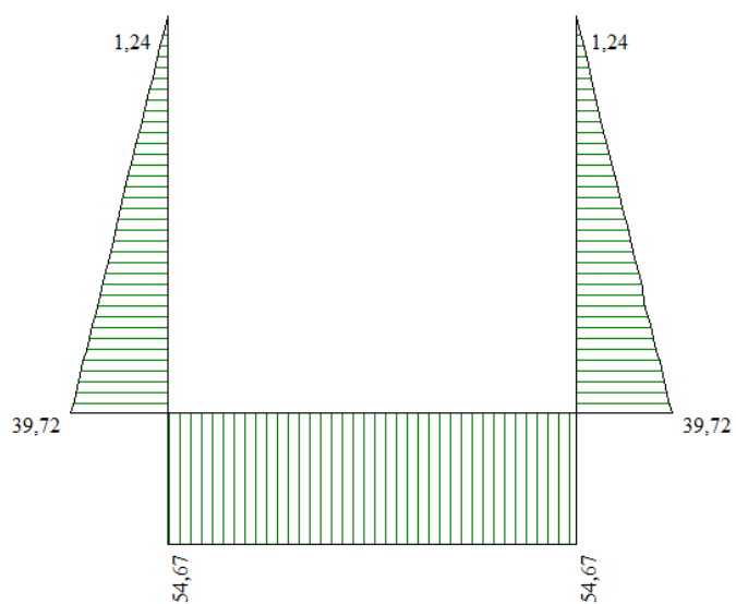
Figura 7 - Diagramma involuppo sforzo normale - SLU
