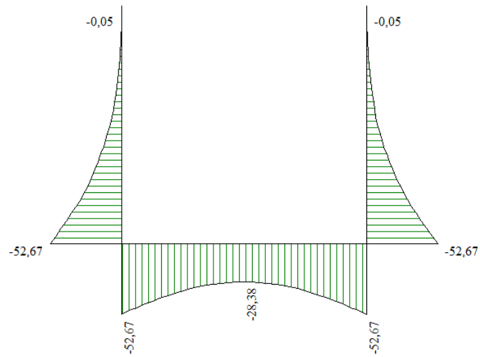
Figura 4 - Diagramma involuppo momento flettente – SLE
