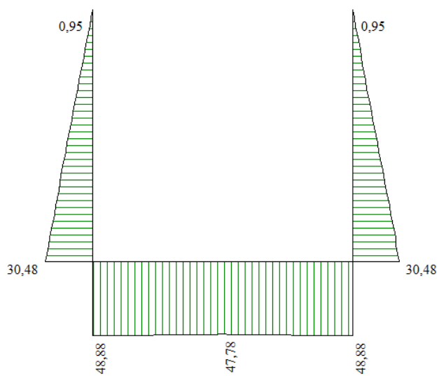
Figura 8 - Diagramma involuppo sforzo normale - SLE
