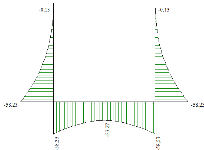
Figura 3 - Diagramma involuppo momento flettente – SLU
