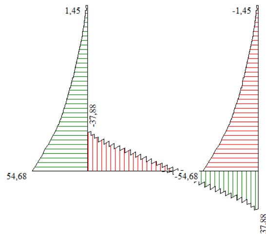
Figura 5 - Diagramma involuppo taglio – SLU
