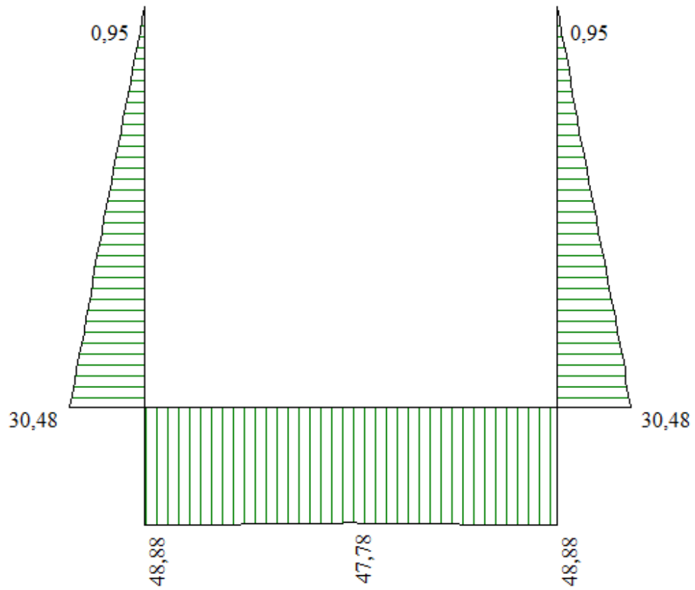
Figura 8 - Diagramma involuppo sforzo normale - SLE
