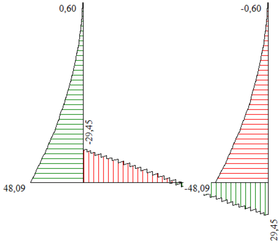
Figura 6 - Diagramma involuppo taglio – SLE
