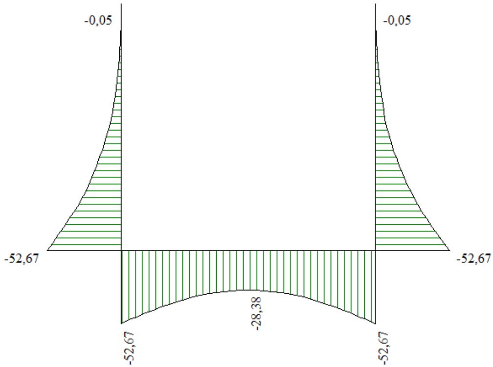
Figura 4 - Diagramma involuppo momento flettente – SLE
