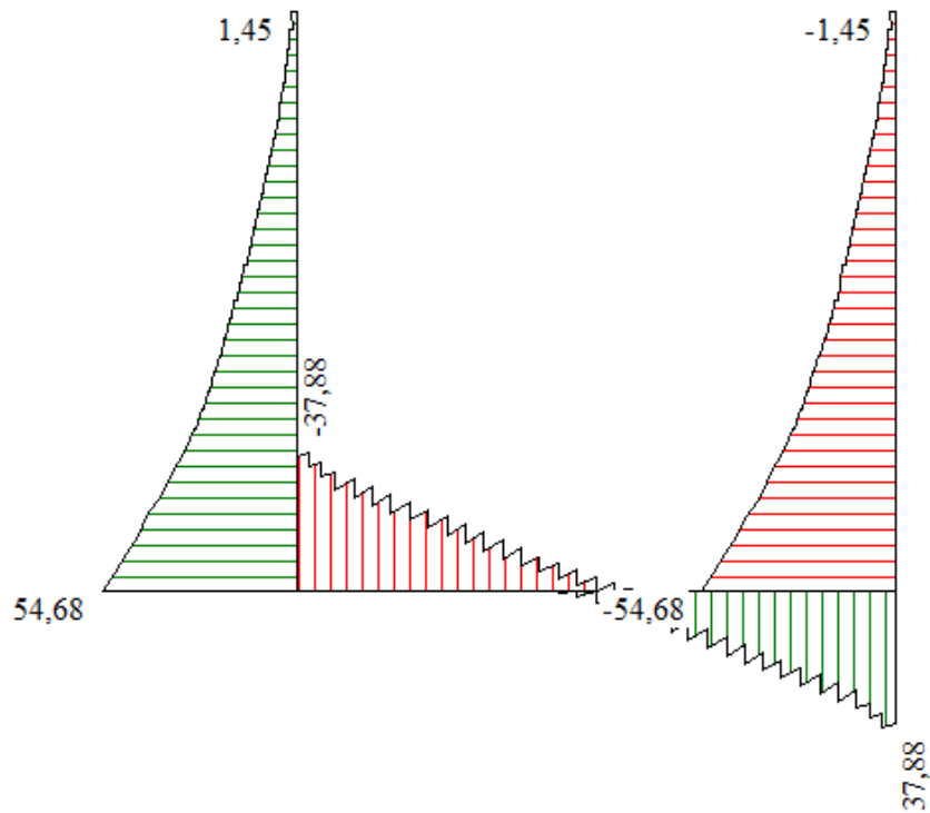
Figura 5 - Diagramma involuppo taglio – SLU
