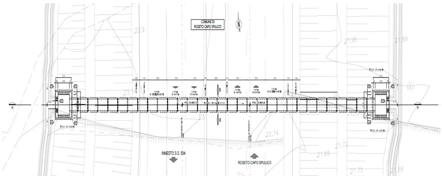
Figura 1 – Stralcio planimetrico
