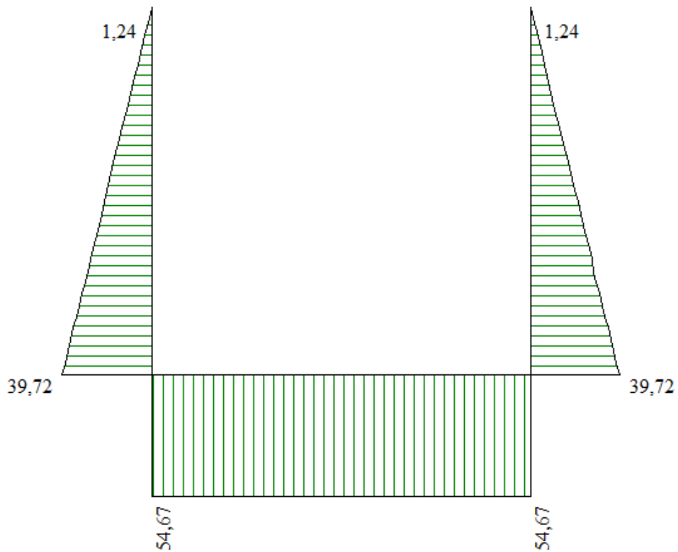
Figura 6 - Diagramma involuppo taglio – SLE
