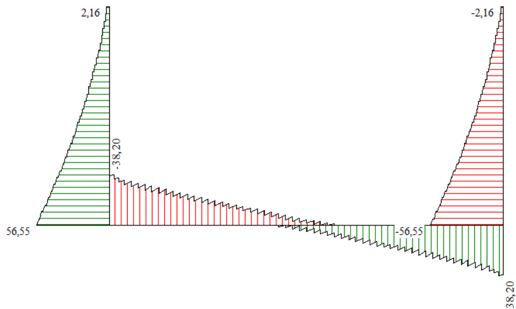
Figura 5 - Diagramma involuopo taglio – SLU
