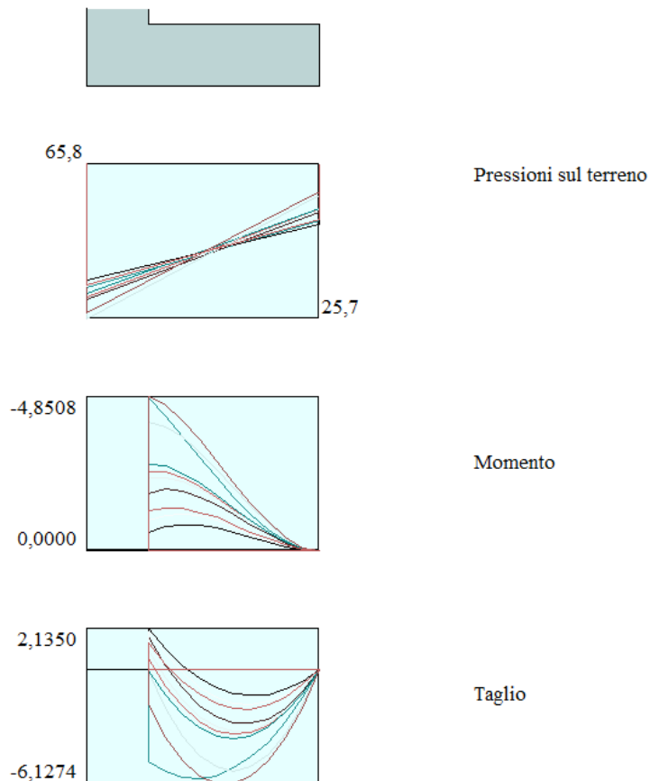
Figura 10 - Diagramma inviluppo sollecitazioni – fondazione
