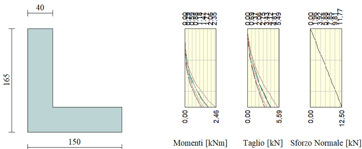
Figura 9 - Diagramma involuppo sollecitazioni - paramento
