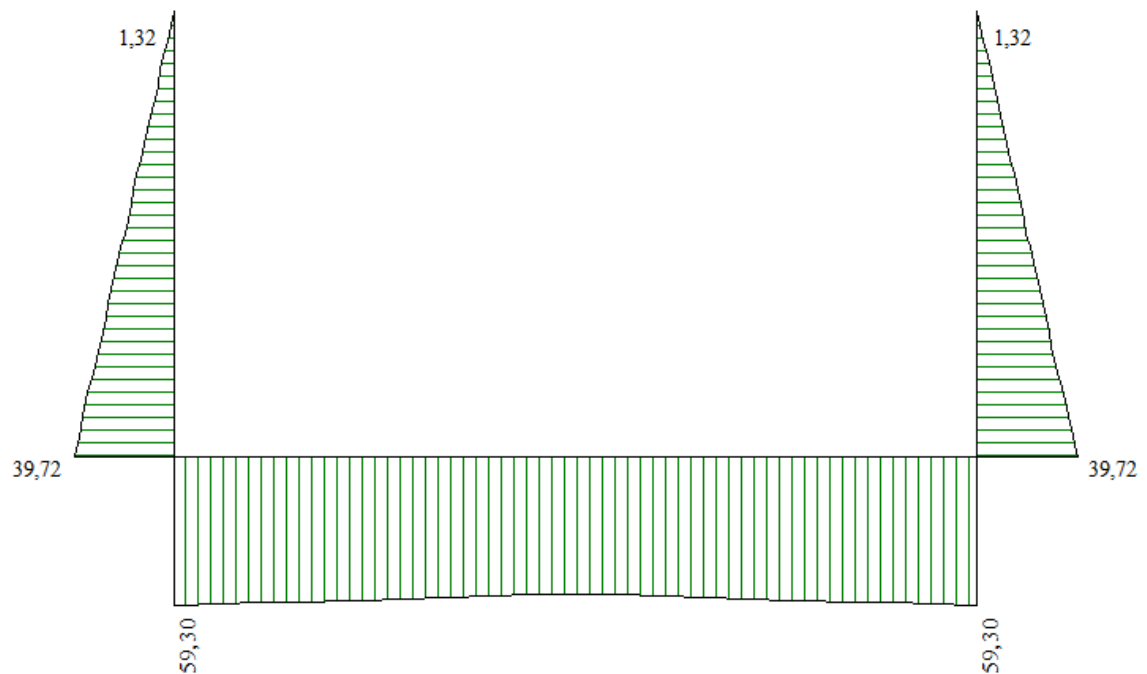
Figura 7 - Diagramma involuopo sforzo normale – SLU
