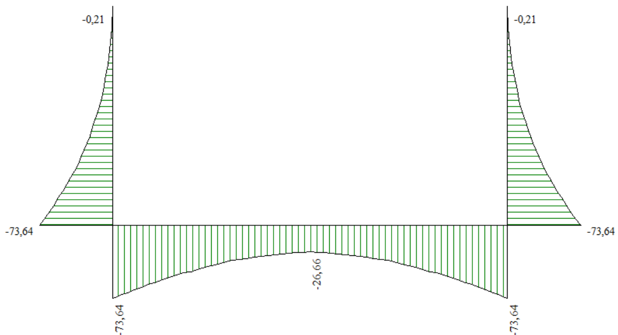
Figura 3 - Diagramma involuppo momento flettente – SLU
