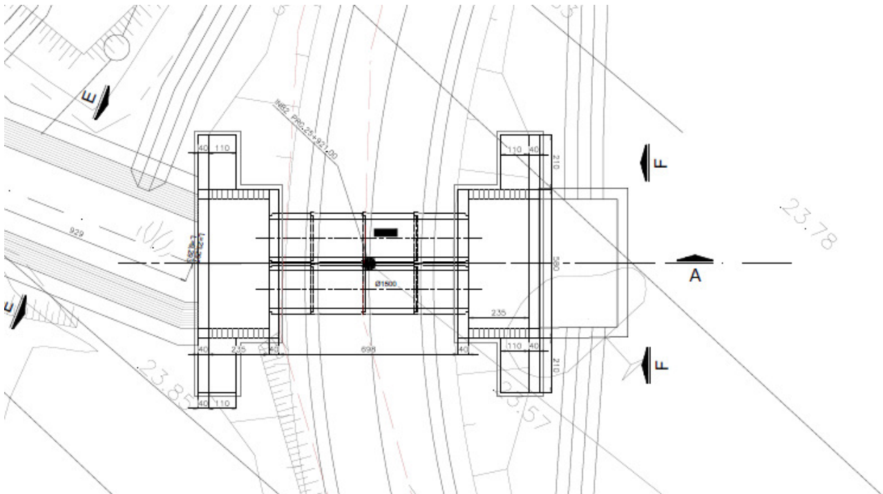
Figura 1 – Stralcio planimetrico
