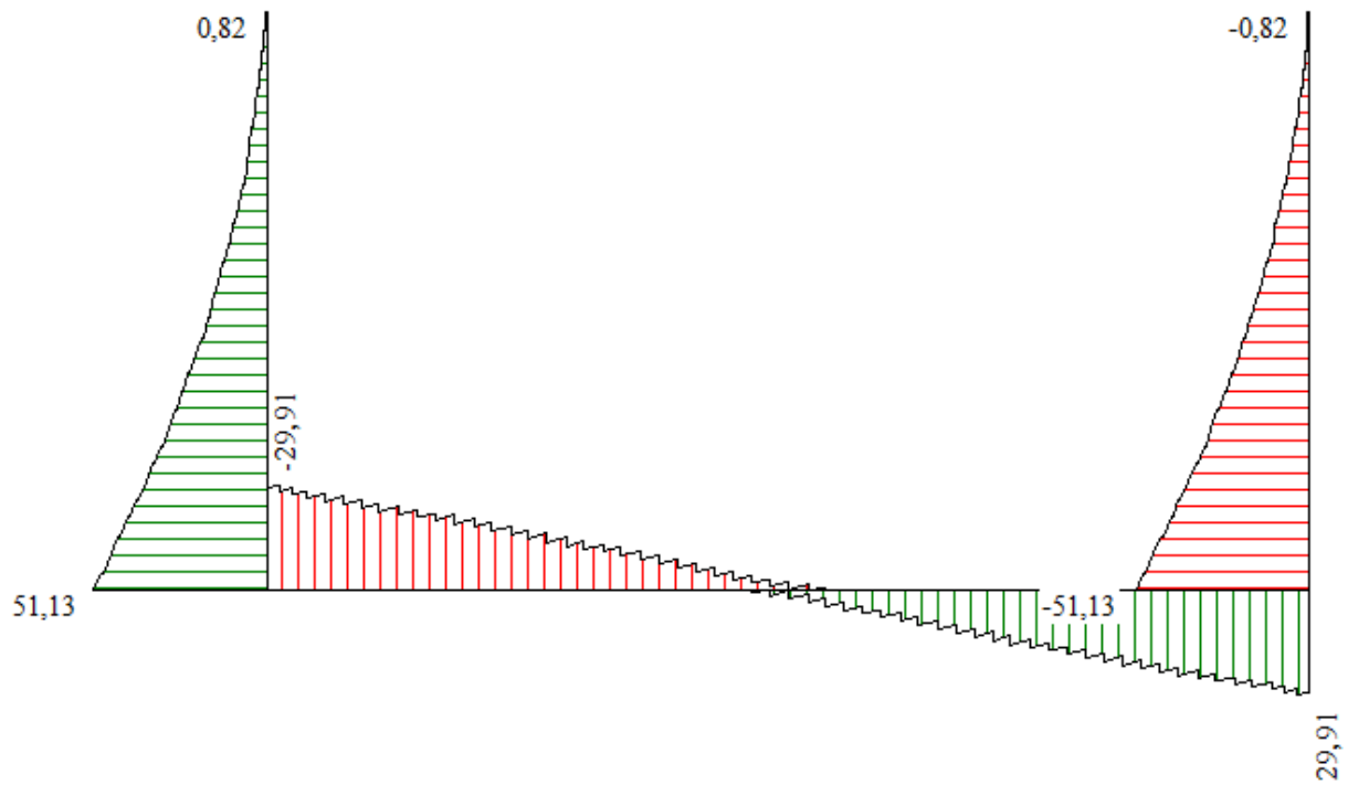
Figura 6 - Diagramma involuopo taglio – SLE
