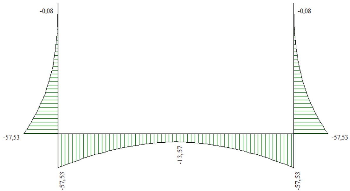
Figura 4 - Diagramma involuopo momento flettente – SLE
