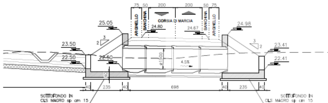
Figura 2 – Profilo longitudinale
