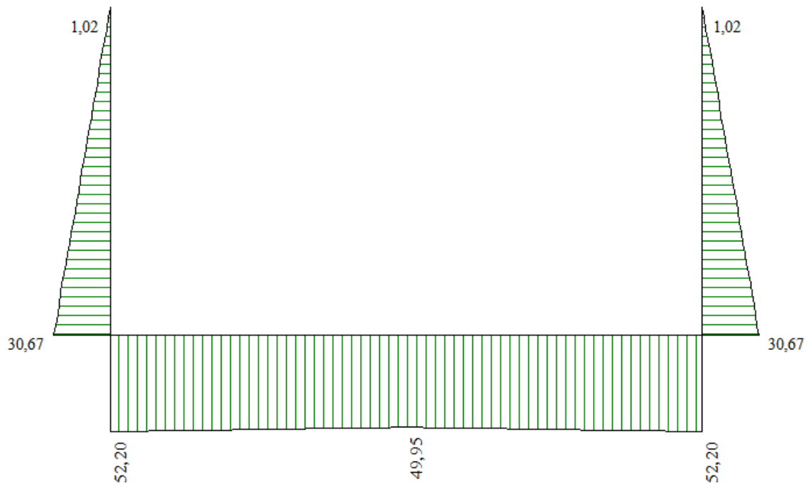
Figura 8 - Diagramma involuppo sforzo normale - SLE
