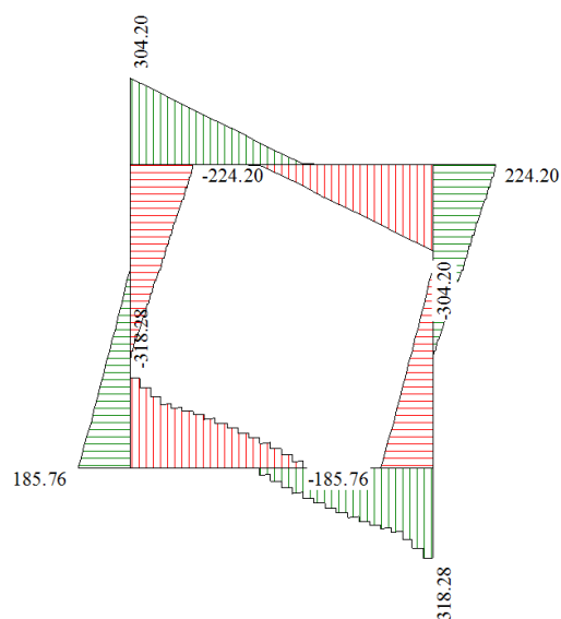
Figura 8 - Diagramma involuppo taglio – SLE
