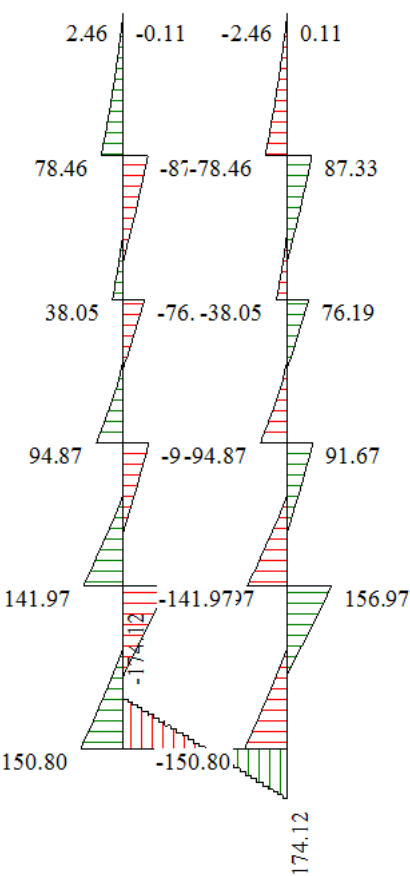
Figura 14 - Diagramma involuppo taglio – SLE
