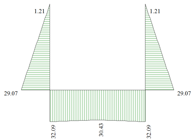
Figura 22 - Diagramma involuppo sforzo normale - SLE
