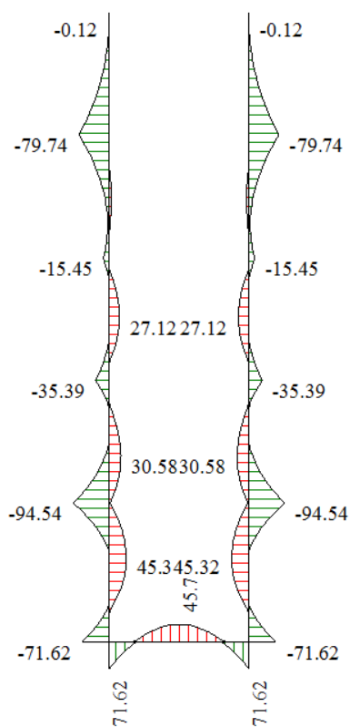
Figura 12 - Diagramma involuppo momento flettente – SLE
