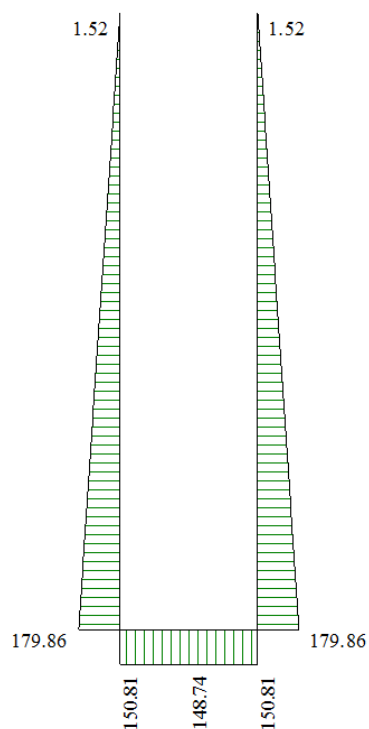
Figura 16 - Diagramma involuppo sforzo normale - SLE
