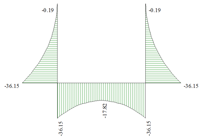
Figura 17 - Diagramma involuppo momento flettente – SLU
