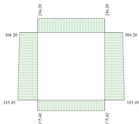
Figura 10 - Diagramma involuppo sforzo normale - SLE
