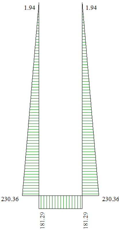
Figura 15 - Diagramma involuppo sforzo normale – SLU
