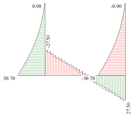
Figura 20 - Diagramma involuppo taglio – SLE
