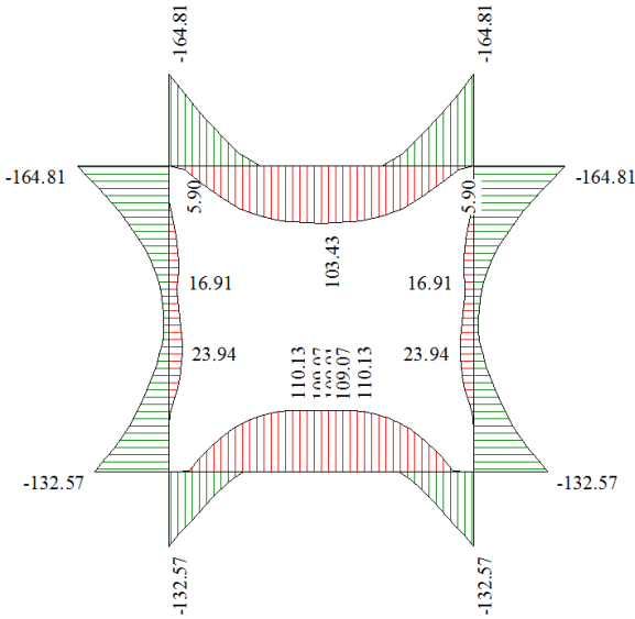
Figura 6 - Diagramma involuipo momento flettente – SLE
