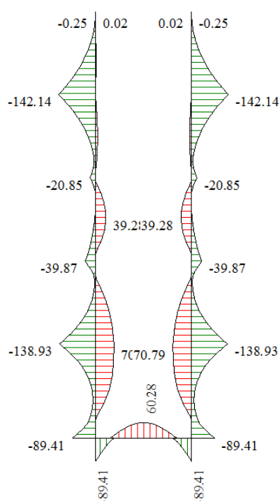
Figura 11 - Diagramma involuppo momento flettente – SLU
