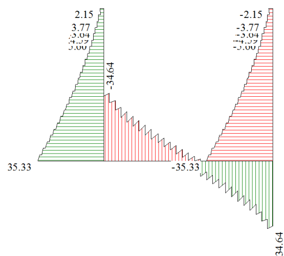
Figura 19 - Diagramma involuppo taglio – SLU
