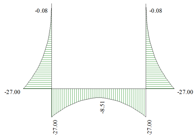
Figura 18 - Diagramma involuppo momento flettente – SLE
