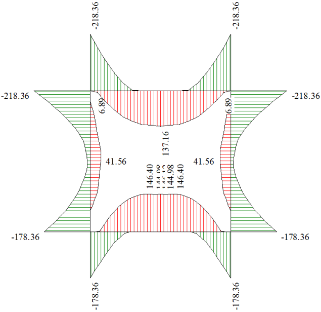
Figura 5 - Diagramma involuipo momento flettente – SLU
