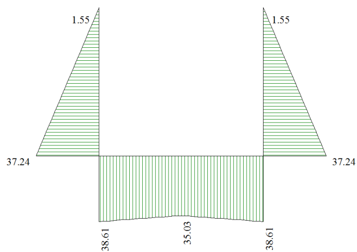
Figura 21 - Diagramma involuppo sforzo normale – SLU
