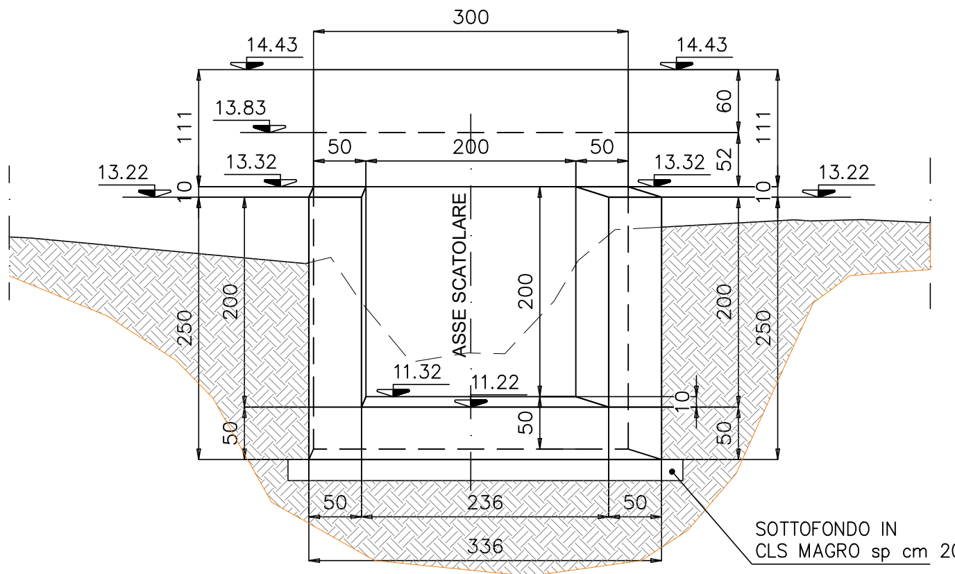
PROSPETTO C-C scala 1:50
