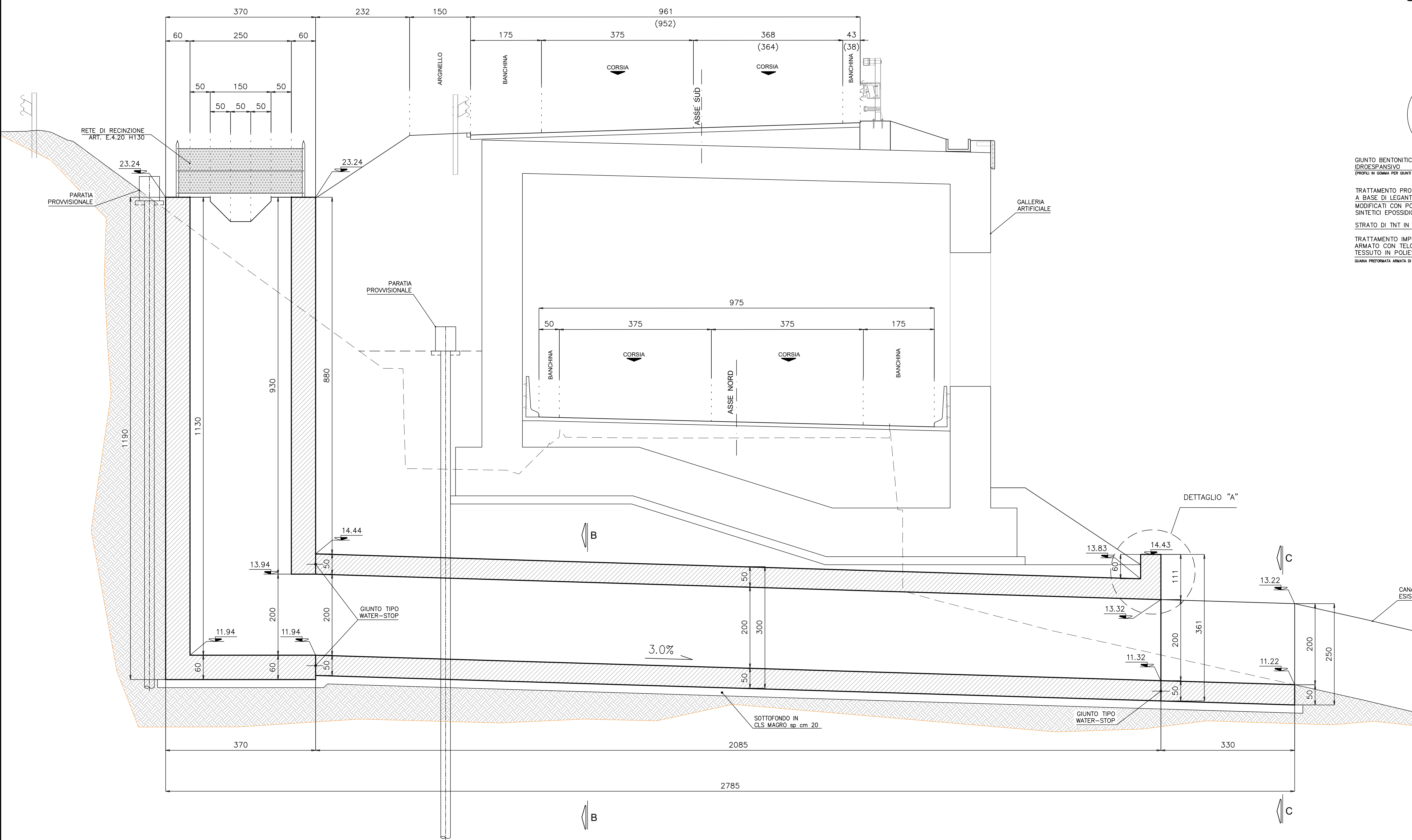
SEZIONE LONGITUDINALE A-A scala 1:50
