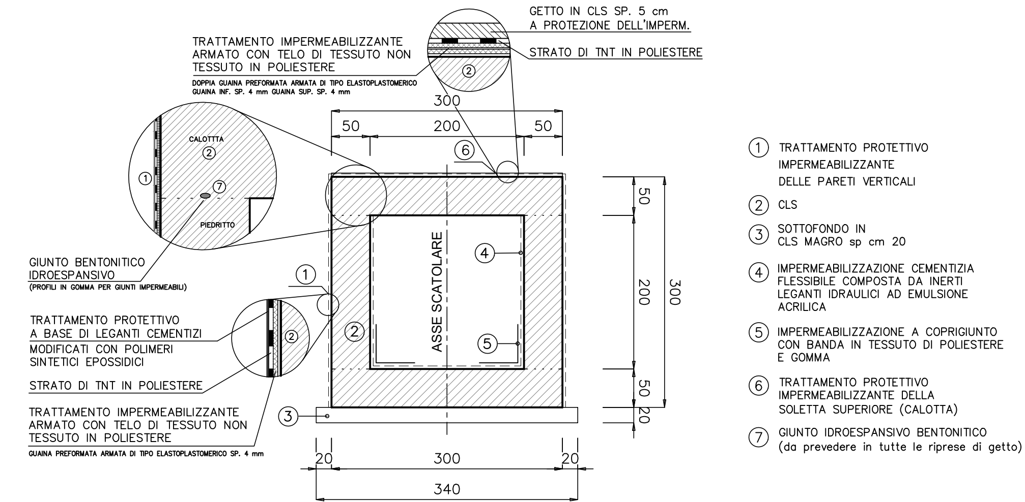
SEZIONE TRASVERSALE B-B scala 1:50
