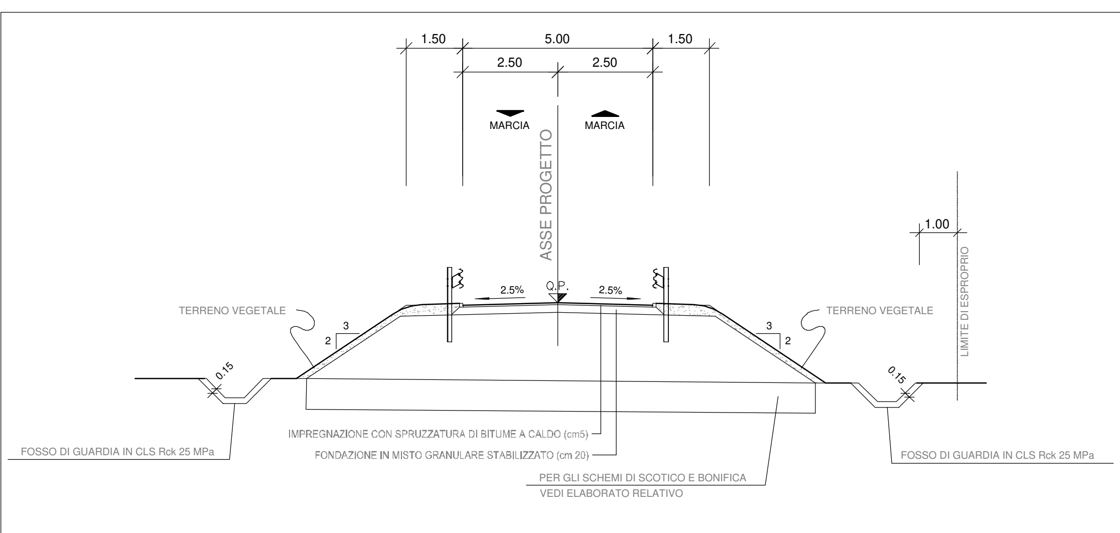
SEZIONE TIPO VP4b scala 1:100
