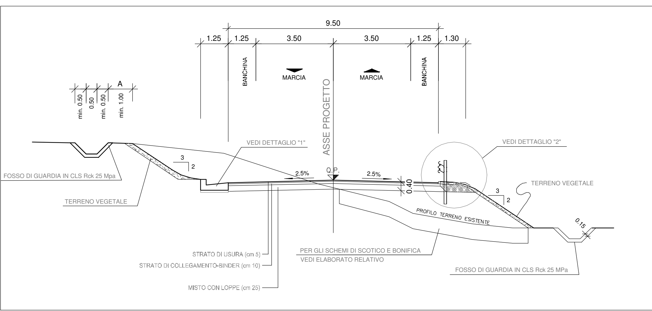
SEZIONE TIPO VP4a scala 1:100
