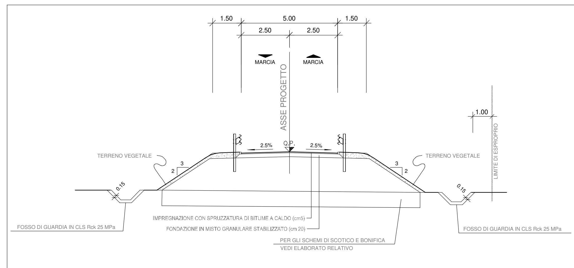
SEZIONE TIPO VP6b scala 1:100
