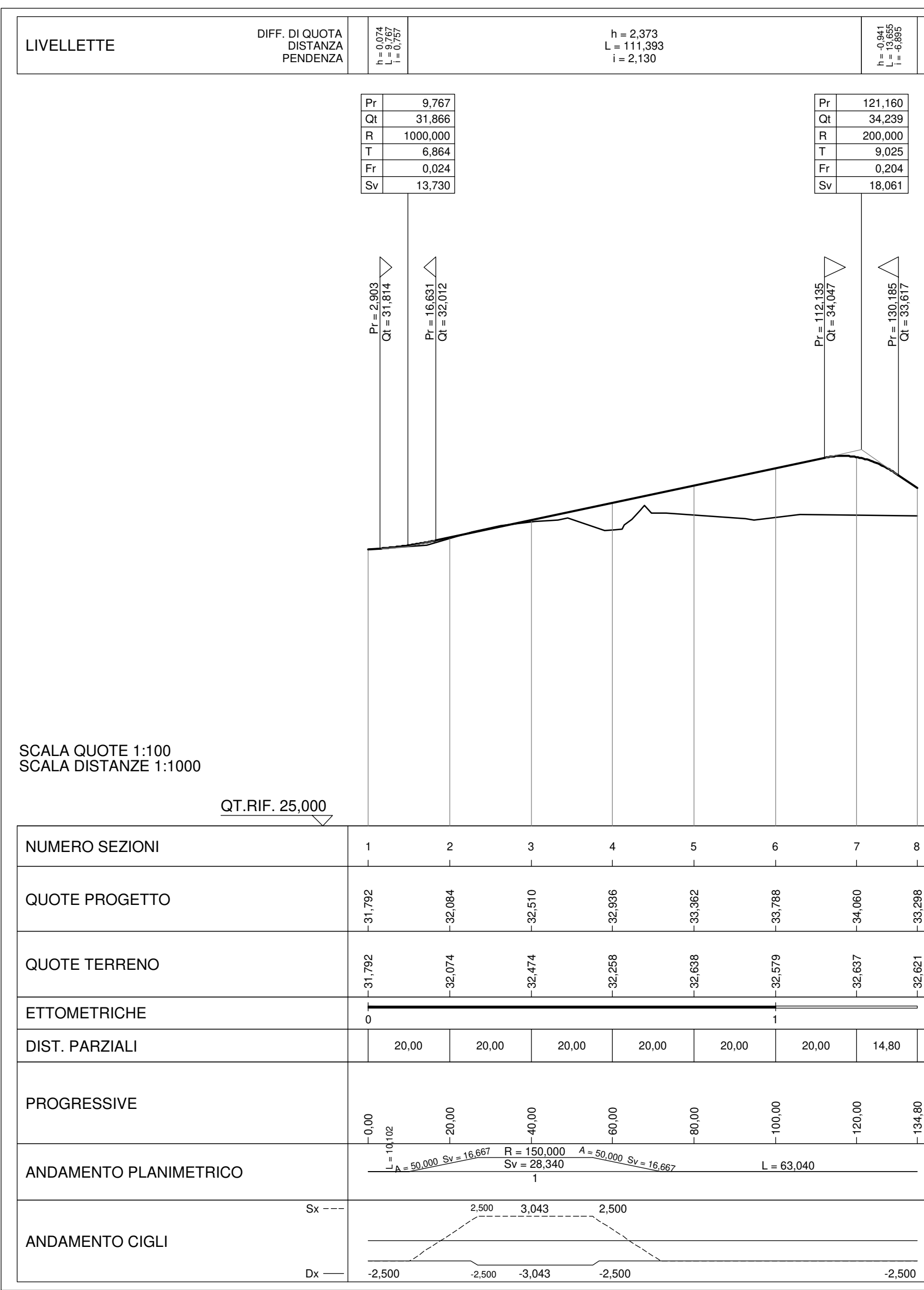
PROFILO LONGITUDINALE VP6b scala 1:1000/1:100
