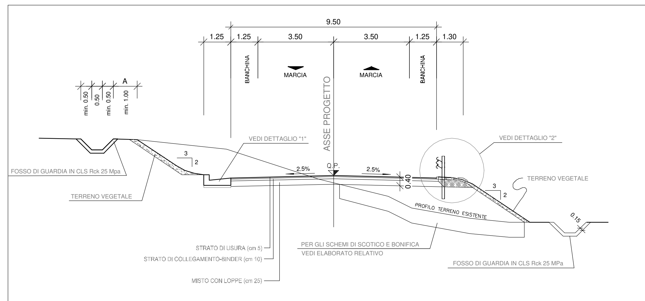
SEZIONE TIPO VP6a scala 1:100
