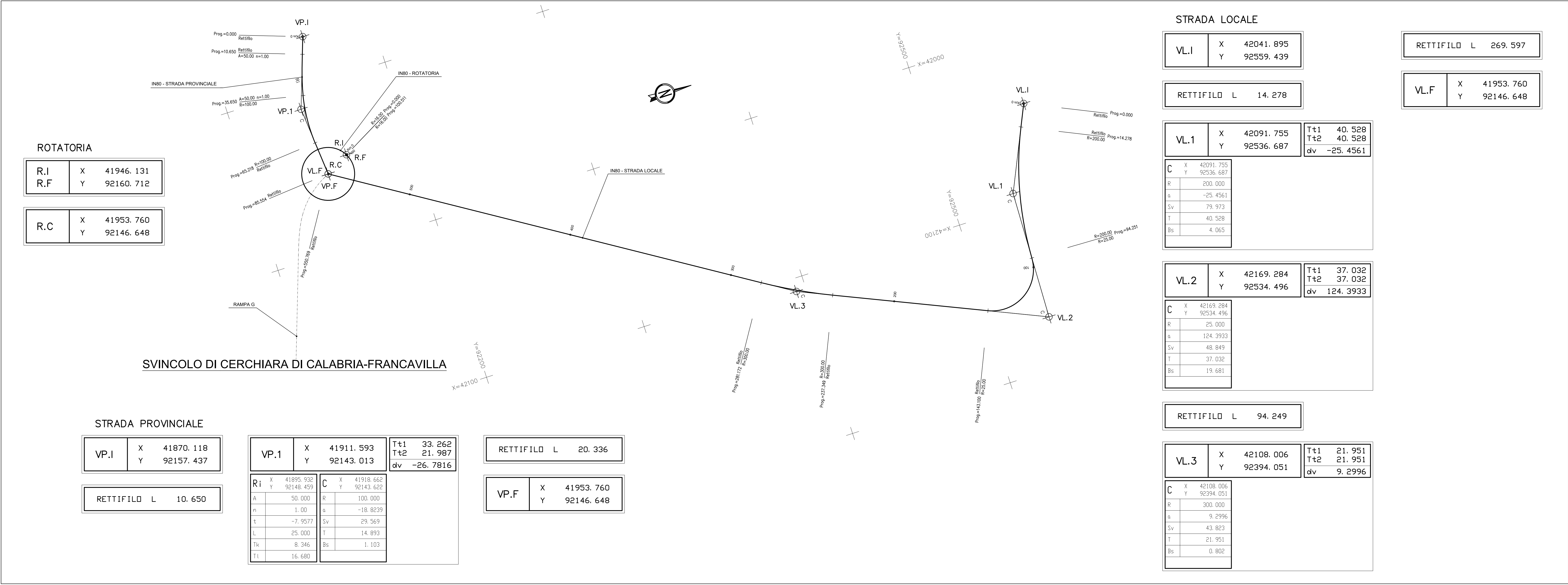
PLANIMETRIA DI TRACCIAMENTO scala 1:1000
