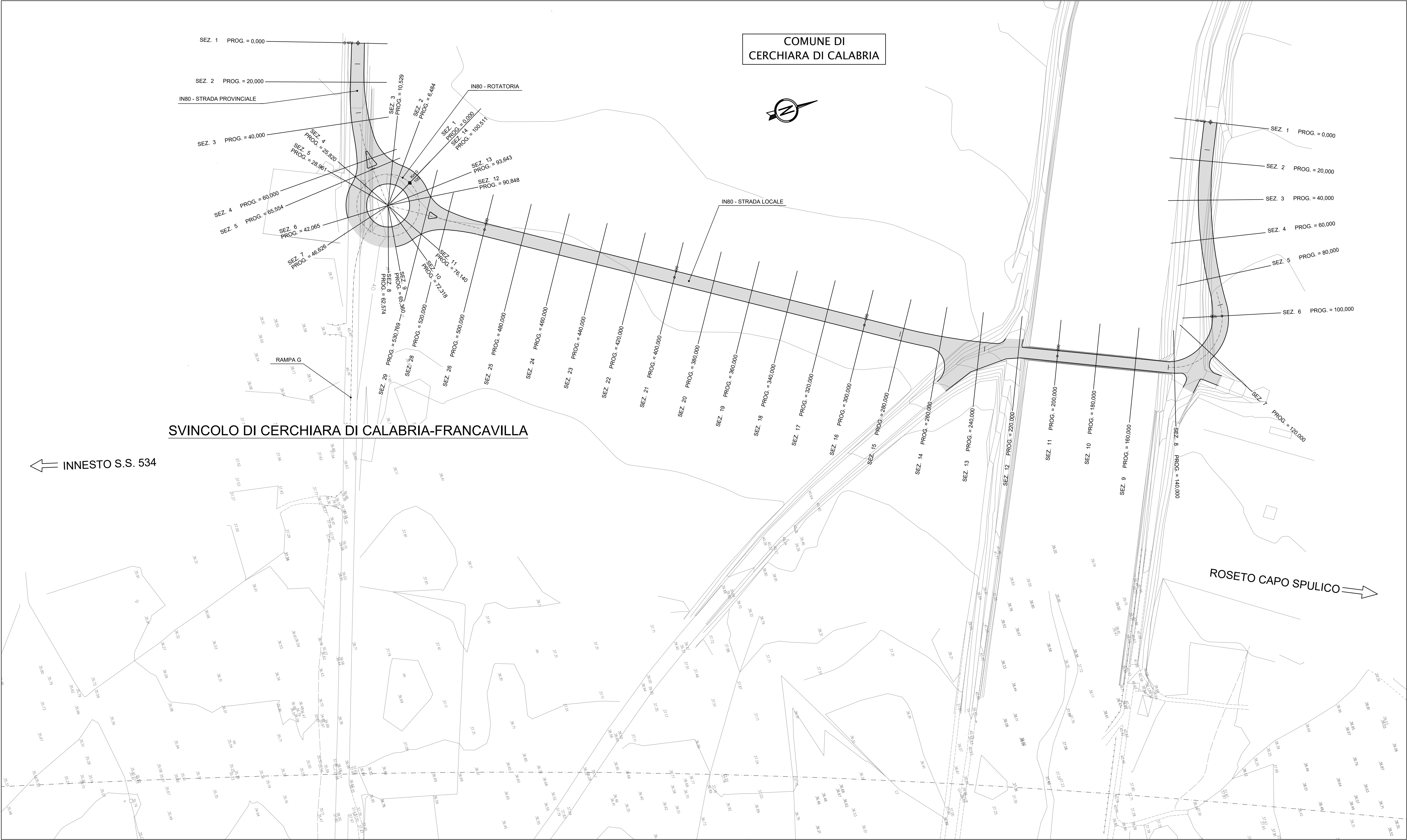
PLANIMETRIA DI TRACCIAMENTO scala 1:1000
