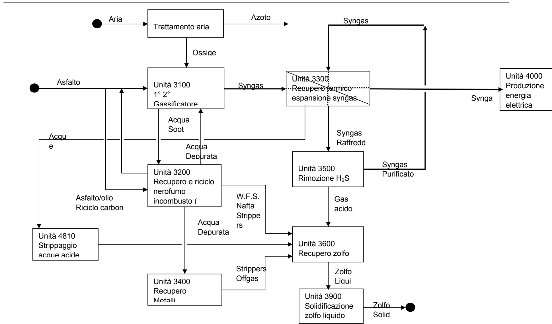
Figura 5.2b Schema a Blocchi dell'Impianto IGCC nella Situazione Ante Operam
