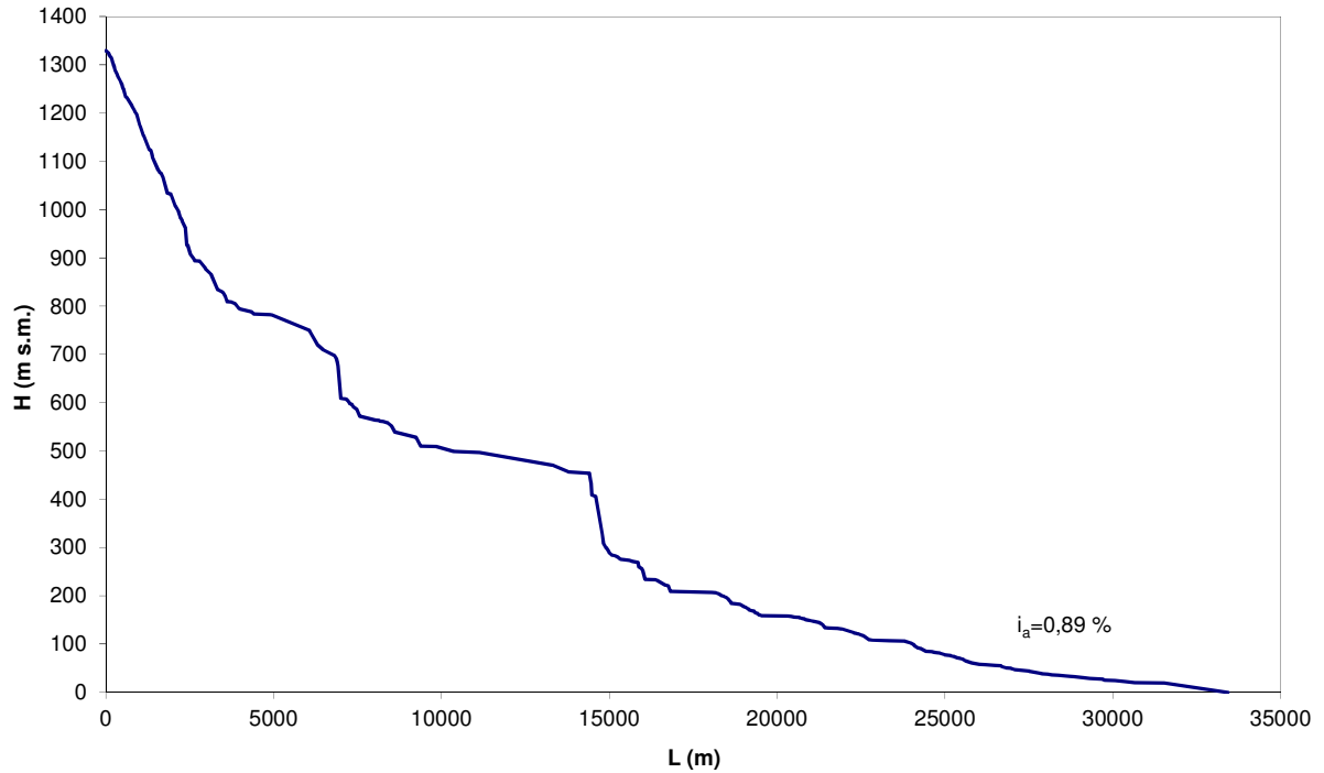
Fig. 3. Profilo longitudinale dell'asta principale del bacino del Torrente Raganello.
