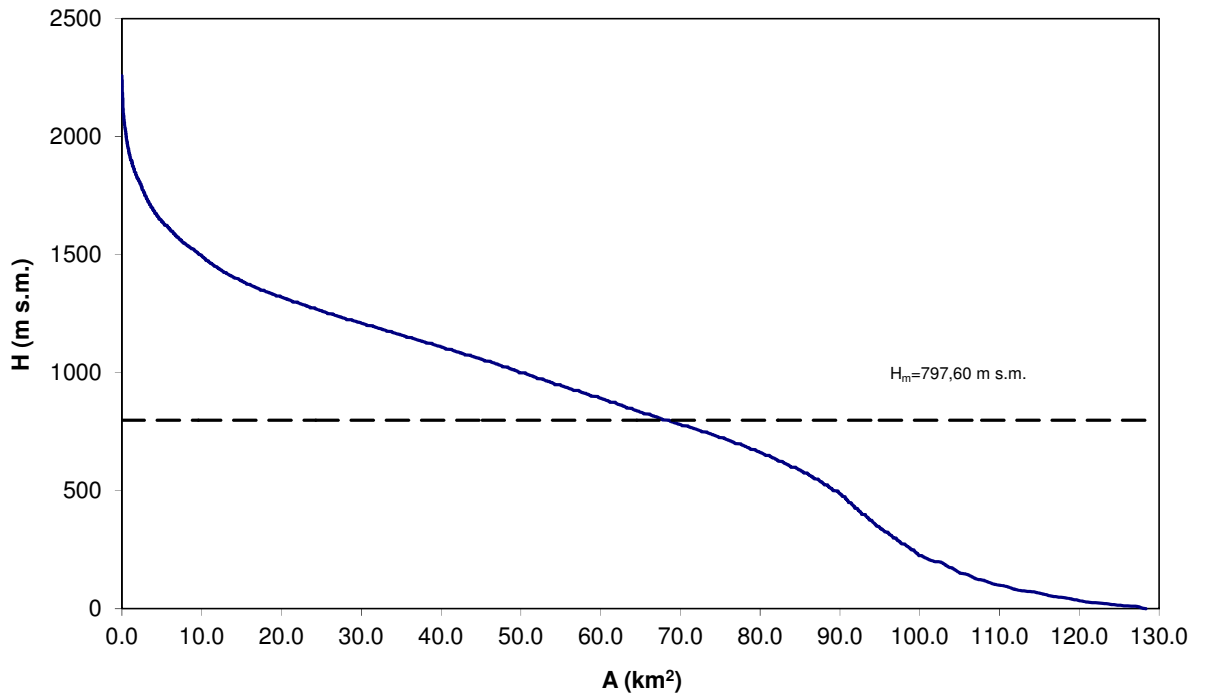
Fig. 2. Curva ipsografica del bacino del Torrente Raganello.
