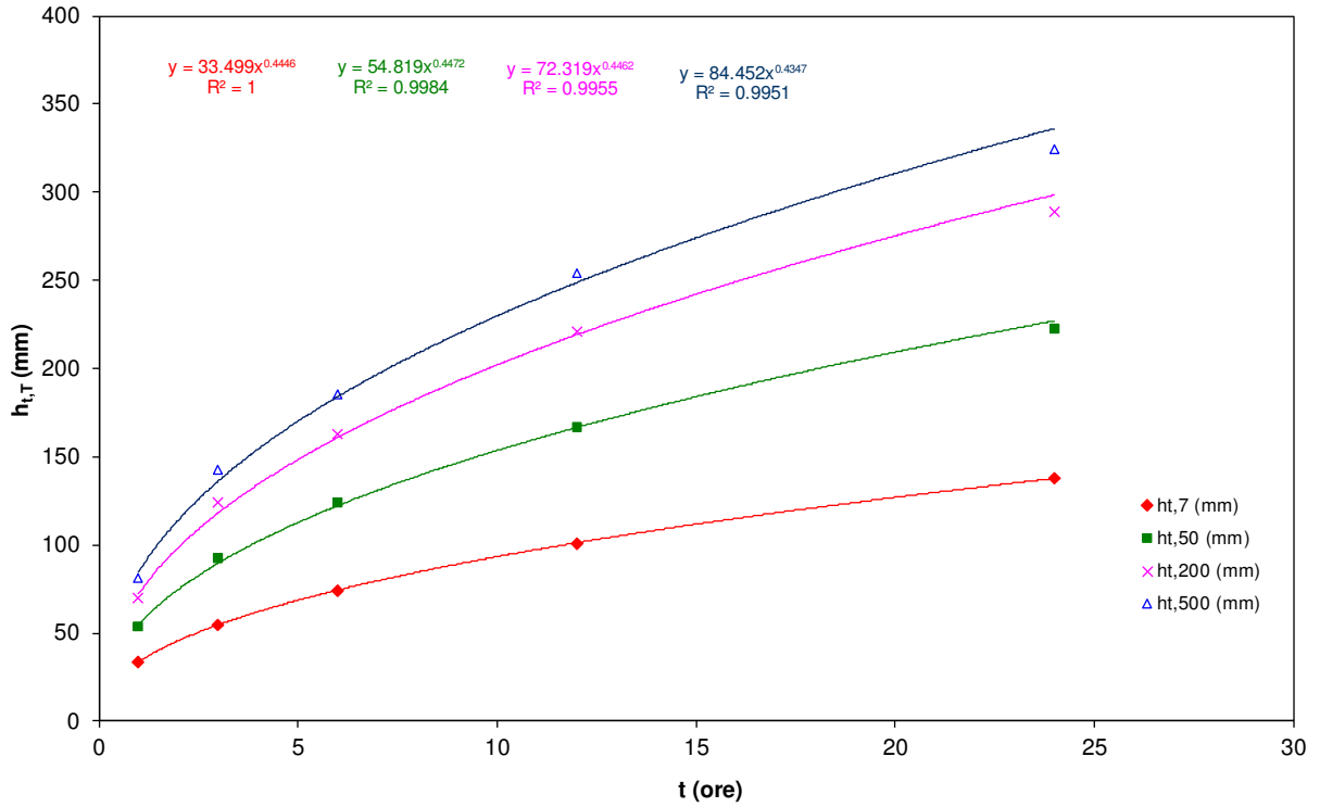
Fig. 4. Curve di probabilità pluviometrica per il bacino in esame del Torrente Raganello calcolata al terzo livello di regionalizzazione.
