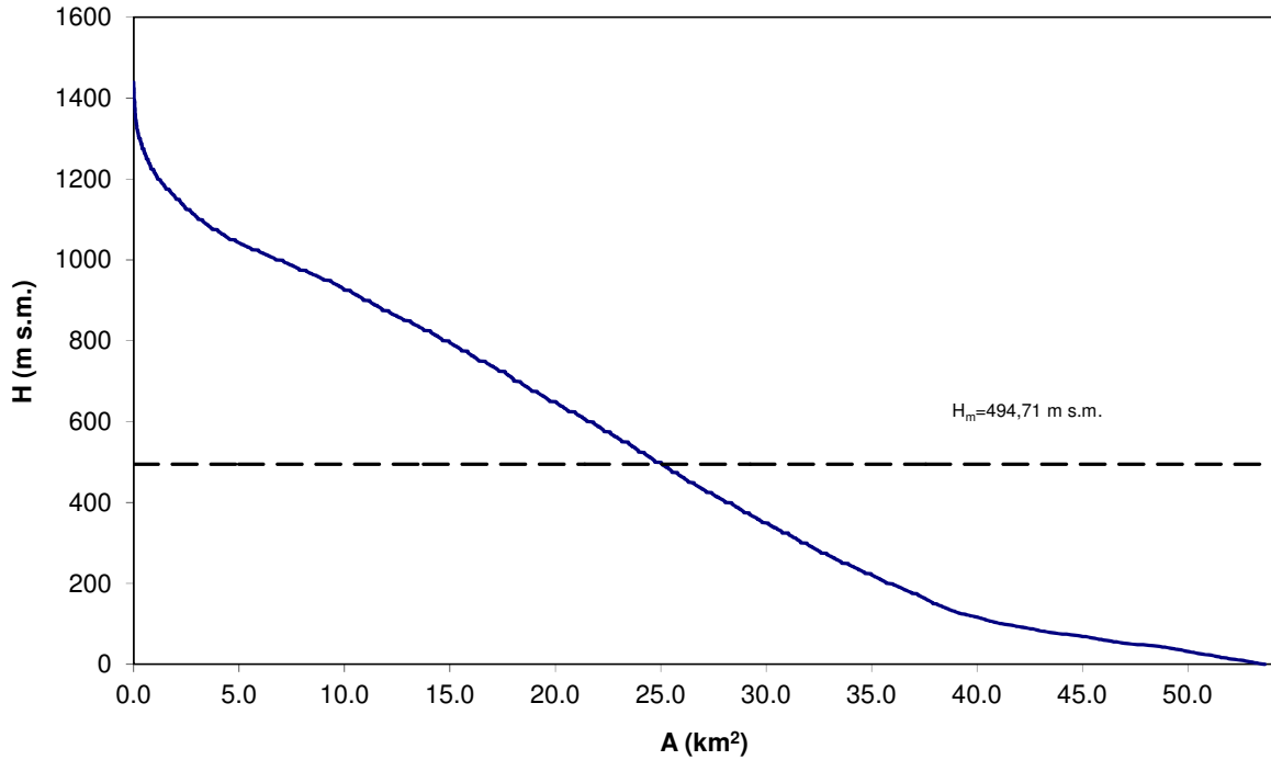
Fig. 2. Curva ipsografica del bacino del Torrente Caldana.
