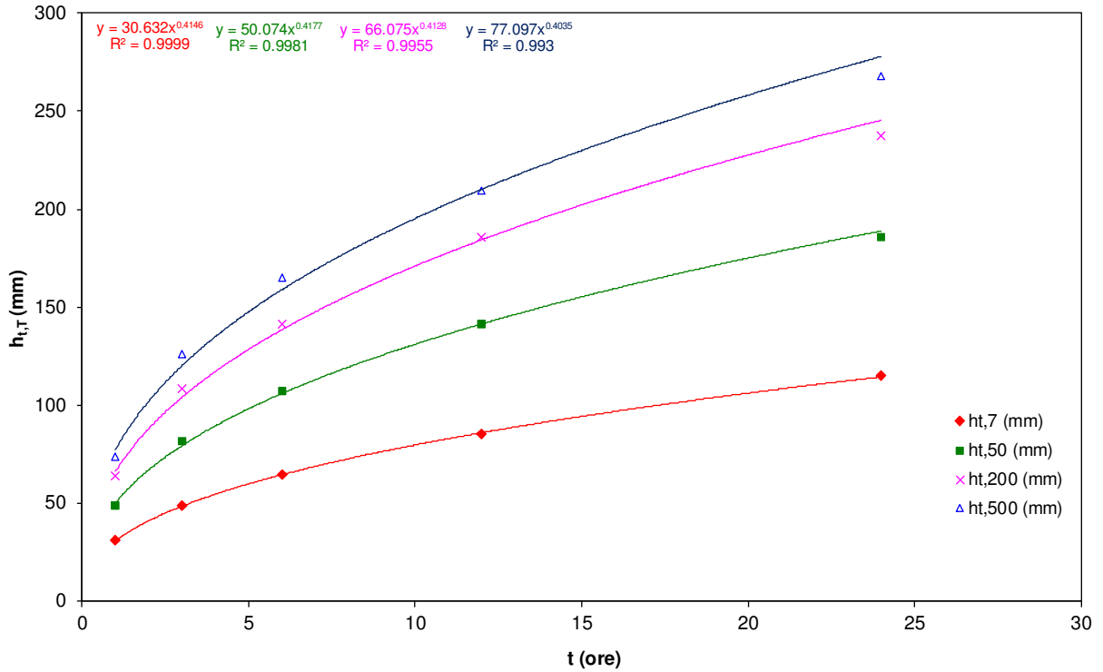
Fig. 4. Curve di probabilità pluviometrica per il bacino in esame del Torrente Caldana calcolata al terzo livello di regionalizzazione.
