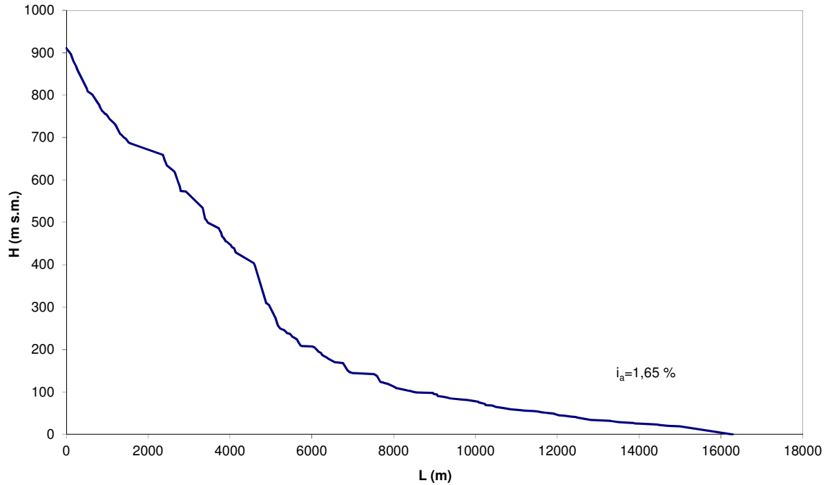
Fig. 3. Profilo longitudinale dell'asta principale del bacino del Torrente Caldana.
