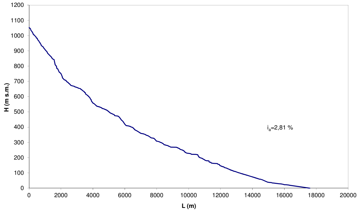
Fig. 3. Profilo longitudinale dell'asta principale del bacino del Torrente Satanasso.
