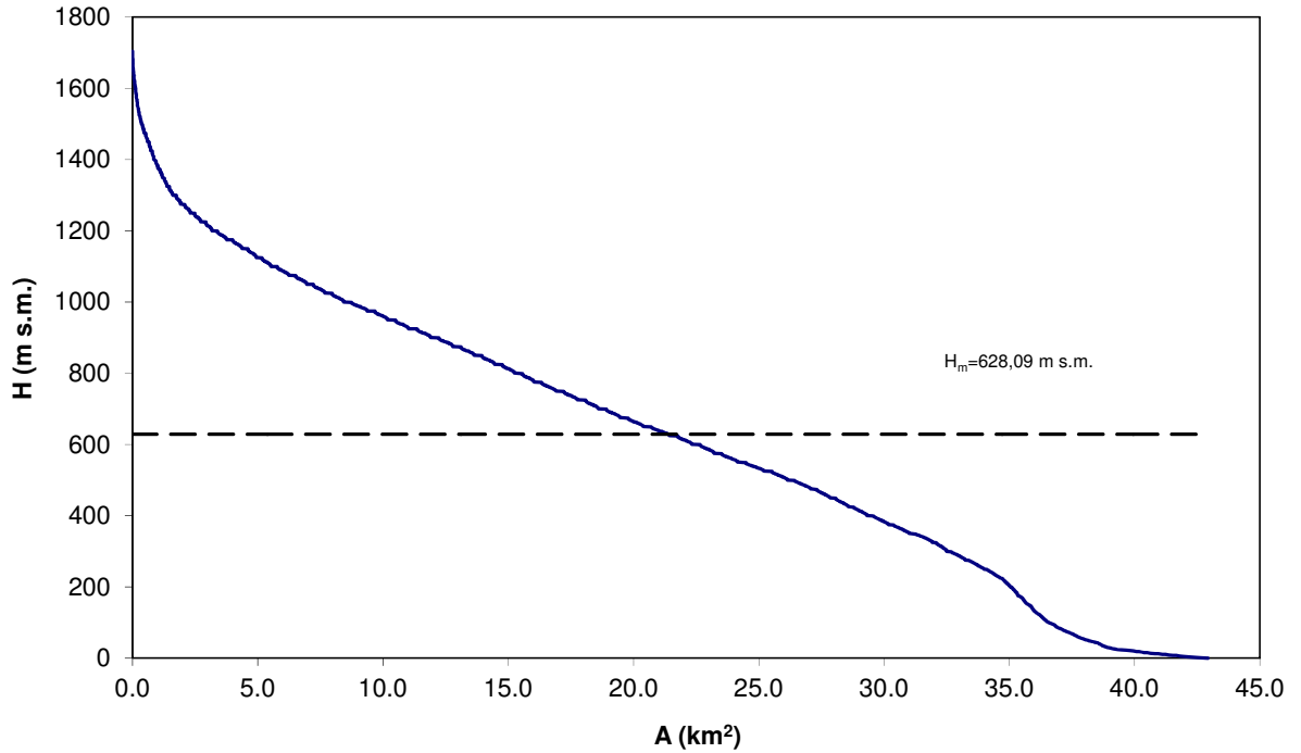
Fig. 2. Curva ipsografica del bacino del Torrente Satanasso.
