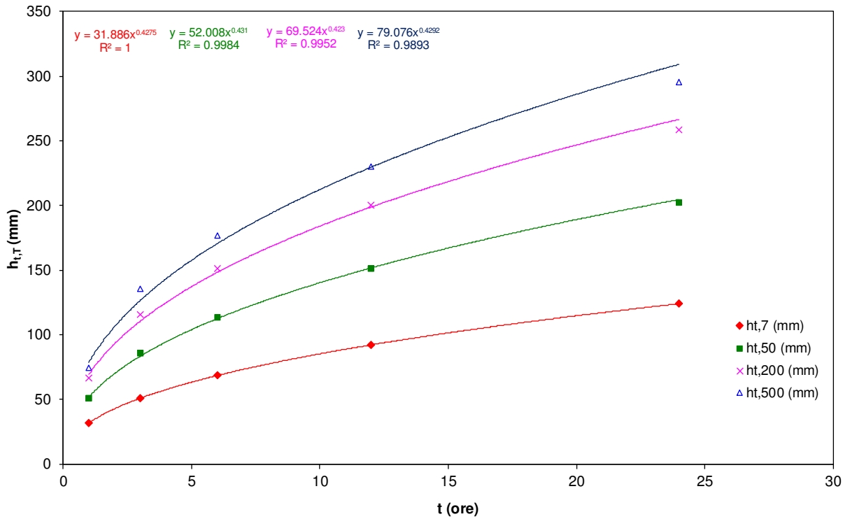
Fig. 4. Curve di probabilità pluviometrica per il bacino in esame del Torrente Satanasso calcolata al terzo livello di regionalizzazione.
