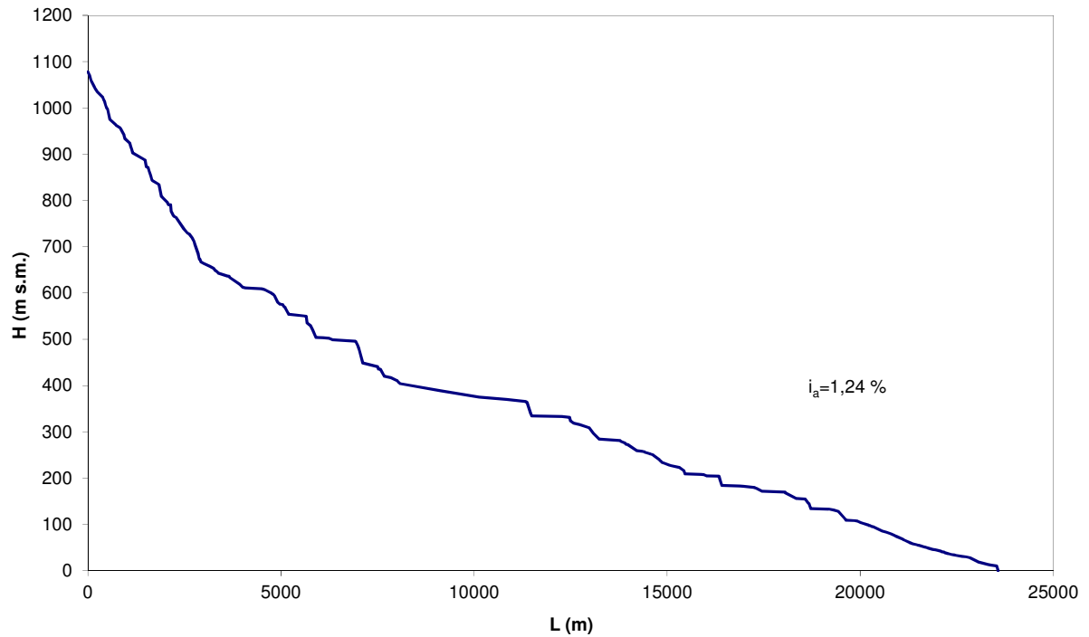
Fig. 3. Profilo longitudinale dell'asta principale del bacino del Torrente Saraceno.
