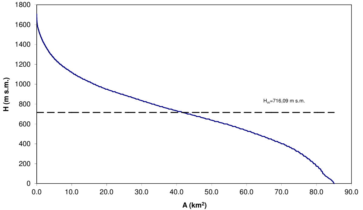
Fig. 2. Curva ipsografica del bacino del Torrente Saraceno.
