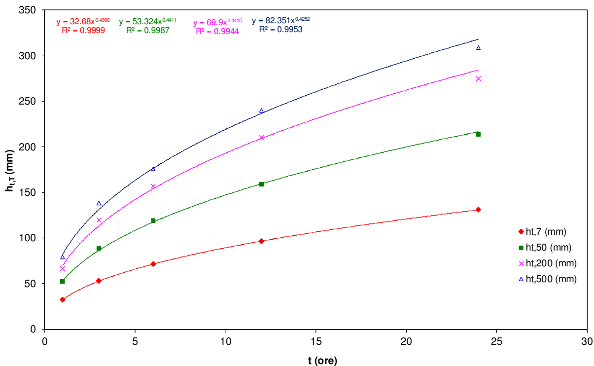
Fig. 4. Curve di probabilità pluviometrica per il bacino in esame del Torrente Saraceno calcolata al terzo livello di regionalizzazione.
