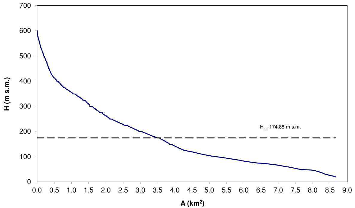
Fig. 2. Curva ipsografica del bacino del Torrente Castiglione.
