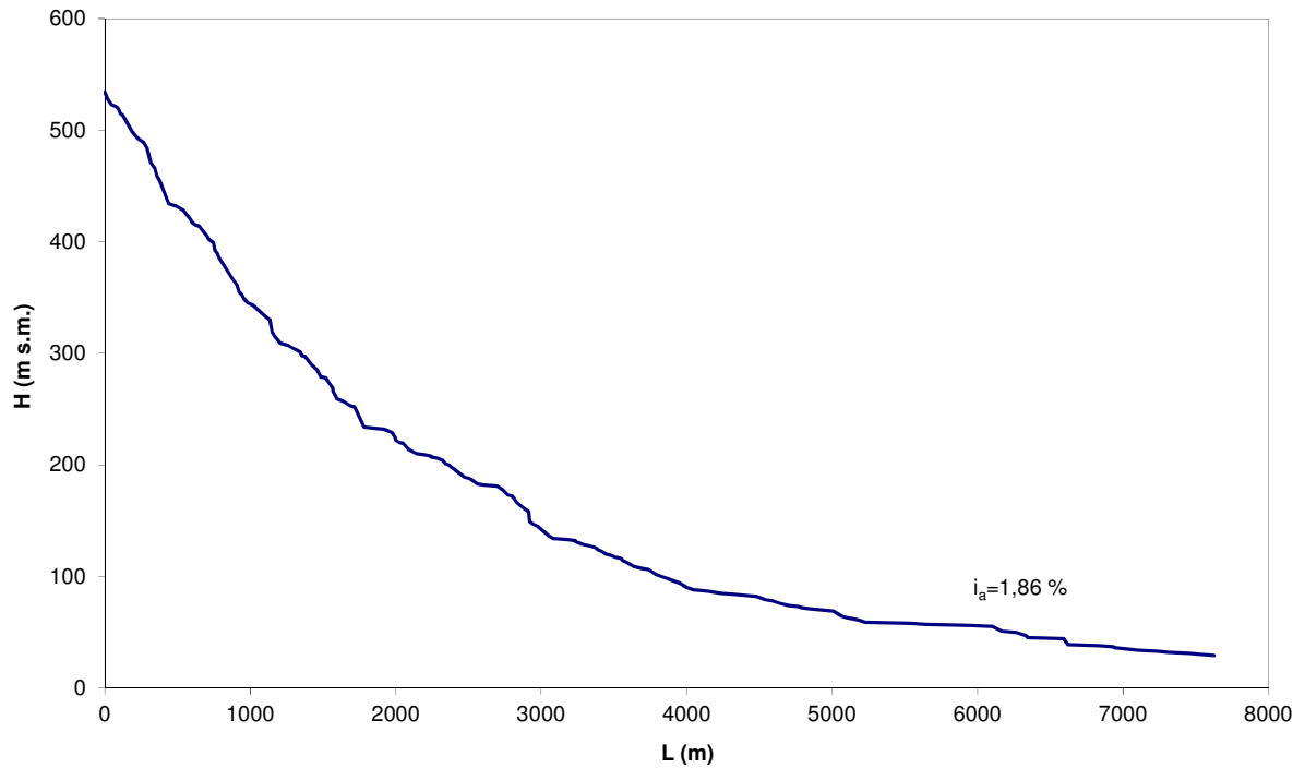
Fig. 3. Profilo longitudinale dell'asta principale del bacino del Torrente Castiglione.
