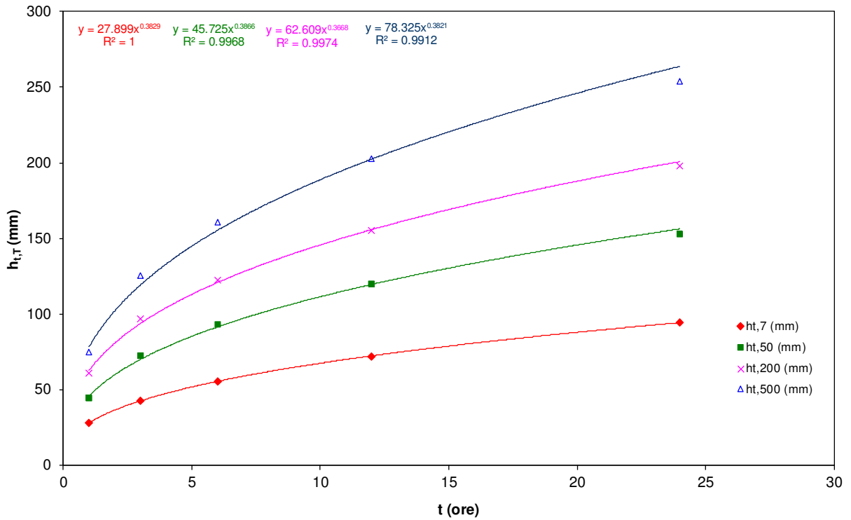
Fig. 4. Curve di probabilità pluviometrica per il bacino in esame del Torrente Castiglione calcolata al terzo livello di regionalizzazione.
