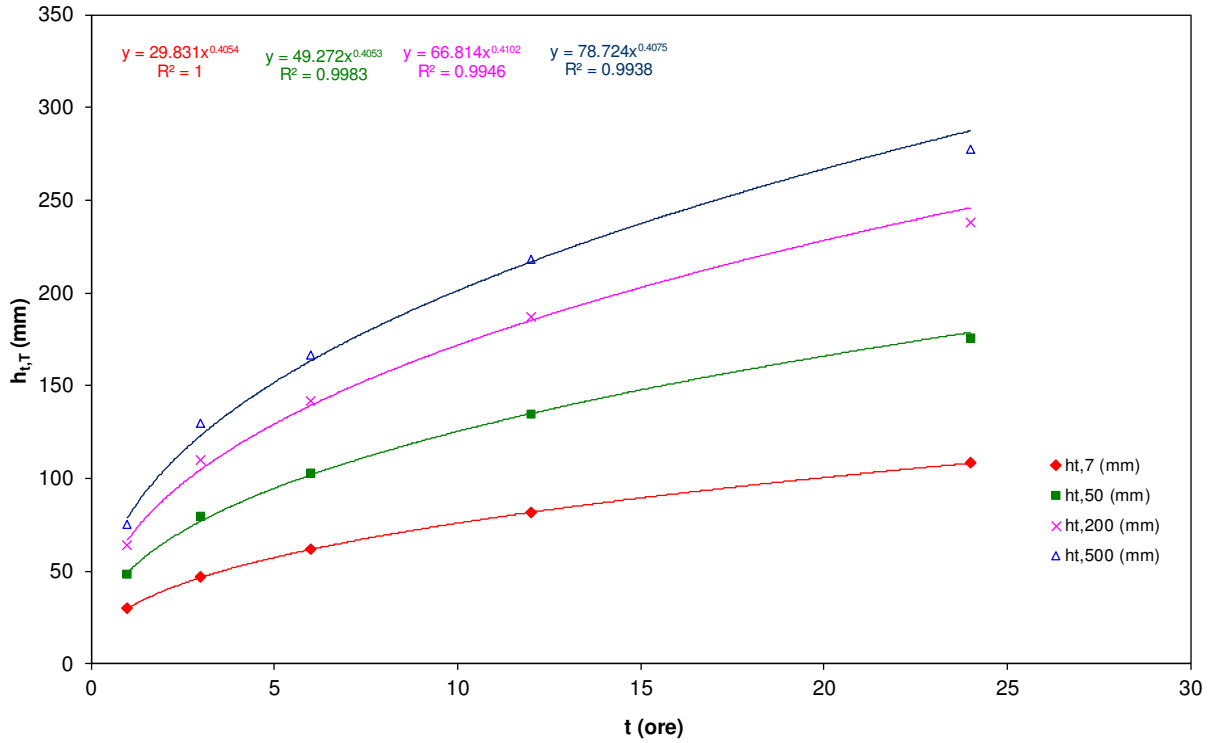
Fig. 4. Curve di probabilità pluviometrica per il bacino in esame del Torrente Pagliaro calcolata al terzo livello di regionalizzazione.
