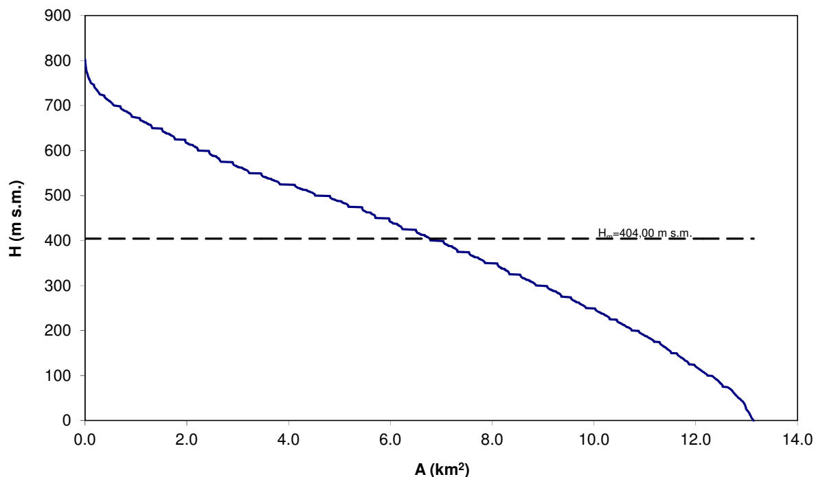
Fig. 2. Curva ipsografica del bacino del Torrente Pagliaro.
