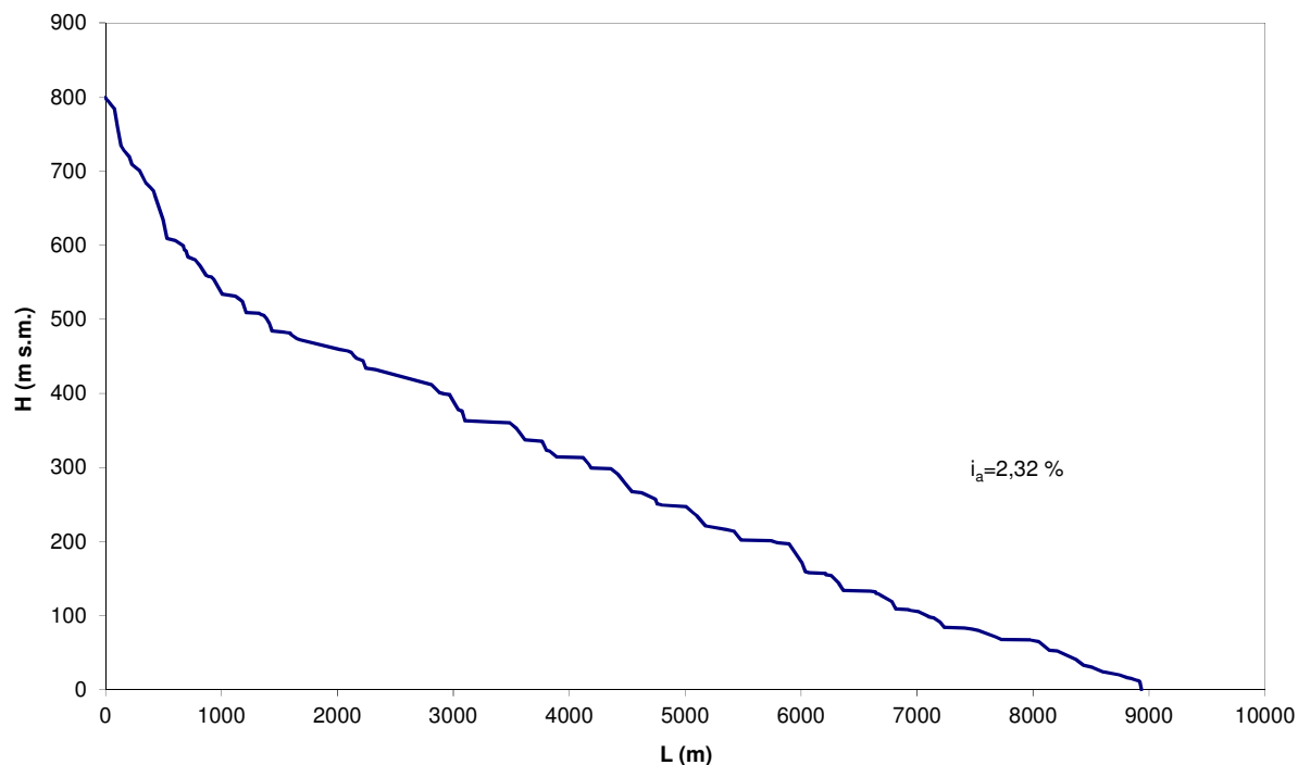
Fig. 3. Profilo longitudinale dell'asta principale del bacino del Torrente Pagliaro.
