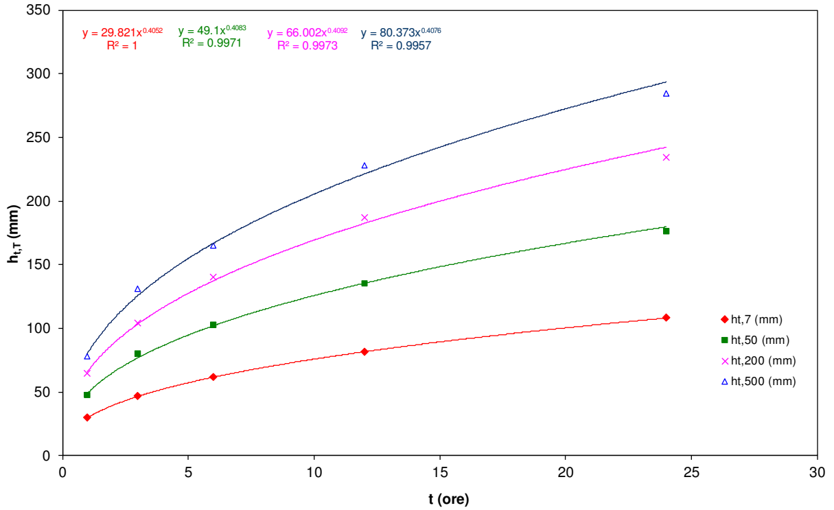
Fig. 4. Curve di probabilità pluviometrica per il bacino in esame del Torrente Avena calcolata al terzo livello di regionalizzazione.
