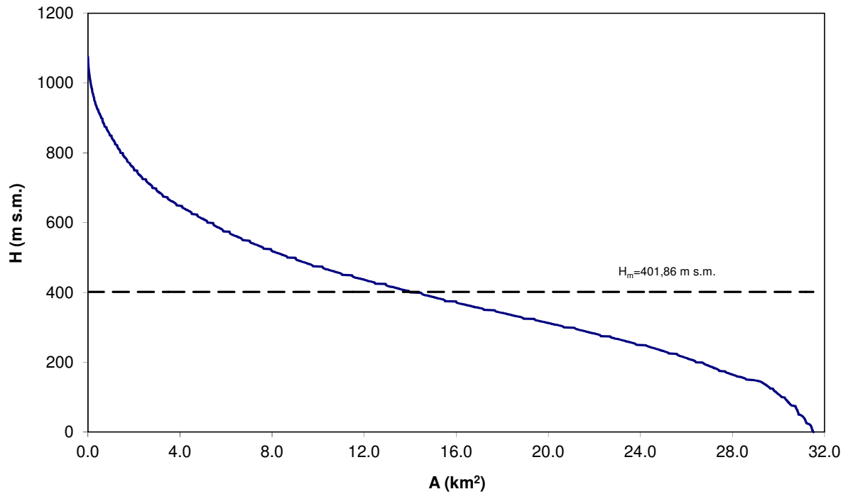
Fig. 2. Curva ipsografica del bacino del Torrente Avena.
