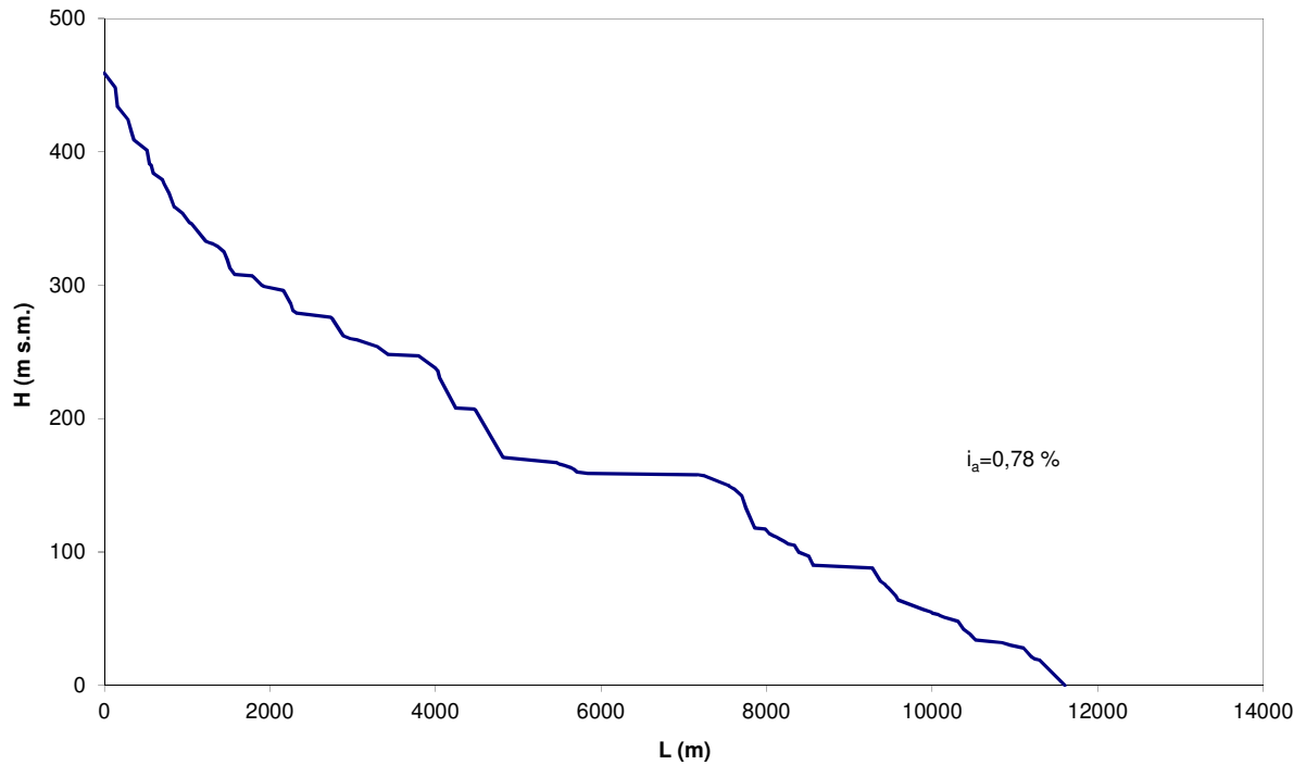
Fig. 3. Profilo longitudinale dell'asta principale del bacino del Torrente Avena.
