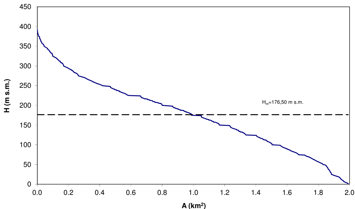
Fig. 2. Curva ipsografica del bacino del Torrente Angeloni.
