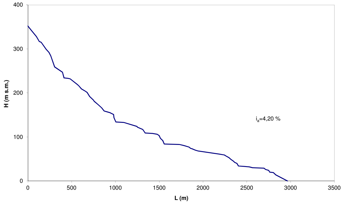
Fig. 3. Profilo longitudinale dell'asta principale del bacino del Torrente Angeloni.
