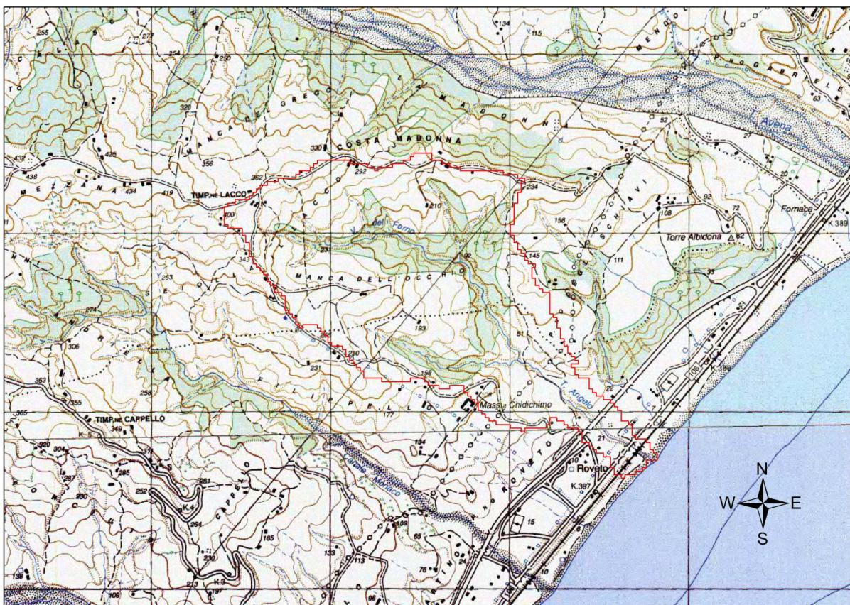
Fig. 1. Corografia del bacino del Torrente Angeloni.
