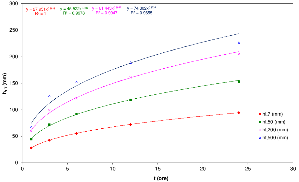
Fig. 4. Curve di probabilità pluviometrica per il bacino in esame del Torrente Angeloni calcolata al terzo livello di regionalizzazione.
