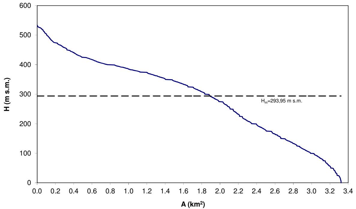
Fig. 2. Curva ipsografica del bacino del Fosso Annunziata.
