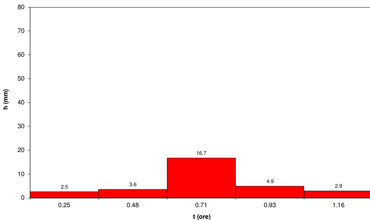
Fig. 5. Pluviogramma di calcolo per T=7 anni.
