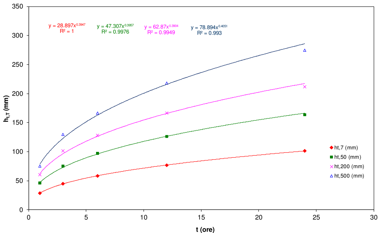
Fig. 4. Curve di probabilità pluviometrica per il bacino in esame del Fosso Annunziata calcolata al terzo livello di regionalizzazione.
