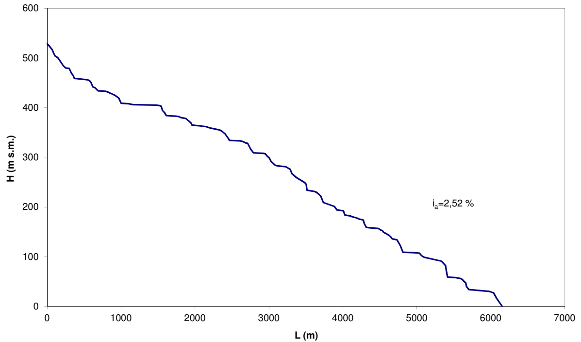
Fig. 3. Profilo longitudinale dell'asta principale del bacino del Fosso Annunziata.
