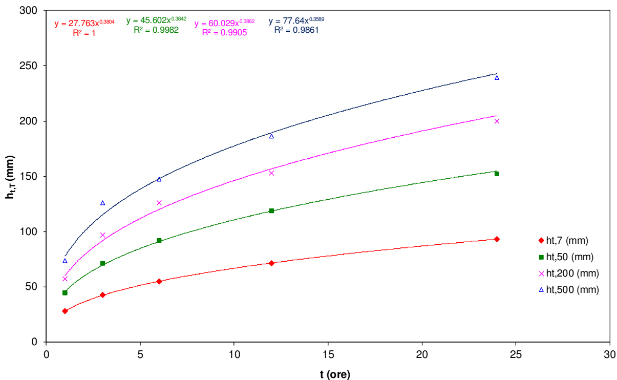
Fig. 4. Curve di probabilità pluviometrica per il bacino in esame del Torrente Della Donna calcolata al terzo livello di regionalizzazione.
