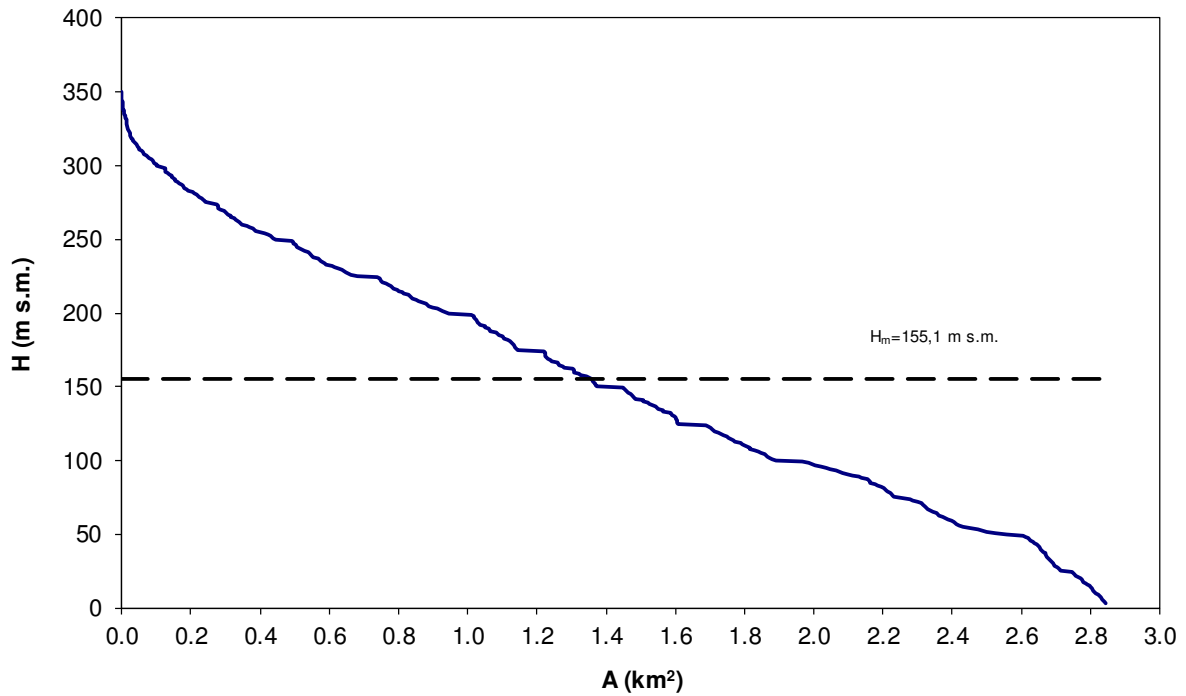
Fig. 2. Curva ipsografica del bacino del Torrente Della Donna.
