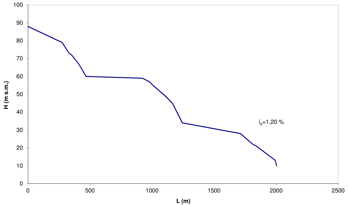
Fig. 3. Profilo longitudinale dell'asta principale del bacino del Torrente Della Donna.
