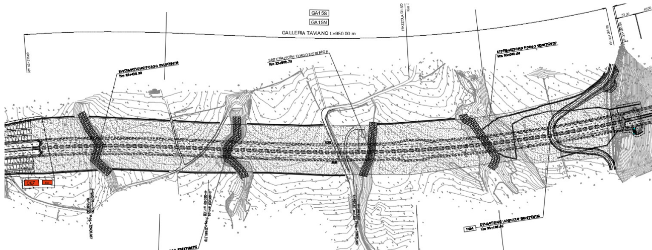
Planimetria
