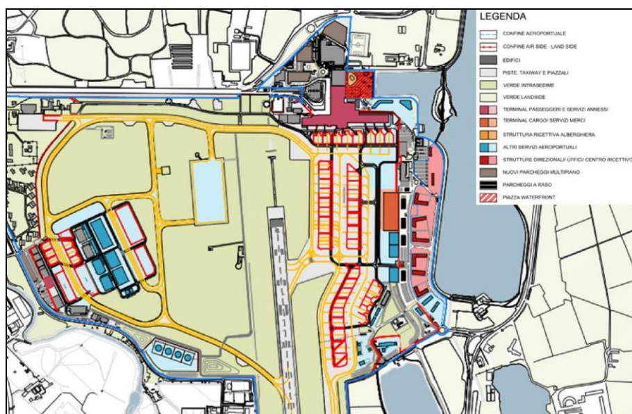
Fig. 1: Configurazione fisica e funzionale aeroportuale di progetto (Fonte: Masterplan)
