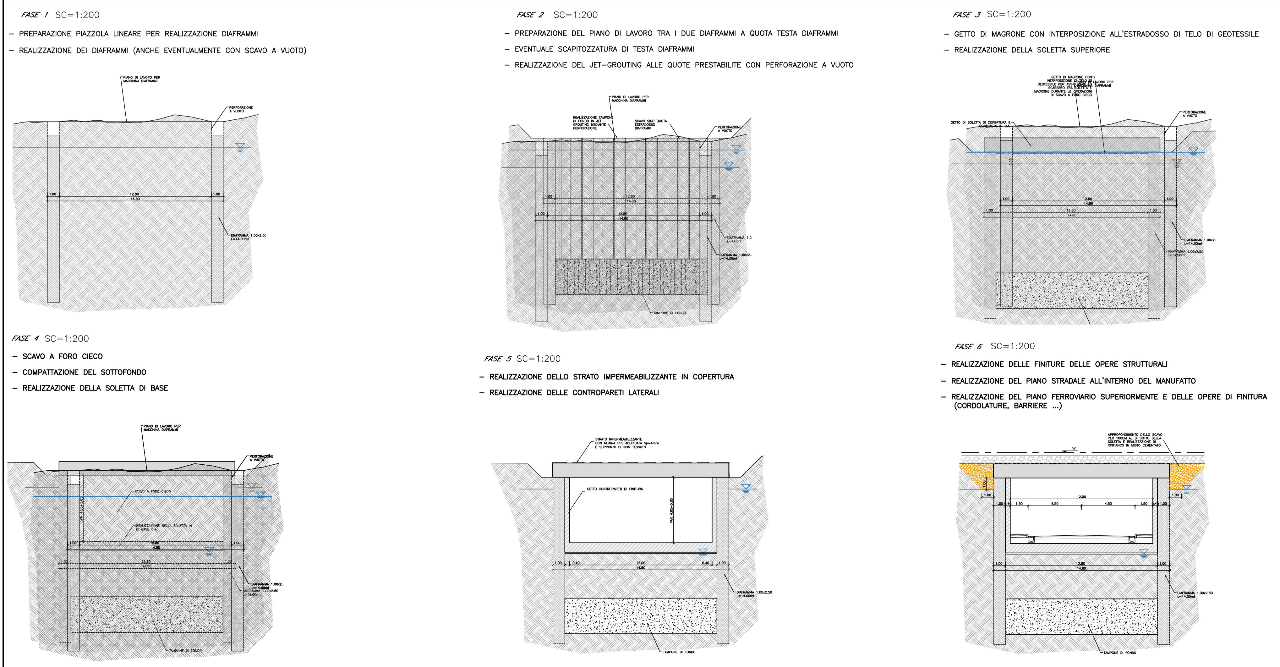
FASI COSTRUTTIVE WBS OC25 - 1:200
