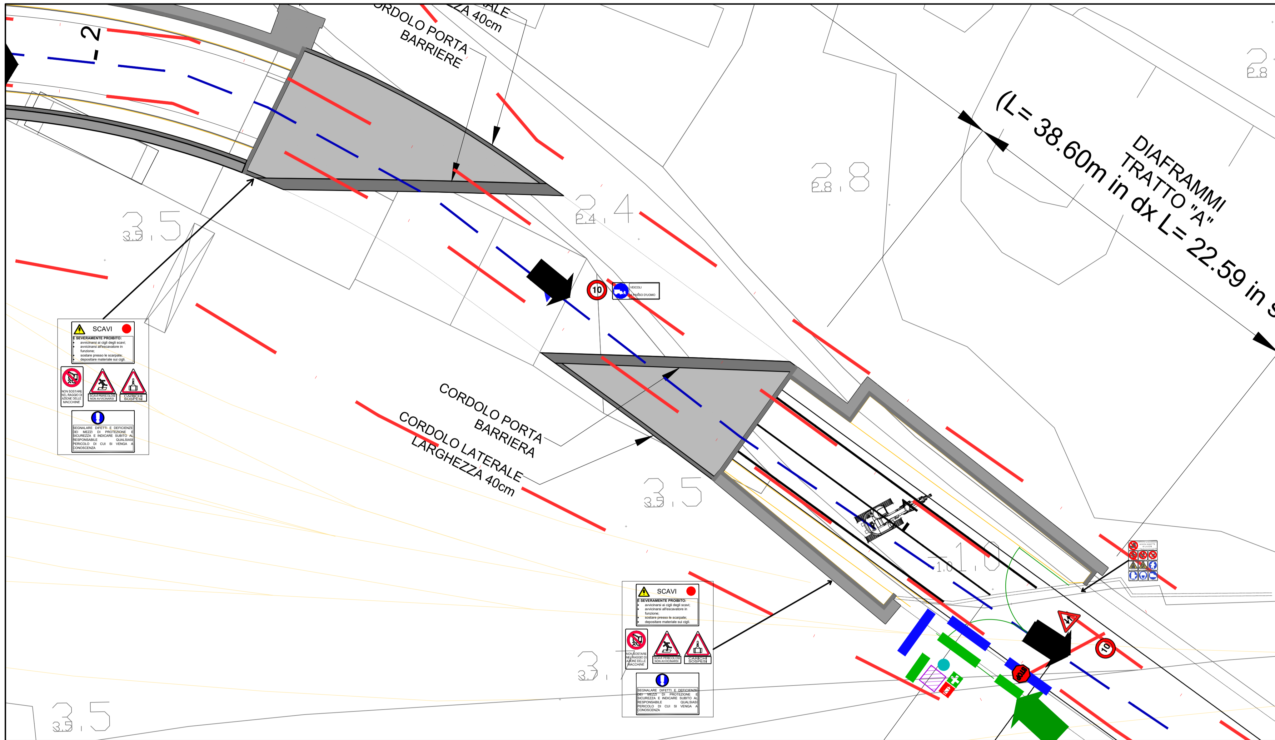
FASI COSTRUTTIVE WBS OC25 - 1:200
