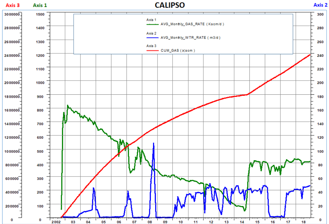
Figura 3 - Campo di Calipso: grafico di produzione storica
