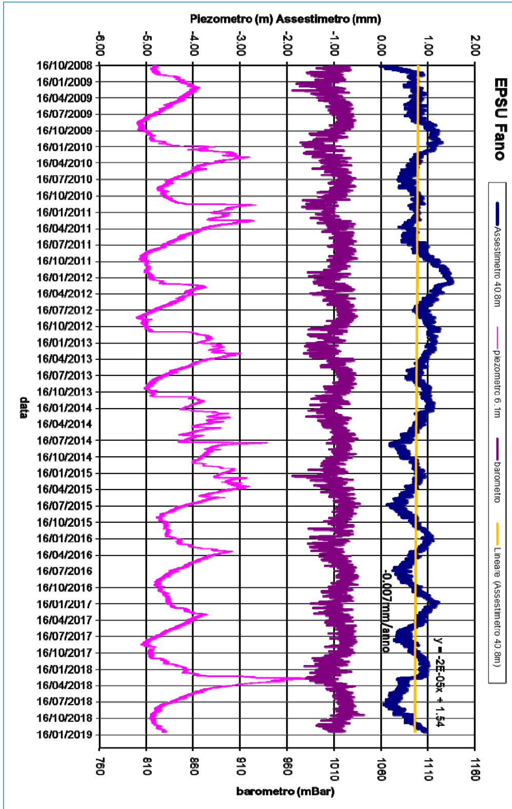
Figura 11B - Stazione EPSU di Fano: misure piezometrico-assestometriche
