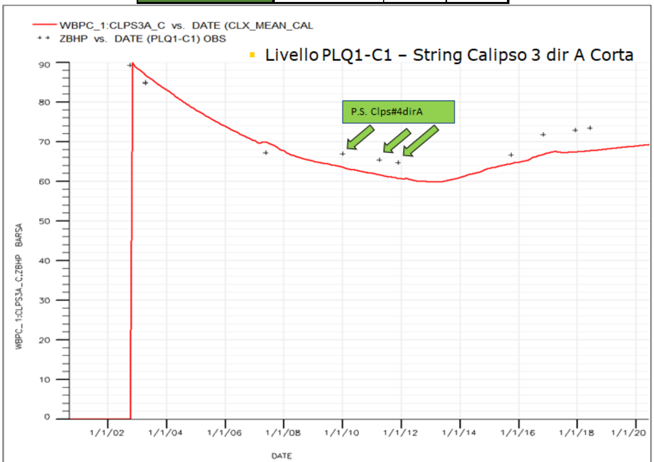
Figura 7 - Campo di Calipso: pressioni statiche misurate e modello Eclipse 2017 (livello PLQ1-C1)
