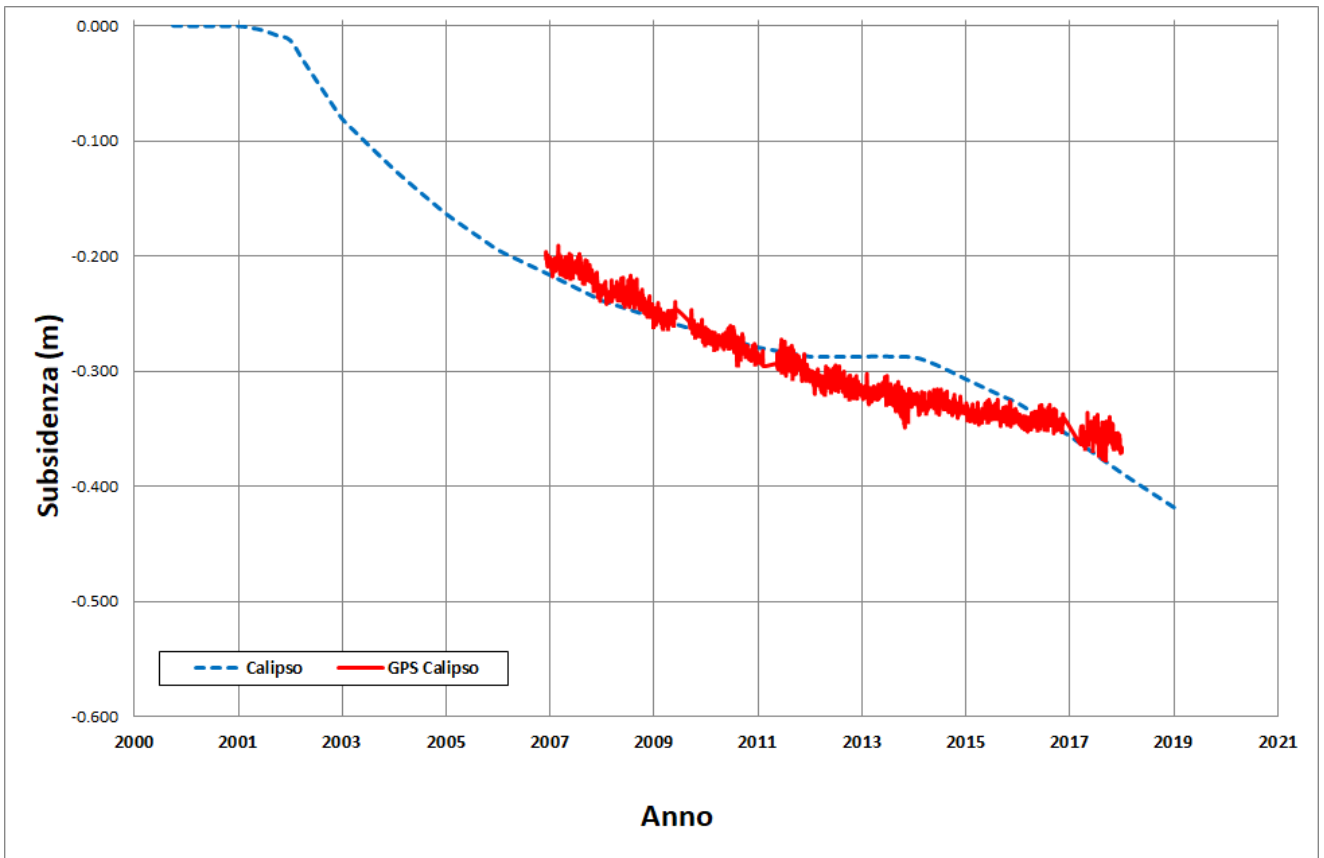
Figura 13 - Calipso: andamento della subsidenza misurata (CGPS in p.ma) vs. modello
