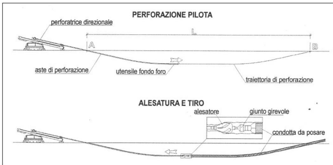
Figura 46 - Fasi tipiche della realizzazione di una TOC
