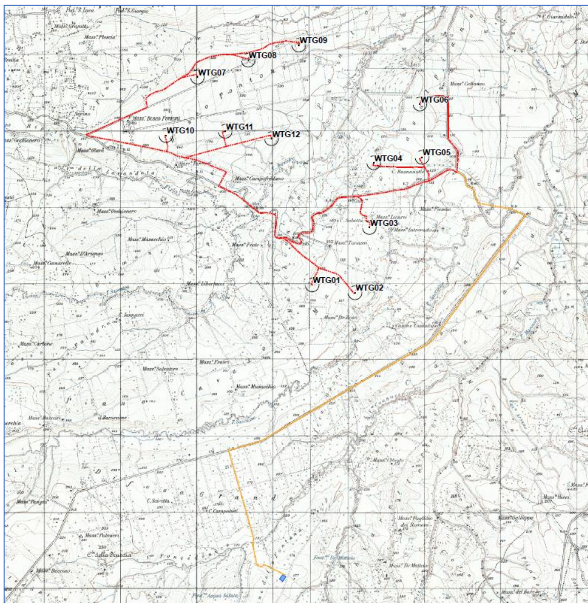
Figura 7 - layout impianto definitivo a n.12 aerogeneratori
