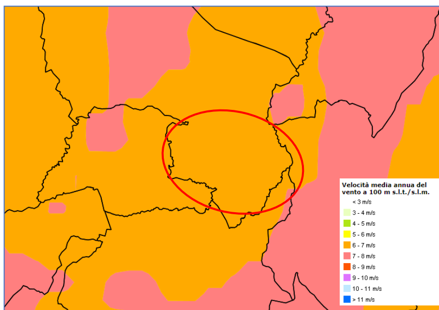
Figura 11 - Velocità media annua del vento a 100 m s.l.m.m - fonte Atlante Eolico
