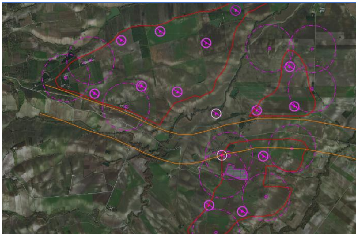
Figura 4 - Ipotesi di layout a 13 aerogeneratori - analisi vincolistica
