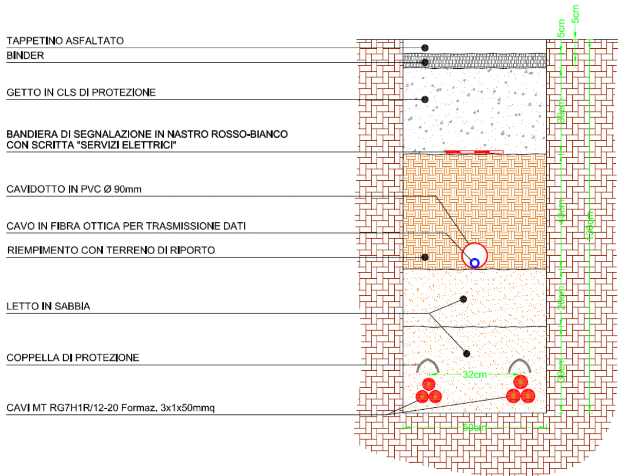
Fig. 5.2 Ipotesi di modalità di posa del caavidotto oggetto dell'analisi
