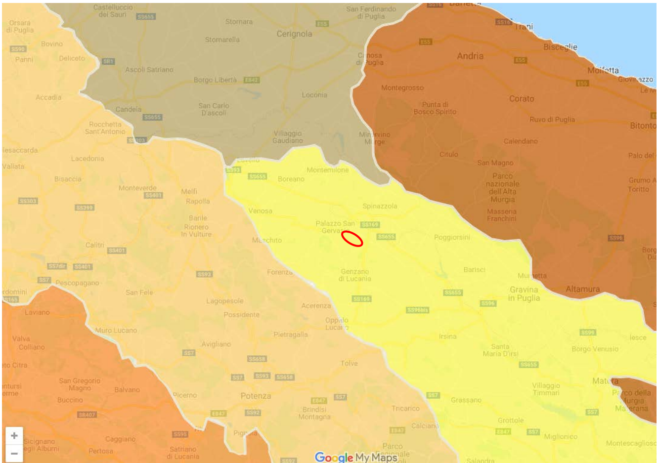
Figure 7-9: regioni pedologiche nell'area vasta (in rosso l'area di intervento)
