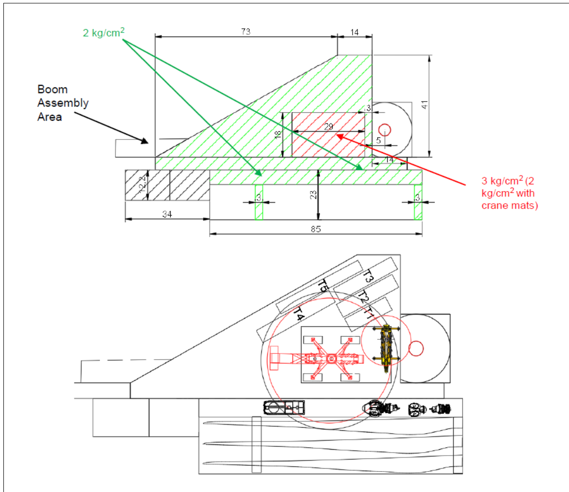
Figure 6-9: configurazione piazzola tipo in fase di cantiere (in rosso la piazzola definitiva)
