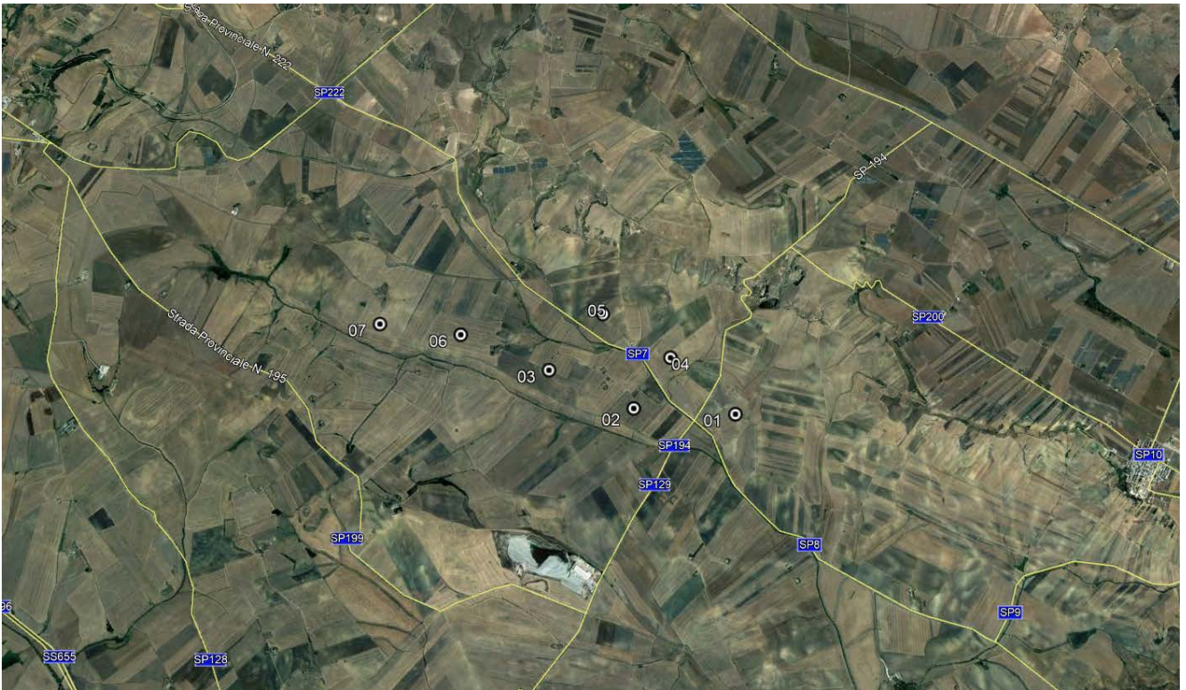
Fig. 2-1: localizzazione degli aerogeneratori rispetto alle strade circostanti
