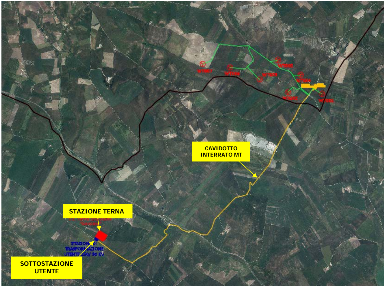
Fig. 2-5: Inquadramento dell'impianto su ortofoto
