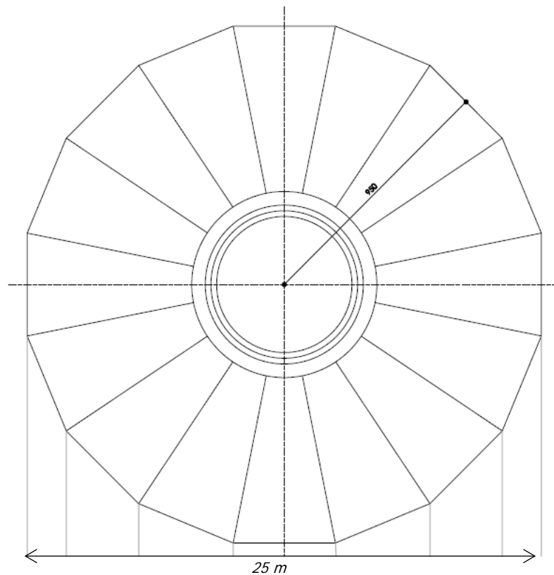
Fig. 6-1: pianta della fondazione tipo della torre eolica
