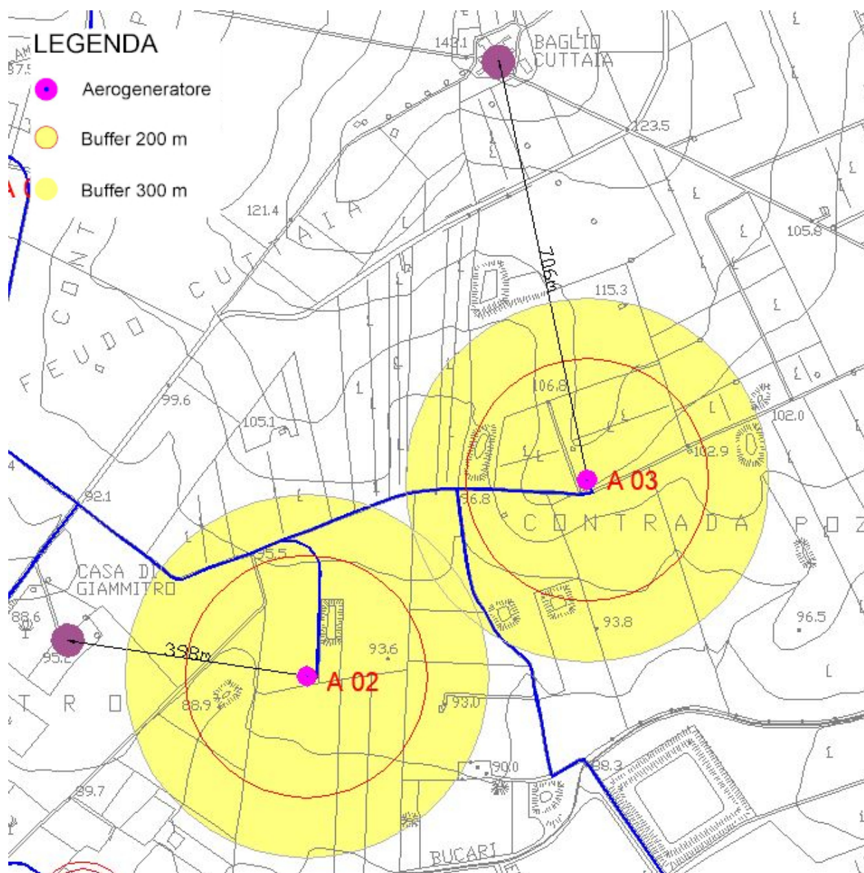
Figura 5: Distanza dei fabbricati dalle Torri 02 e 03
