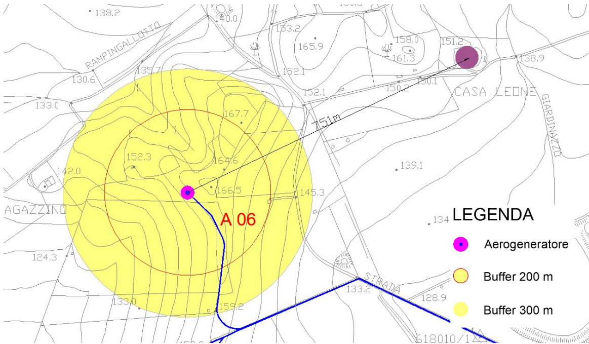
Figura 6: Distanza dei fabbricati dalla Torre 06
