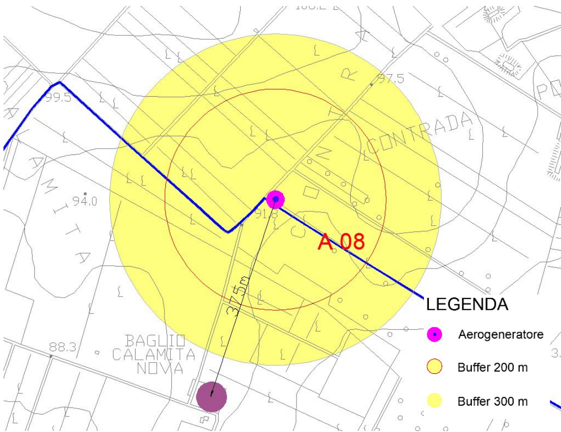
Figura 7: Distanza dei fabbricati dalla Torre 08
