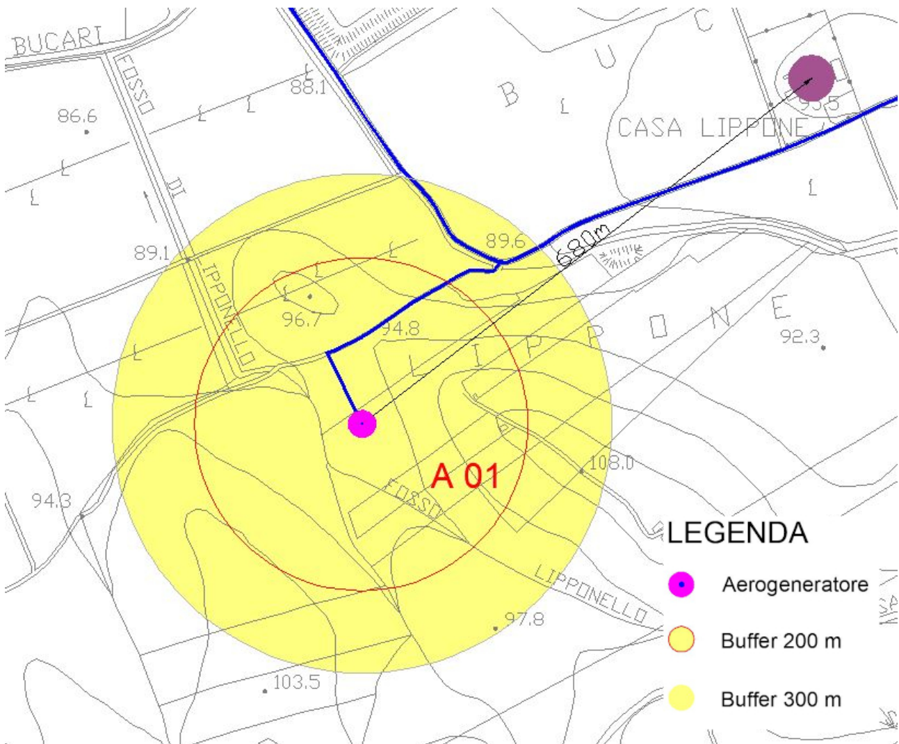
Figura 4: Distanza dei fabbricati dalla Torre 01
