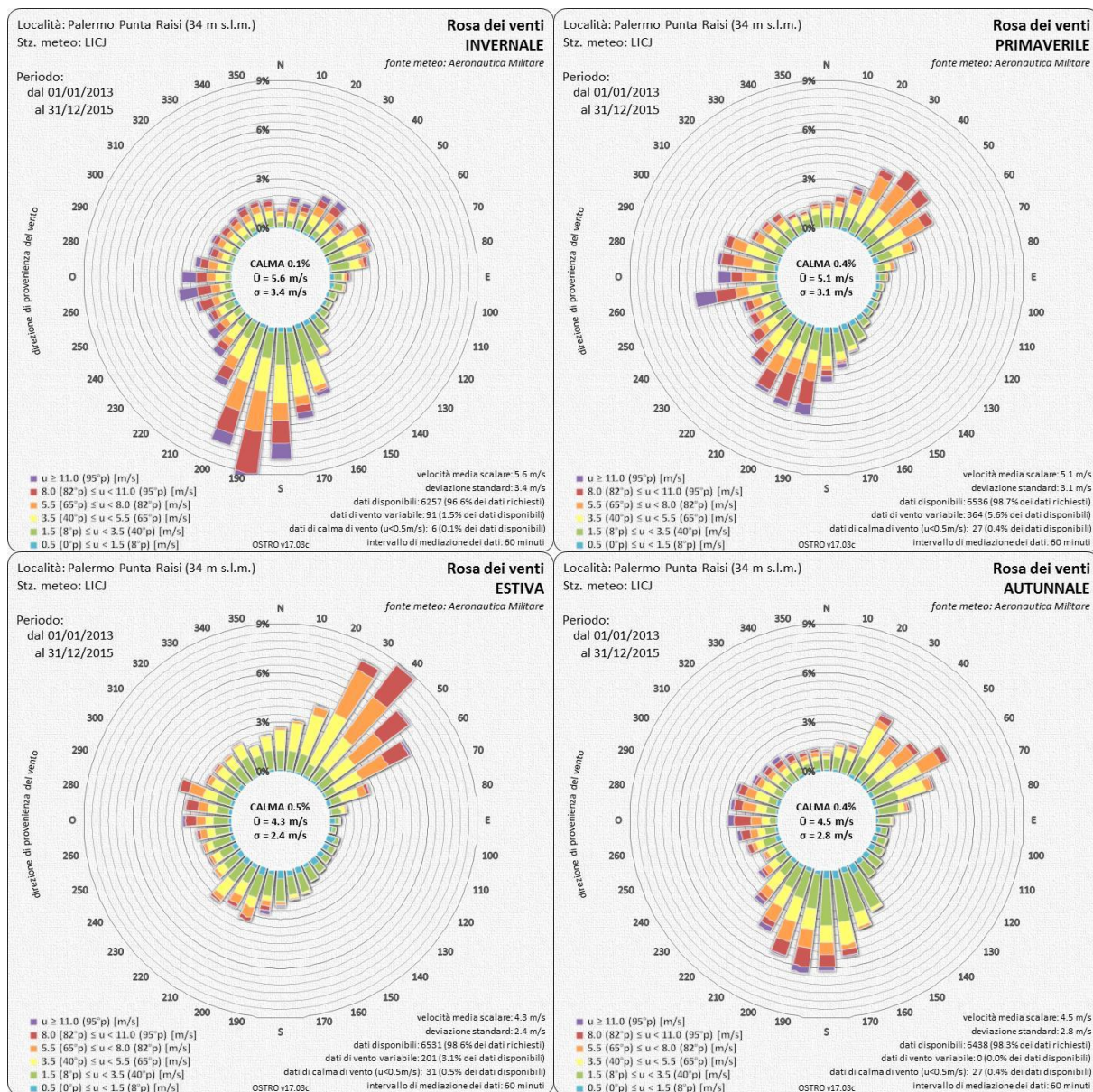
Figura 4.4.10 – Dati stazione meteo Palermo Punta Raisi. Rose dei venti stagionali. Dati misurati nel periodo 2013-2015.
