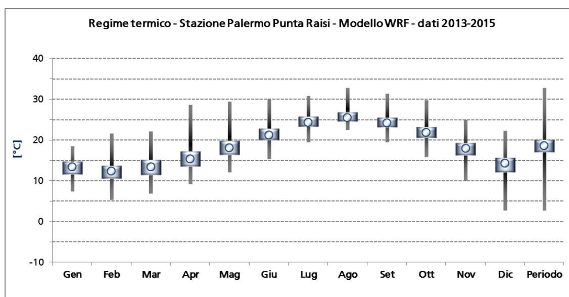
Figura 4.4.13 – Andamento termico stimato nella stazione di Palermo Punta Raisi (WRF). Periodo 2013-2015.
