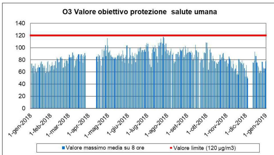
Figura 3.2.7 –Medie massime giornaliere su 8 ore dell’ozono a Termini Imerese
