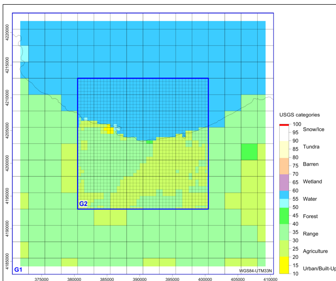
Figura 4.4.3 – Classe prevalente di uso del suolo alla risoluzione del modello meteorologico CALMET (elaborazione da fonte: USGS Global)
