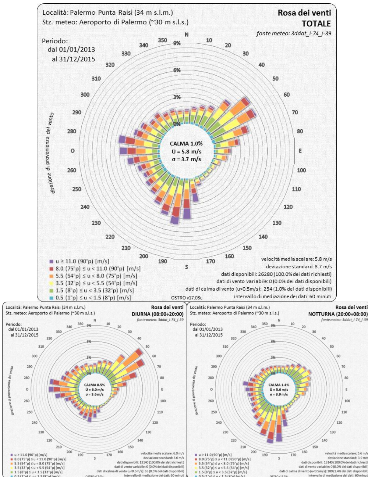
Figura 4.4.9 – Dati estratti dal modello WRF in corrispondenza della stazione meteo di Palermo Punta Raisi. Rose dei venti totale, diurna e notturna. Dati stimati nel periodo 2013-2015.
