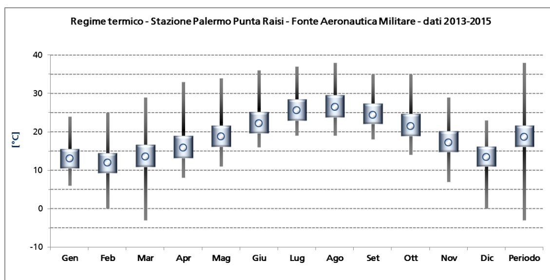
Figura 4.4.12 – Andamento termico stazione di Palermo Punta Raisi (fonte Aeronautica Militare). Periodo 2013-2015.
