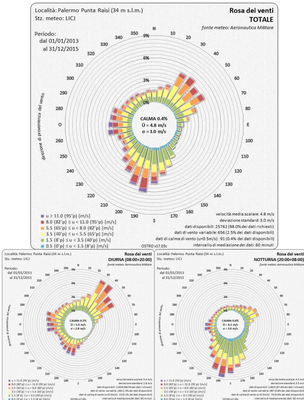
Figura 4.4.8 – Dati stazione meteo Palermo Punta Raisi. Rose dei venti totale, diurna e notturna. Dati misurati nel periodo 2013-2015.
