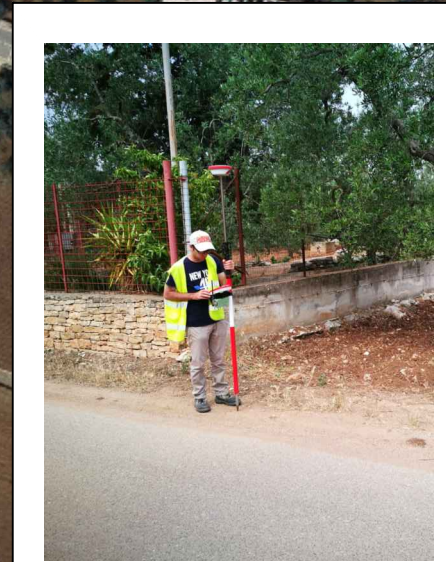
Foto 82 - Asse condotta (3152)
