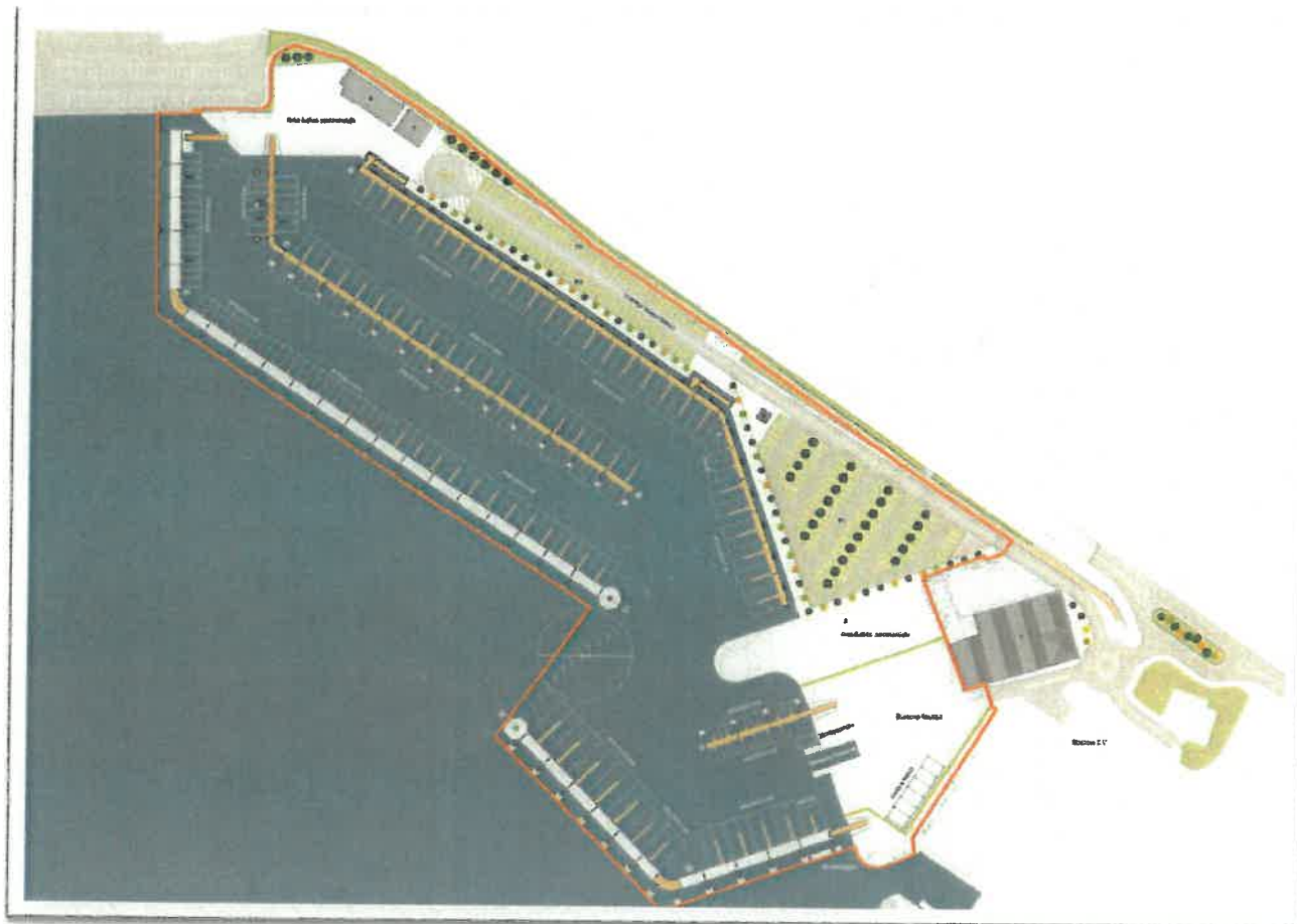
Figura 2 - Planimetria generale degli interventi
