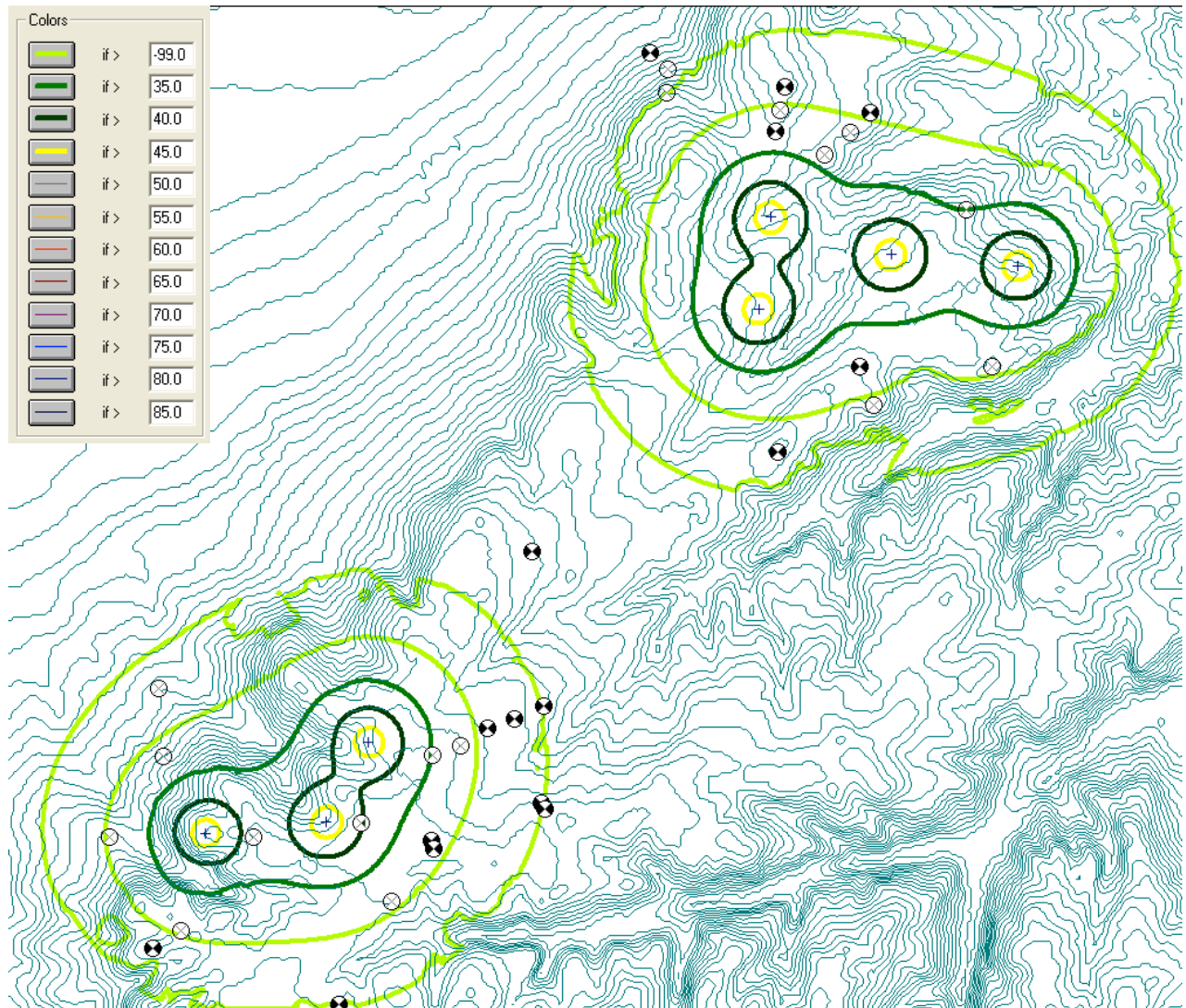
Figura 6 – Mappa isorumore durante l'esercizio nell'area interessata dalla centrale eolica (croci blu: turbine, dischi b/w: ricettori sensibili).
