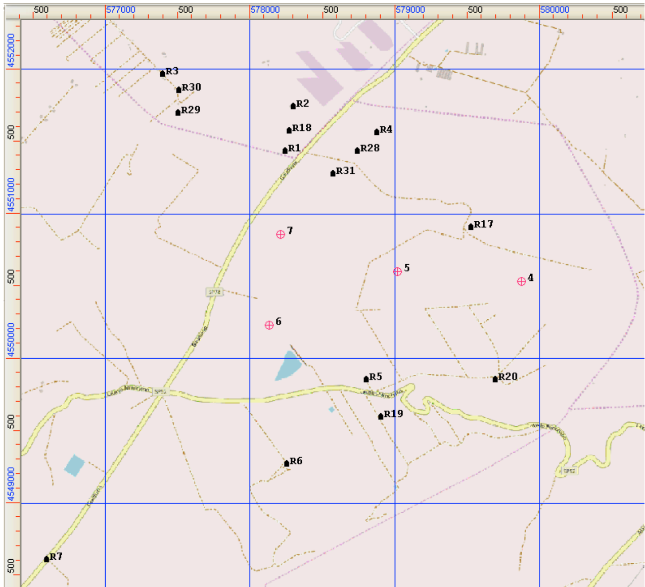
Figura 3 – Dettaglio layout impianto zona nord e ricettori presenti nell'area
