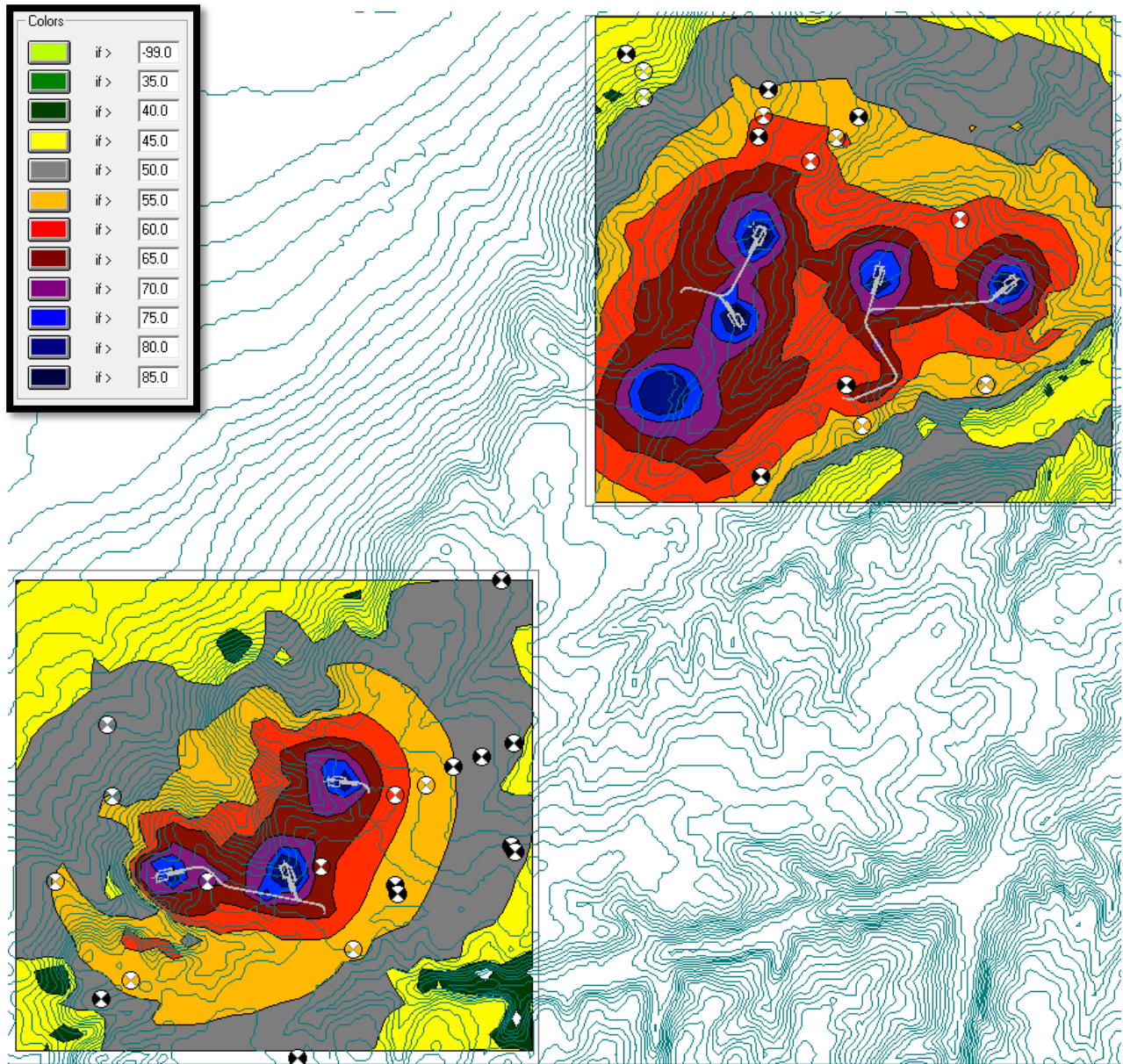
Figura 10 – Mappa isoruma esterno durante le operazioni di cantiere dell’area interessata dalla centrale eolica (croci blu: turbine, aree tratteggiate: cantieri, dischi b/w: ricettori sensibili).
