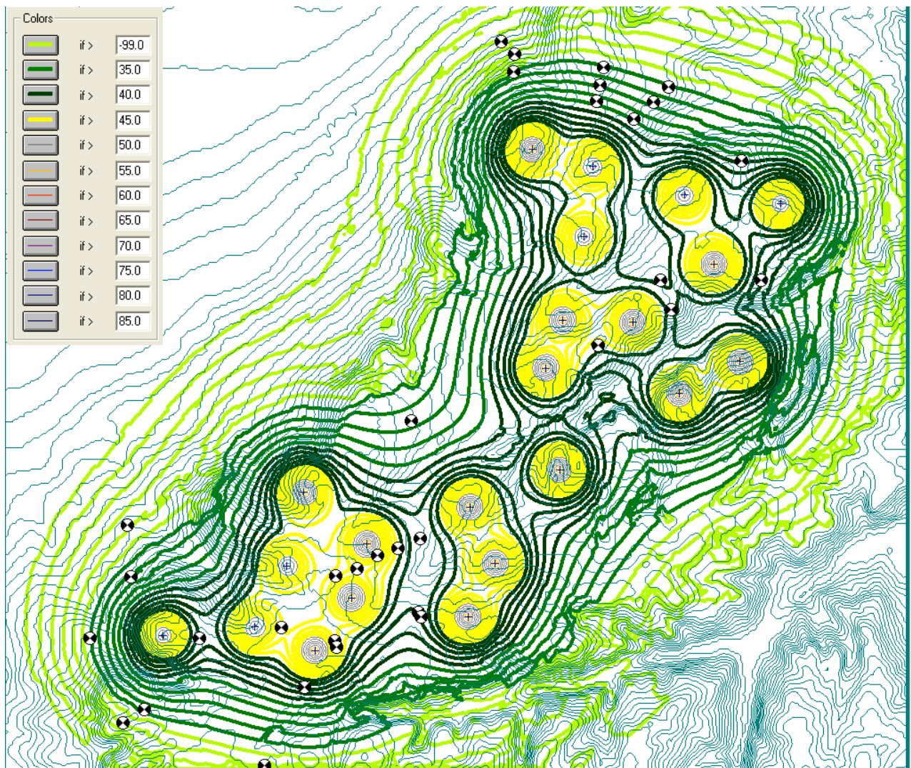
Figura 7 – Mappa isorumore durante l’esercizio nell’area interessata dalla centrale eolica proposta assieme alla centrale eolica esistente (croci blu: turbine, dischi b/w: tutti i ricettori).
