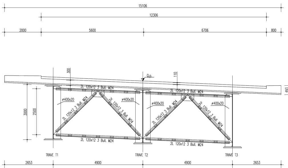
Figura 2 – Sezione trasversale tipica
