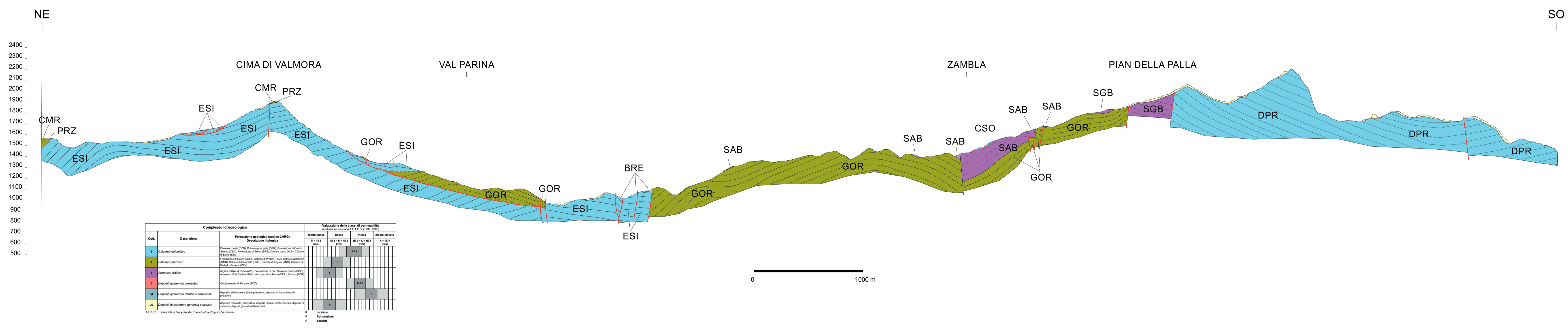
SEZIONE D-D
