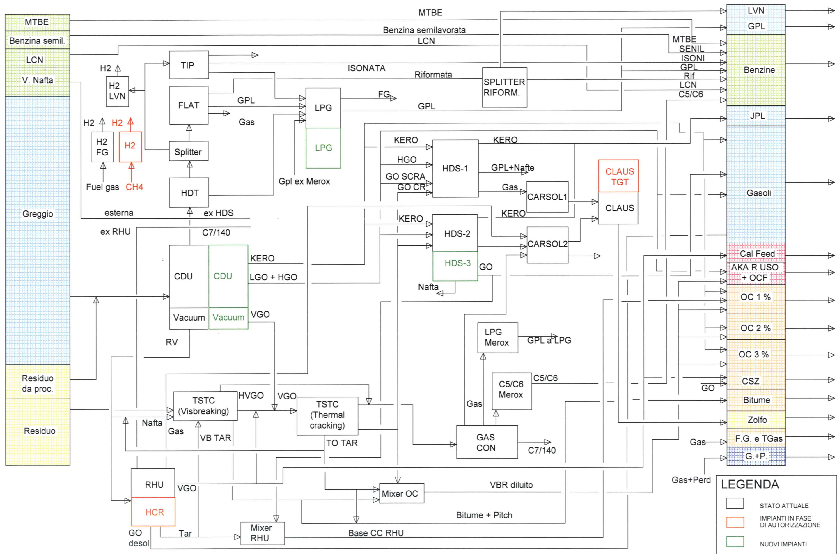
Figura 4.2.1b Schema a Blocchi della Raffineria
