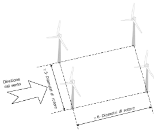
Figura 62: distanze minime tra aerogeneratori rispetto alla direzione prevalente del vento - fonte PIEAR
