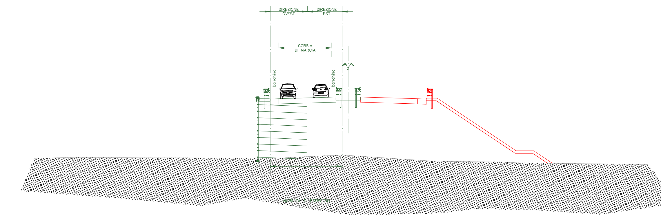
SEZIONE B-B' - FASE 3
