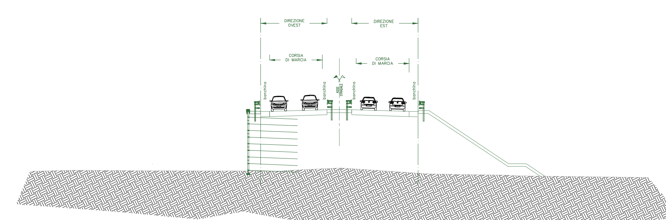
SEZIONE B-B' - FASE 4
