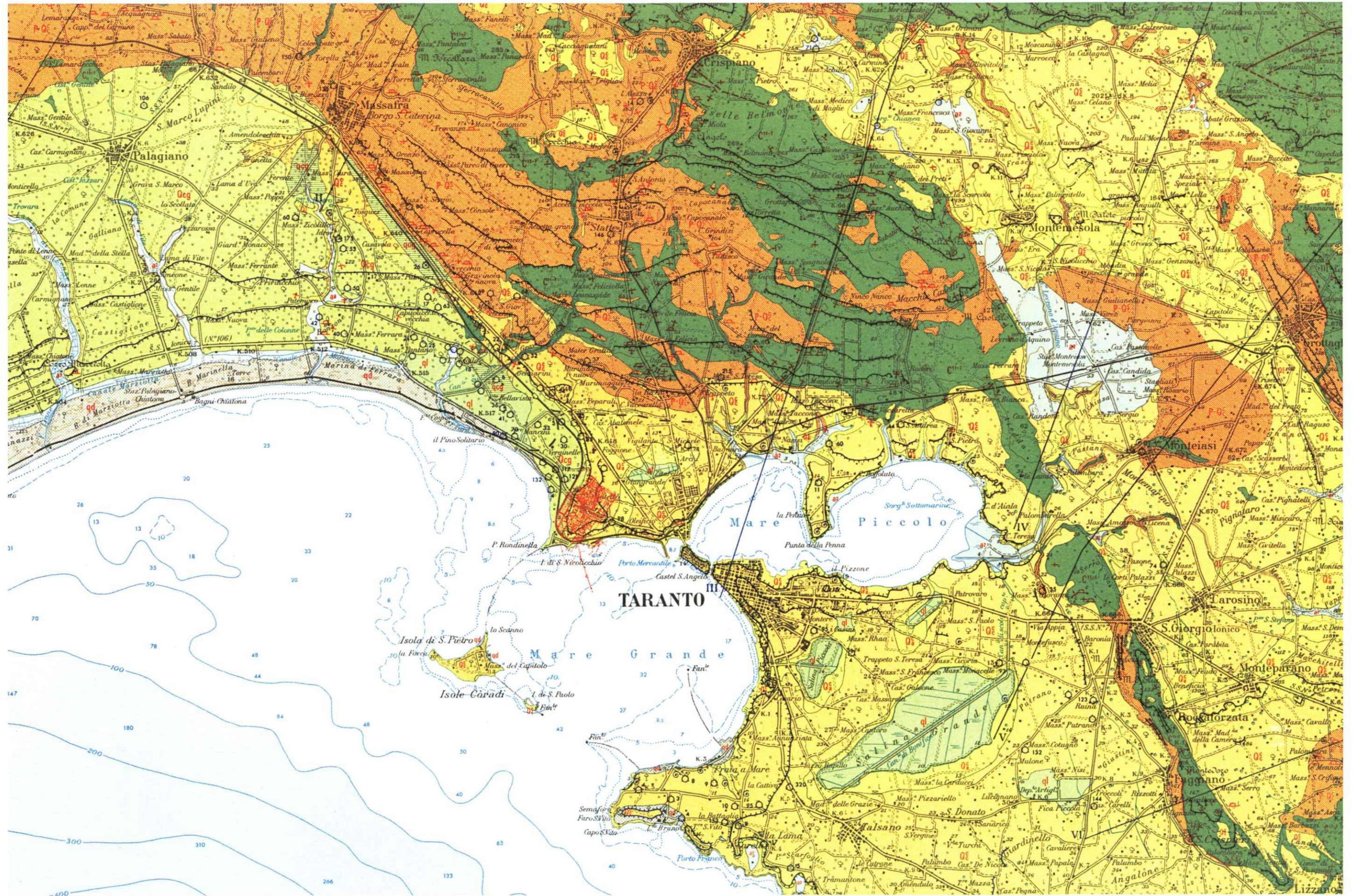
Figura 5.2.3.1a Carta Geologica (Scala 1:100.000) (2 di 2)
