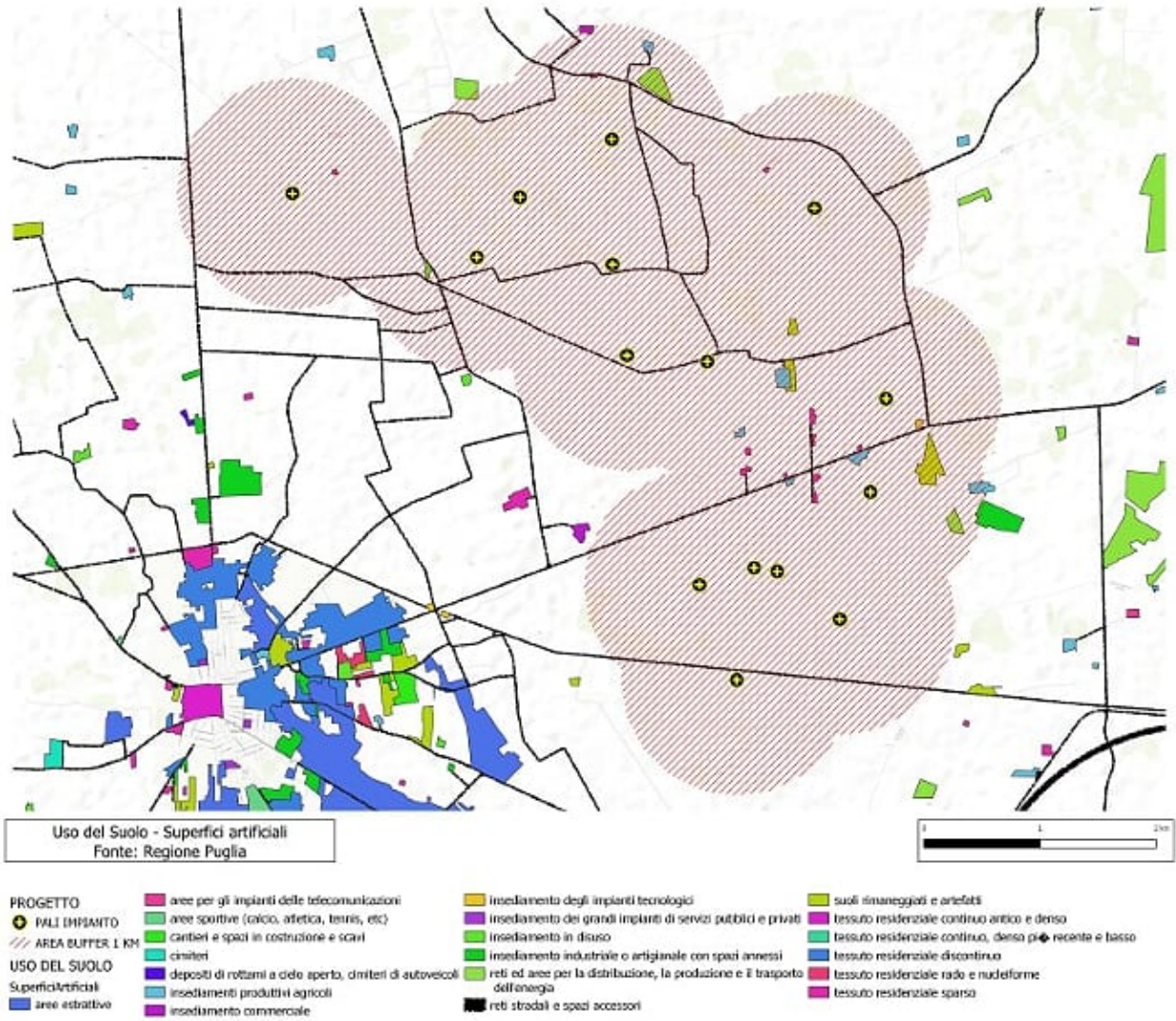
FIGURA 9 CARTA DI USO DEL SUOLO, SUPERFICI ARTIFICIALI
