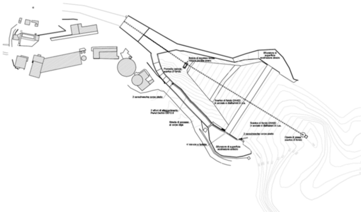
Figura 3 – Stato attuale della Diga Drove di Cepparello
