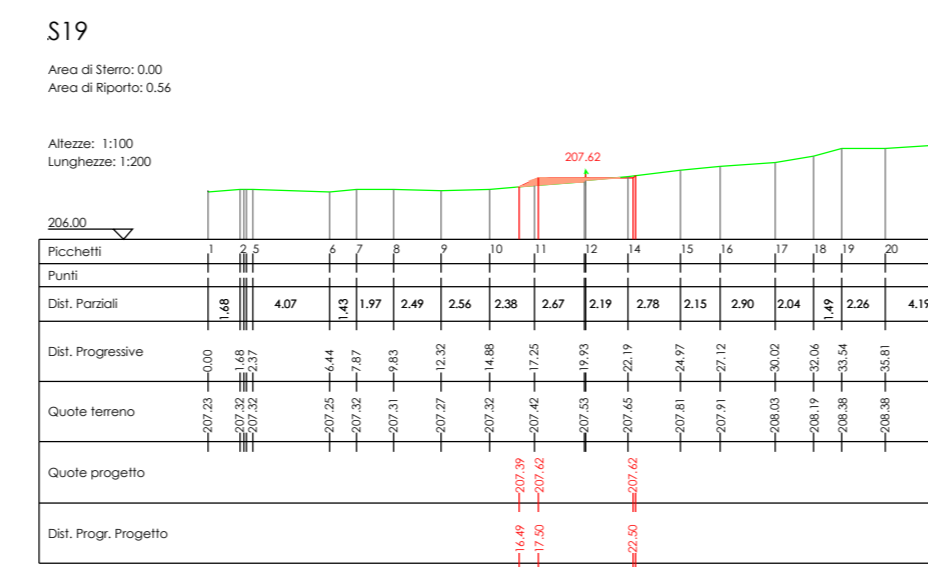
Sezioni su piazza Provvisoria
