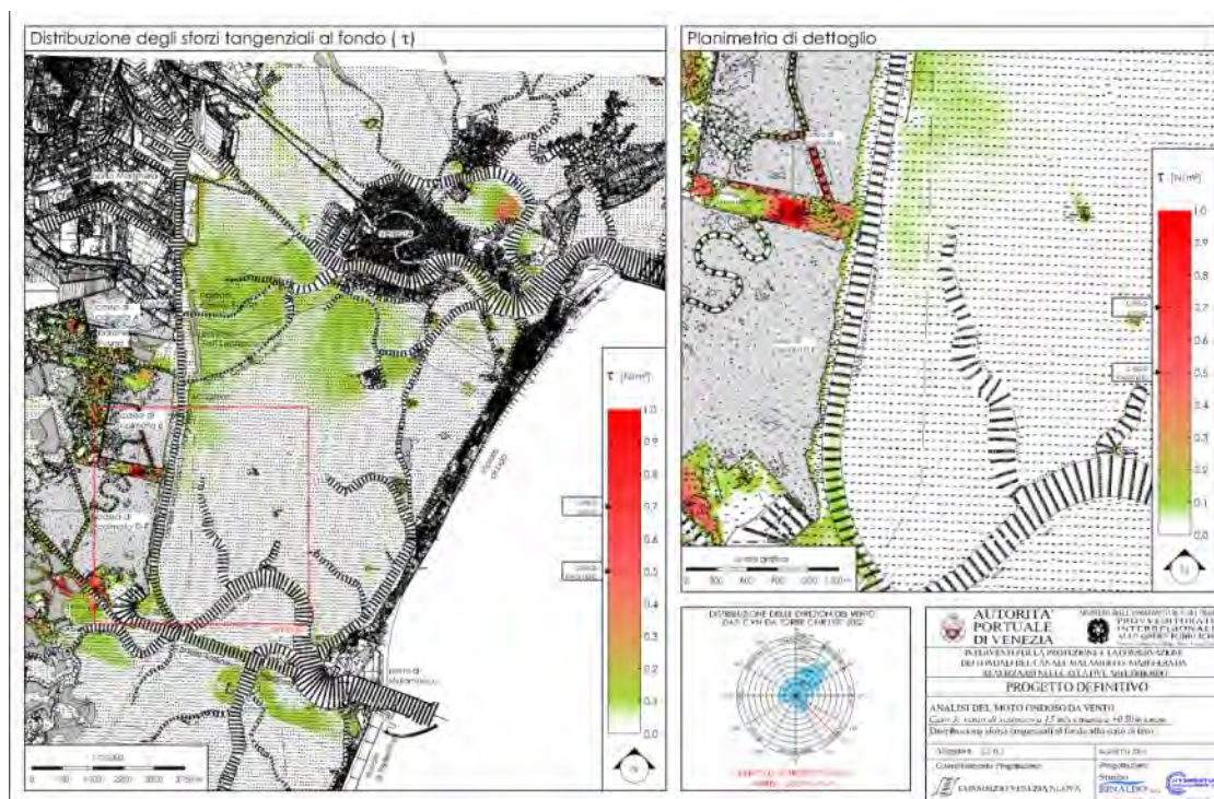
Figura 101: sforzi tangenziali al fondo caso 3
