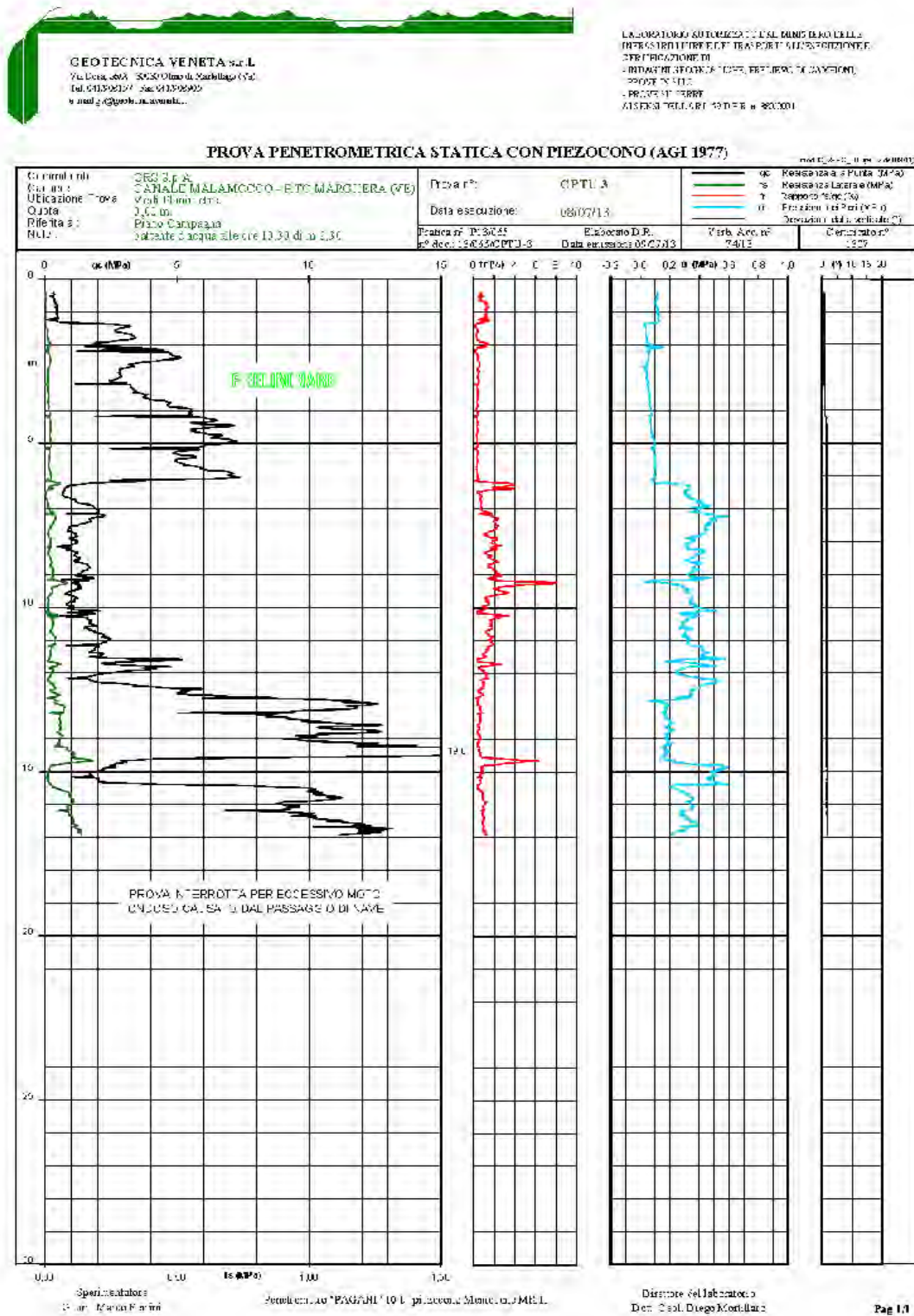
Figura 79: CPTU 3
