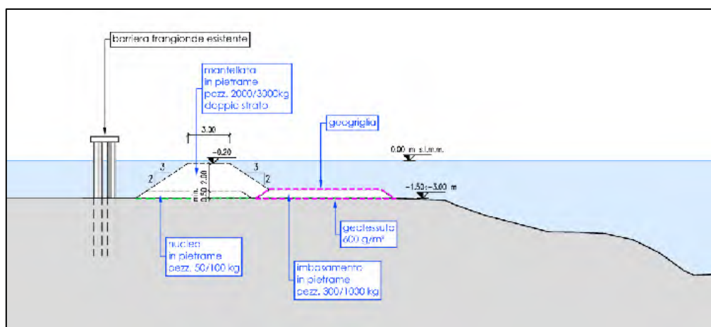
Figura 29: sezione tipo bordo Canale
