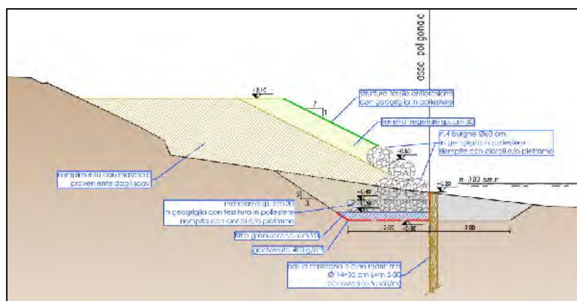
Figura 28: sezione tipo fronte foce Fossetta dei Barambani
