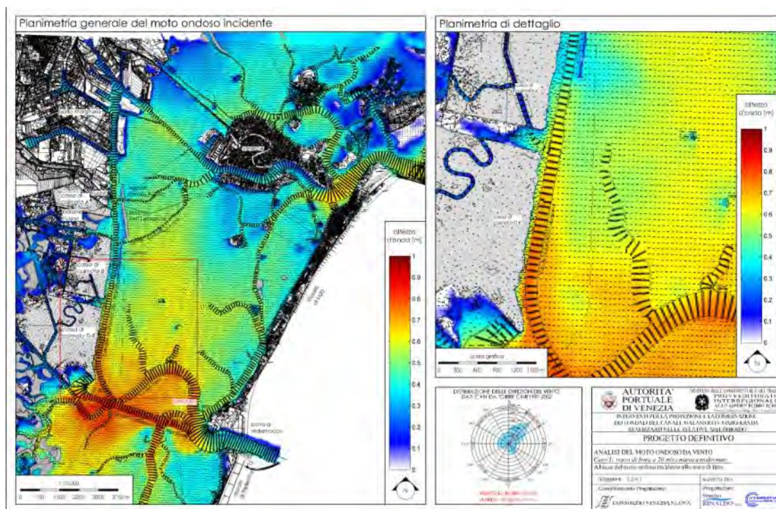
Figura 99: altezza d'onda caso 1
