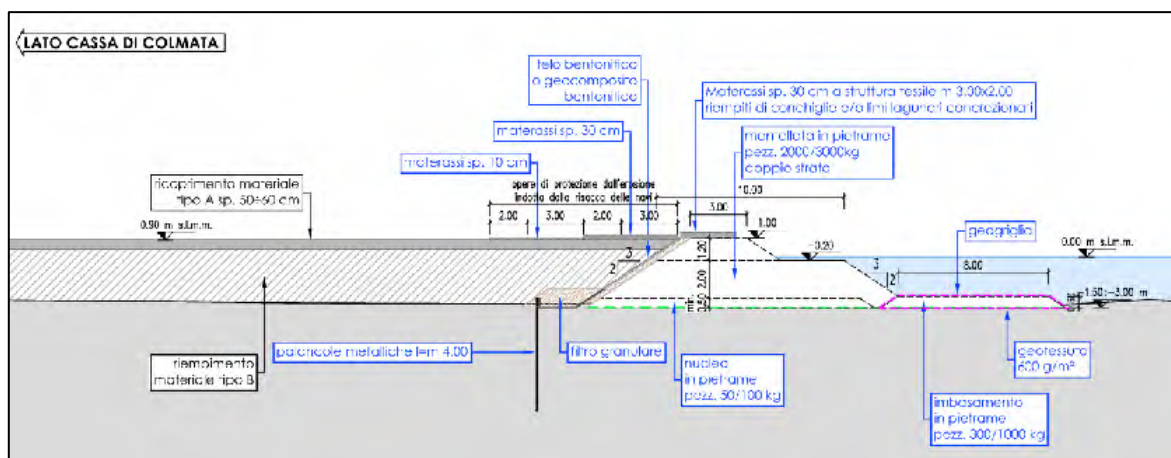
Figura 30: sezione tipo fronte Cassa di Colmata A
