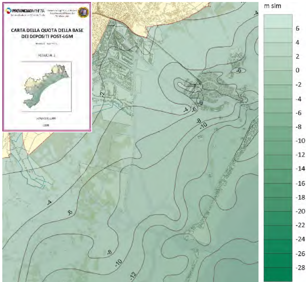
Figura 75: carta della quota della base dei depositi post-LGM
