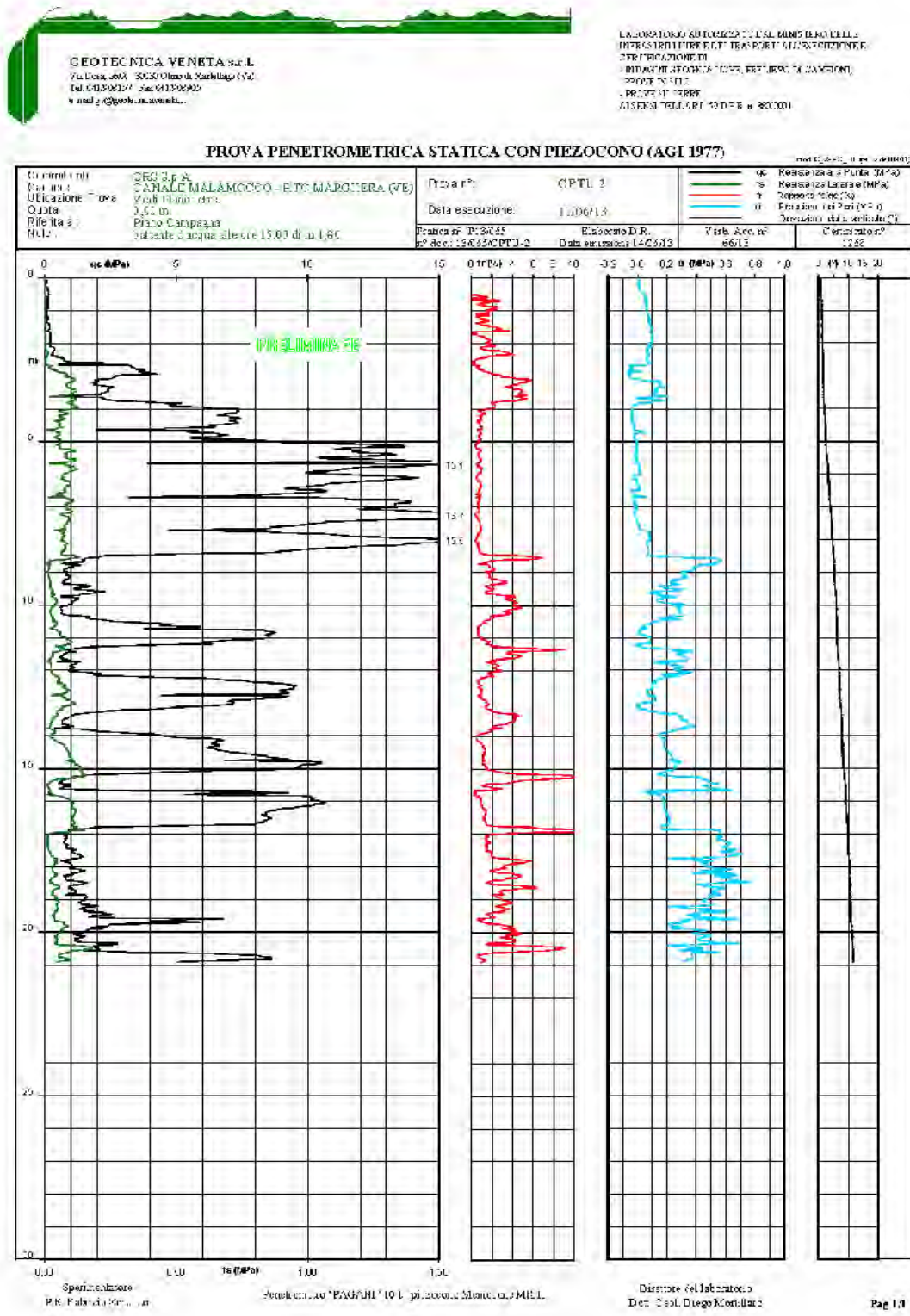
Figura 78: CPTU 2
