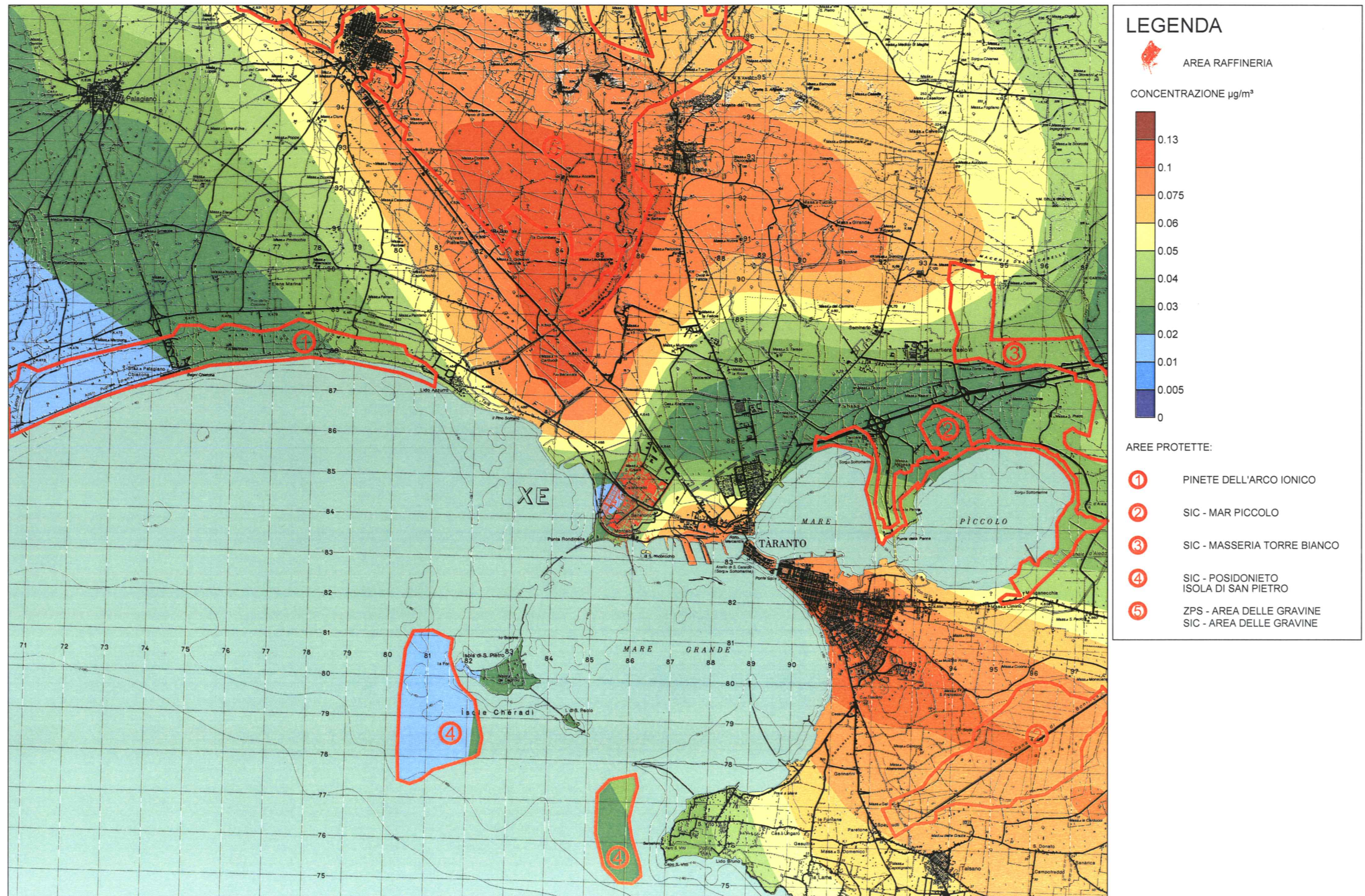
Figura 5.3.1.2d Concentrazioni Medie Annue di PTS nello Scenario Attuale (Scala 1:90.000)
